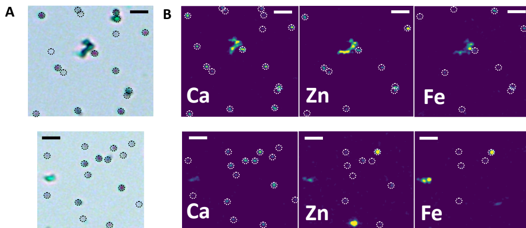
Figure 7-2. Composition chimique des ommochromosomes purifiés à partir des yeux de mouches domestiques.
