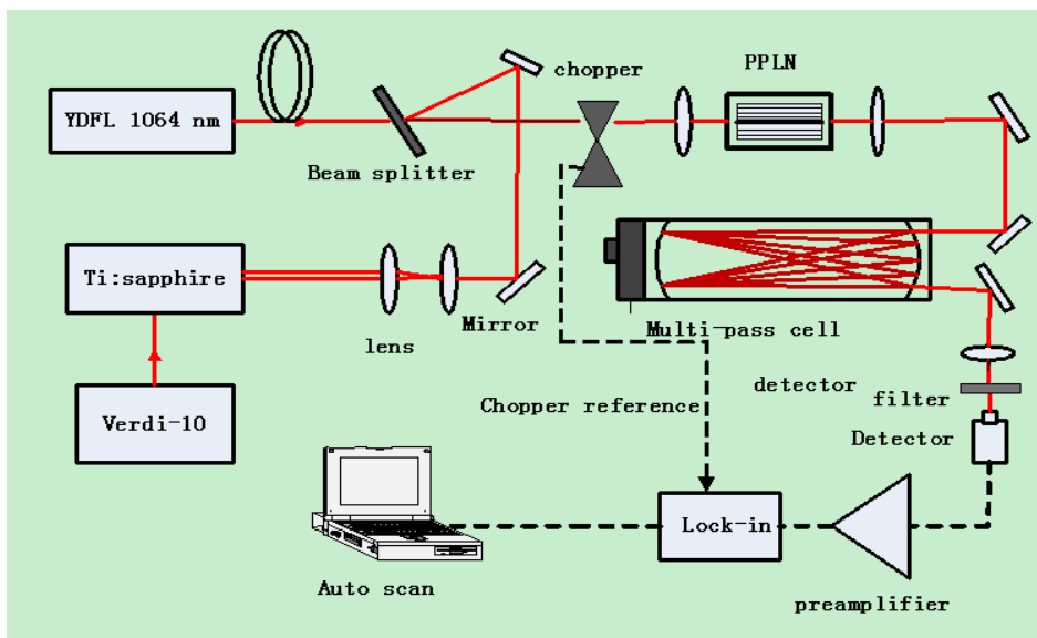
图 5.18 3590 cm -1 差频输出光系统示意图
