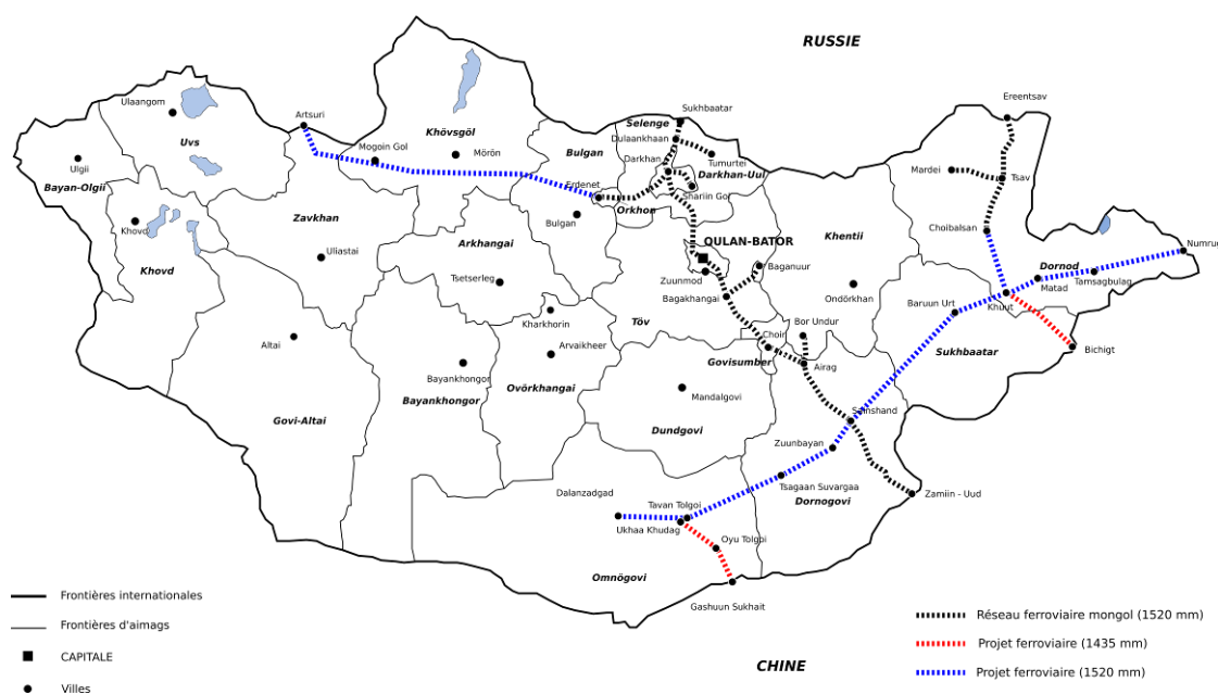
Carte du projet ferroviaire tel que proposé par la résolution parlementaire du 24 octobre 2014 1 .
