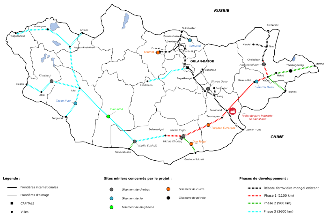
Le projet ferroviaire mongol de juillet 2010 3 .
