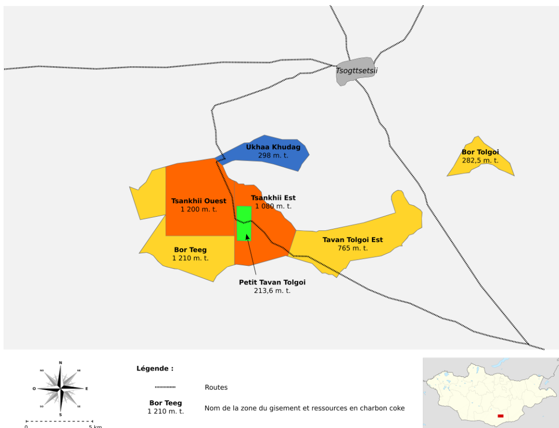
Structure du gisement de Tavan Tolgoi et ses ressources en charbon métallurgique 1 .
