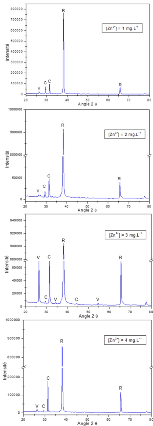
Figure 8 : Diagramme DRX des précipités solides déposés sur la surface pré-entartée en présence du chlorure de zinc
