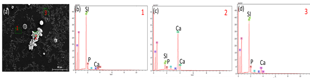
Figure IV-18 : (a) Photo MEB de la surface d'acier inoxydable recouverte par un film sol-gel après un test de QCM. Analyse EDX du film déposé sur acier inoxydable après application de la technique de QCM pour (b) la zone 1, (c) la zone 2 et (d) la zone 3.
