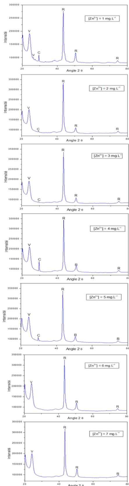
Figure 9 : Diagramme DRX des précipités solides déposés sur la surface pré-entartée en présence du nitrate de zinc
