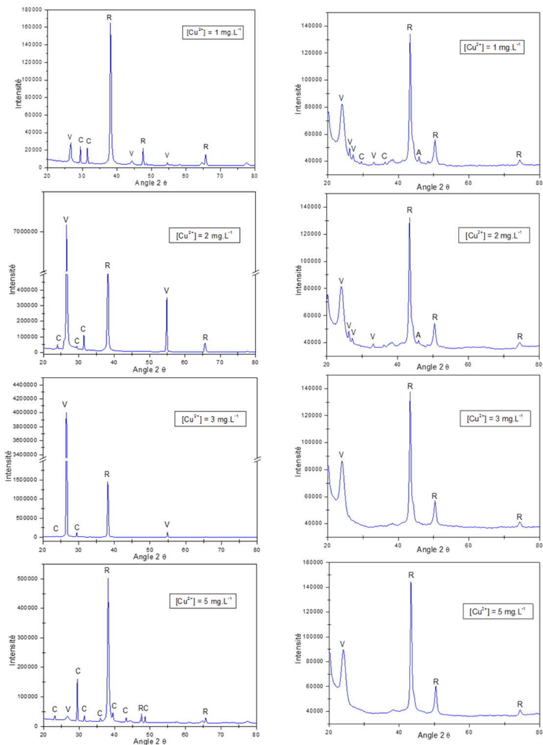
Figure 6 : Diagramme DRX des précipités solides déposés sur la surface pré-entartée en présence du chlorure de cuivre
