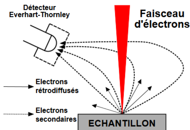
Figure II-11 : Fonctionnement général du MEB [34].
