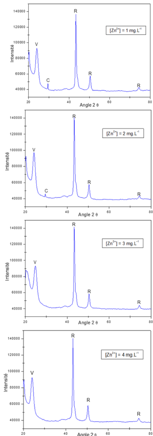
Figure 8 : Diagramme DRX des précipités solides déposés sur la surface pré-entartée en présence du chlorure de zinc
