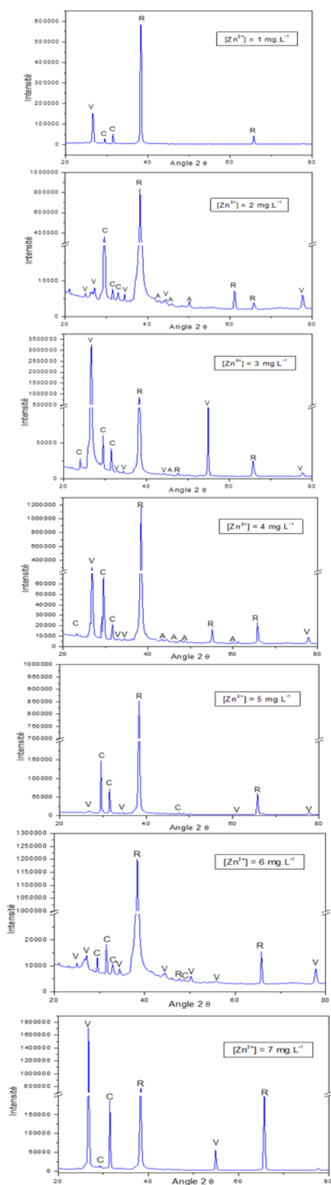
Figure 9 : Diagramme DRX des précipités solides déposés sur la surface pré-entartée en présence du nitrate de zinc
