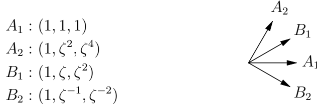
Figure 2.1 – Représentation des quatre bases optimales pour CHSH-3
