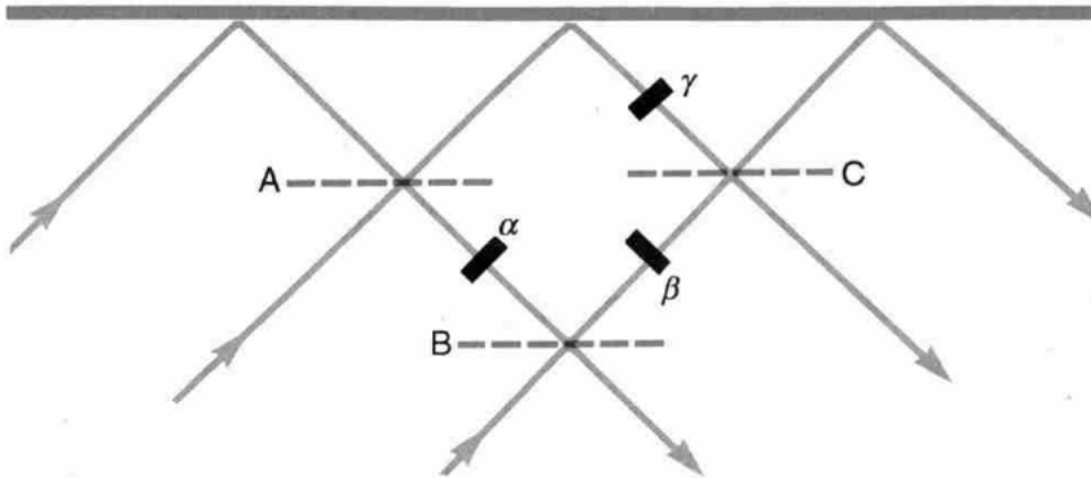
Figure 1.1 – Schéma de tritter pour d = 3
