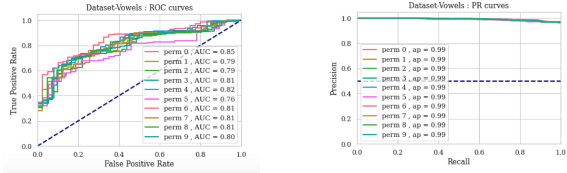
(a) Courbes ROC et valeurs AUC
