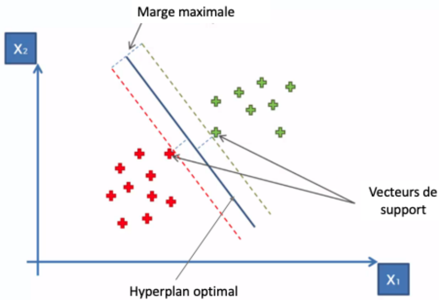
FIGURE 3.1: illustration d'un classificateur SVM
