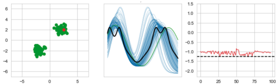
FIGURE 5.4: Cas d’un échantillon de test normal : La figure à gauche présente l’ensemble d’entraînement en vert et l’échantillon normal à prédire en rouge. La figure du milieu montre les courbes des densités des k-distances des données d’entraînement en bleu. La courbe noire représente la densité moyenne des courbes bleues et la courbe verte représente la densité de la k-distance de l’échantillon rouge. La figure à droite montre le rapport des densités d’atteignabilité locales pour l’échantillon de test (courbe rouge) et le paramètre offset en ligne discontinue noire.
