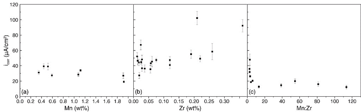
Figure 1-14 : Valeurs de densité de courant de corrosion ( i_{\text{corr}} ) en fonction de la teneur en élément d'alliage : (a) alliage binaire Mg-Mn, (b) alliage binaire Mg-Zr et (c) alliage ternaire Mg-Mn-Zr [94].
