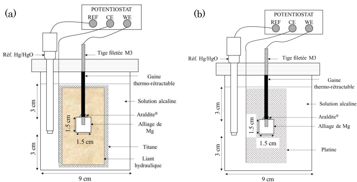
Figure 2-11 : Systèmes utilisés pour l'acquisition des courbes de polarisation : (a) électrodes enrobées dans le géopolymère et (b) électrodes simples.
