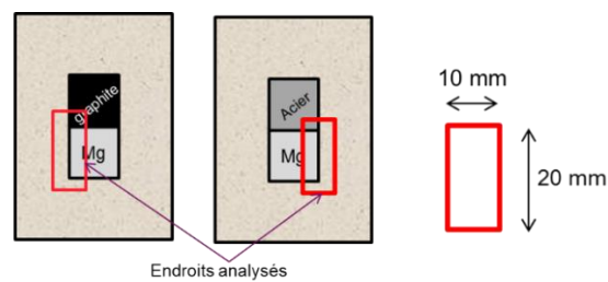
Figure 2-16 : Schéma des dimensions choisies pour les analyses FIB-STEM.
