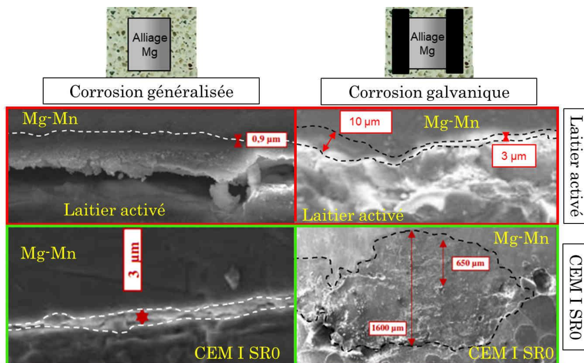
Figure 1-33 : Caractérisation MEB de l'interface Mg-Mn/Laitier activé et Mg-Mn/CEM I SR0 après un an de corrosion généralisée et galvanique (adapté de Rifai [8]).
