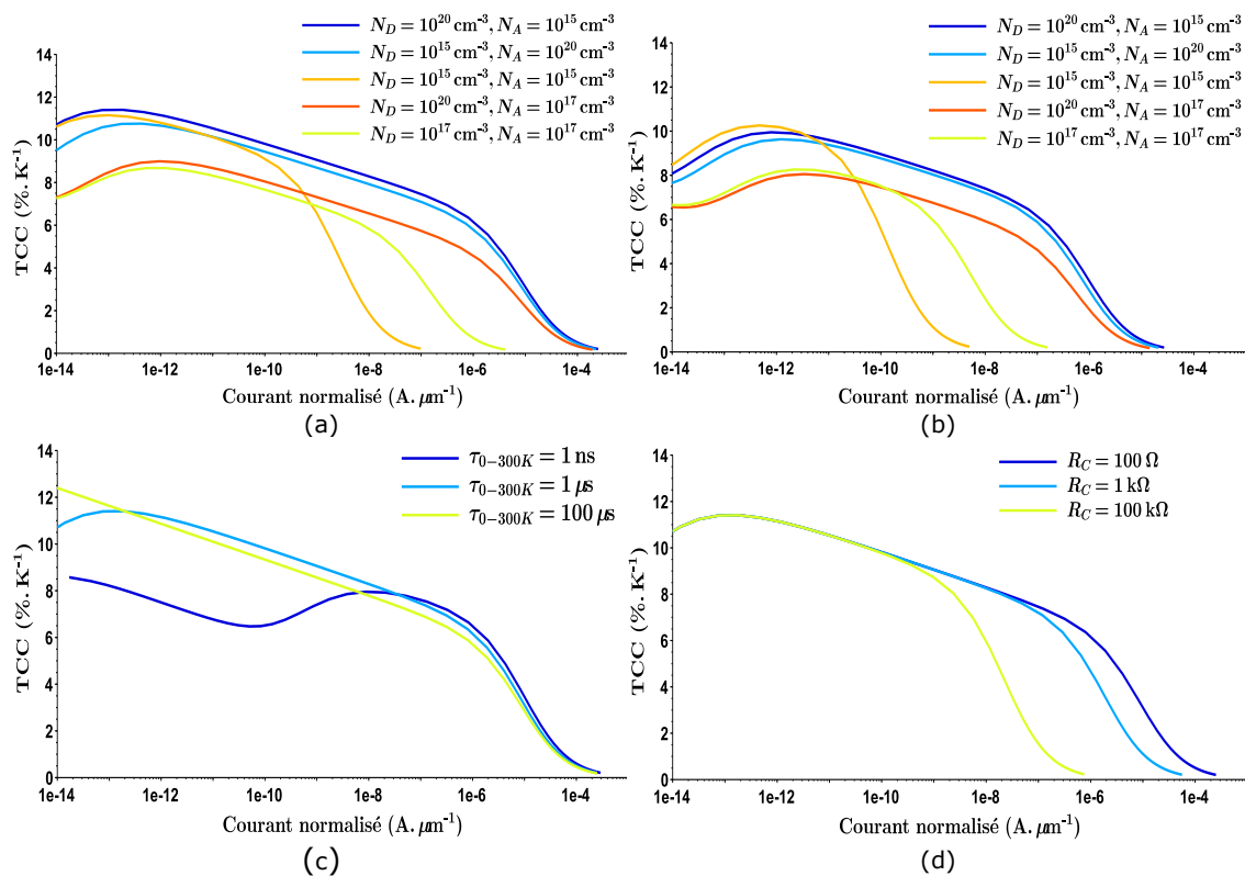
FIGURE 2.5 – TCC d’une jonction PN à T = 300 K en fonction du courant normalisé pour différentes configurations. (a) TCC en fonction du dopage pour une jonction courte W_n = W_p = 5 \mu m . (b) TCC en fonction du dopage pour une jonction longue W_n = W_p = 100 \mu m . (c) TCC en fonction de \tau_{0-300K} pour une jonction courte p-n + avec N_A = 10^{15} cm^{-3} et N_D = 10^{20} cm^{-3} . (d) TCC en fonction de R_C pour une jonction courte p-n + avec N_A = 10^{15} cm^{-3} et N_D = 10^{20} cm^{-3} .
