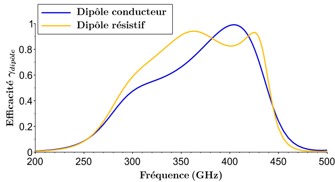
FIGURE 5.11 – Comparaison de l'absorption entre un dipôle conducteur avec charge discrète adaptée R = 40 \Omega et dipôle résistif R_{\square} = 2.67 \Omega \cdot \square^{-1} , pour H_{\text{cap}} = 50 \mu\text{m} , W_{\text{dip}} = 20 \mu\text{m} , L_{\text{dip}} = 300 \mu\text{m} et H_{\text{couplage}} = 10 \mu\text{m} .
