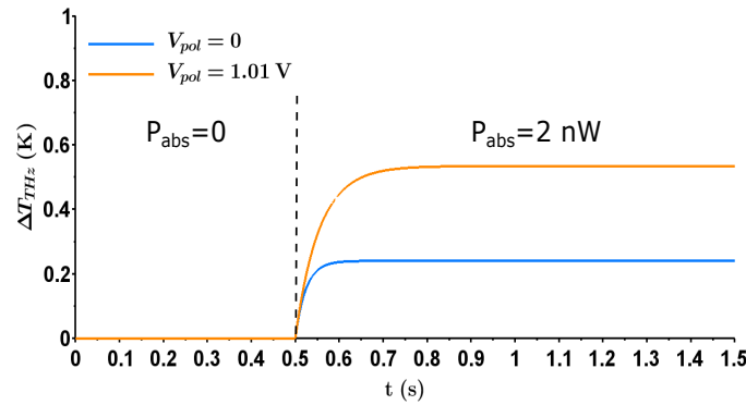
FIGURE 5.30 – Comparaison de la réponse indicielle \Delta T_{THz}(t) du bolomètre, pour une puissance optique absorbée P_{abs} = 2 \text{ nW} à partir de t = 0.5 \text{ s} , entre une polarisation nulle de la diode (courbe bleue) et une polarisation en tension continue (courbe orange).
