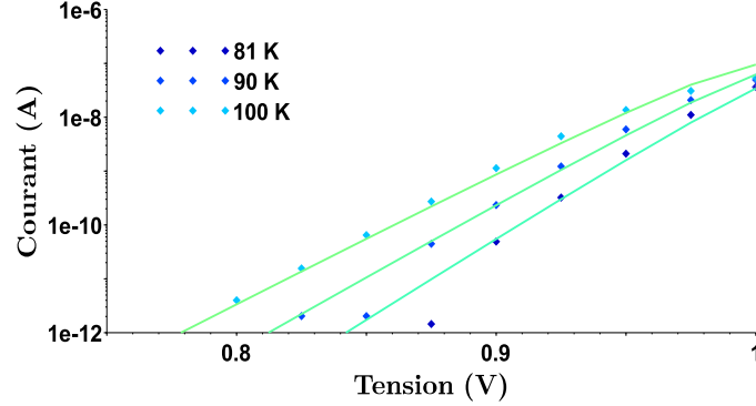
FIGURE 4.15 – Modélisation du courant inverse I_R de la jonction latérale caisson L_i = 20 \mu\text{m} entre 81 K et 100 K. Les symboles représentent les mesures. Les lignes continues sont le courant de recombinaison I_r calculé avec le modèle 4.10.
