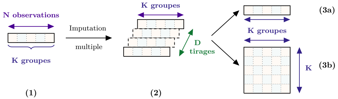
Figure 3: Méthodologie d'imputation multiple. (1) Jeu de données initial contenant des valeurs manquantes, avec N observations réparties dans K groupes. (2) L'imputation multiple renvoie D estimateurs pour le vecteur de paramètres d'intérêt. (3a) Les D estimateurs sont combinés grâce à la première règle de Rubin pour obtenir l'estimateur combiné. (3b) L'estimateur de la matrice de variance-covariance de l'estimateur combiné est donné par la deuxième règle de Rubin.
