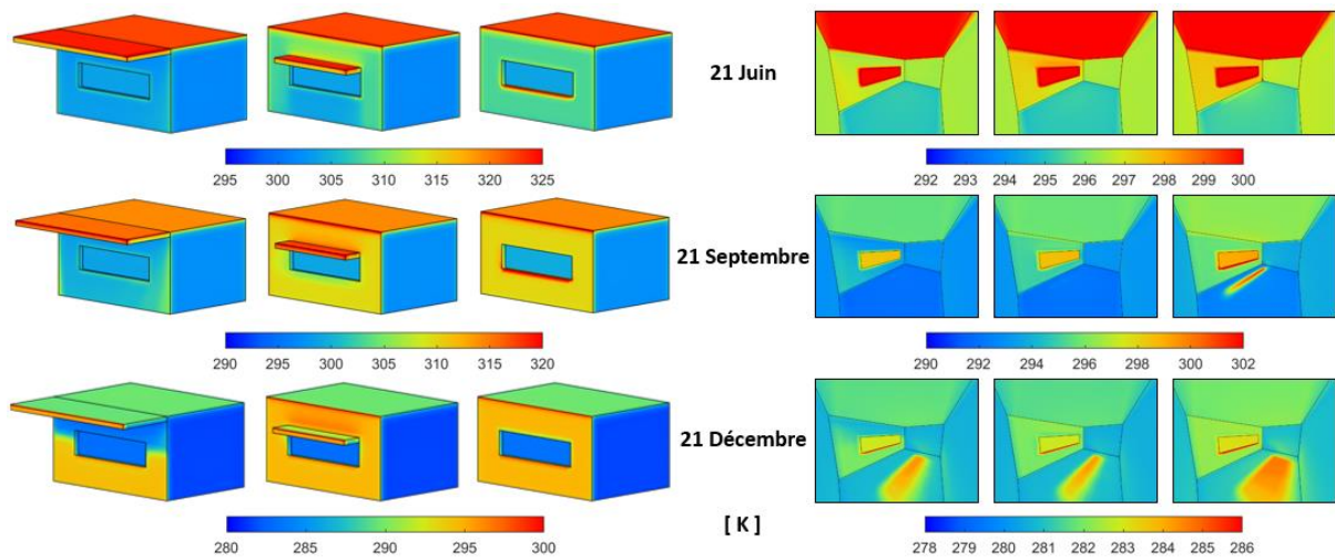
Figure 2.25 Températures de surface au midi solaire pour les trois jours étudiés.
