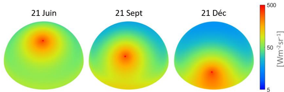
Figure 2.23 Distribution des radiances du ciel au midi solaire pour les trois jours étudiés à Cordoue.
