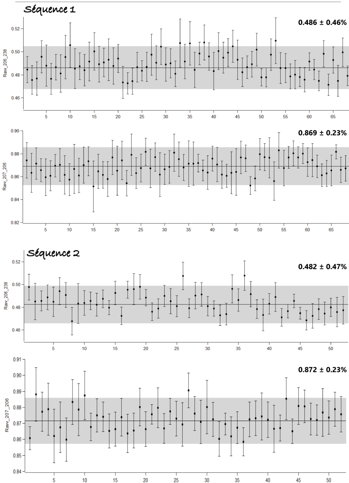
Figure III-5 - Séquences « test » montrant la fluctuation des rapports mesurés sur une durée de ~ 10h, réalisées en Novembre 2019. L'axe des ordonnées correspond aux rapports ^{207}Pb/^{206}Pb ou ^{206}Pb/^{238}U mesurés sur le NIST614 et l'axe des abscisses correspond aux différentes analyses reportées au cours du temps.
