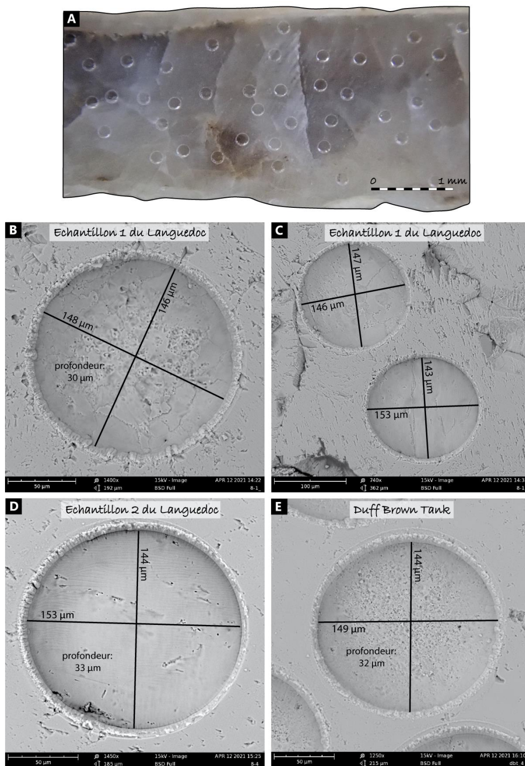
Figure III-7 - Illustration des cratères d'ablation A. Observation d'un échantillon de calcite de faille du Languedoc (échantillon GD-1, cf. CHAPITRE V.1.4.) en lumière réfléchie après analyse au LA-ICP-MS. B. C. et D. Images MEB de cratères d'ablation sur des échantillons de calcite de faille du Languedoc. E. Image MEB d'un cratère d'ablation sur le matériel de référence secondaire Duff Brown Tank. Les paramètres d'ablation correspondent à une fréquence de 8 Hz, une fluence de 4 \text{ J.cm}^{-2} et un diamètre du faisceau LASER de 150 \text{ }\mu\text{m} .
