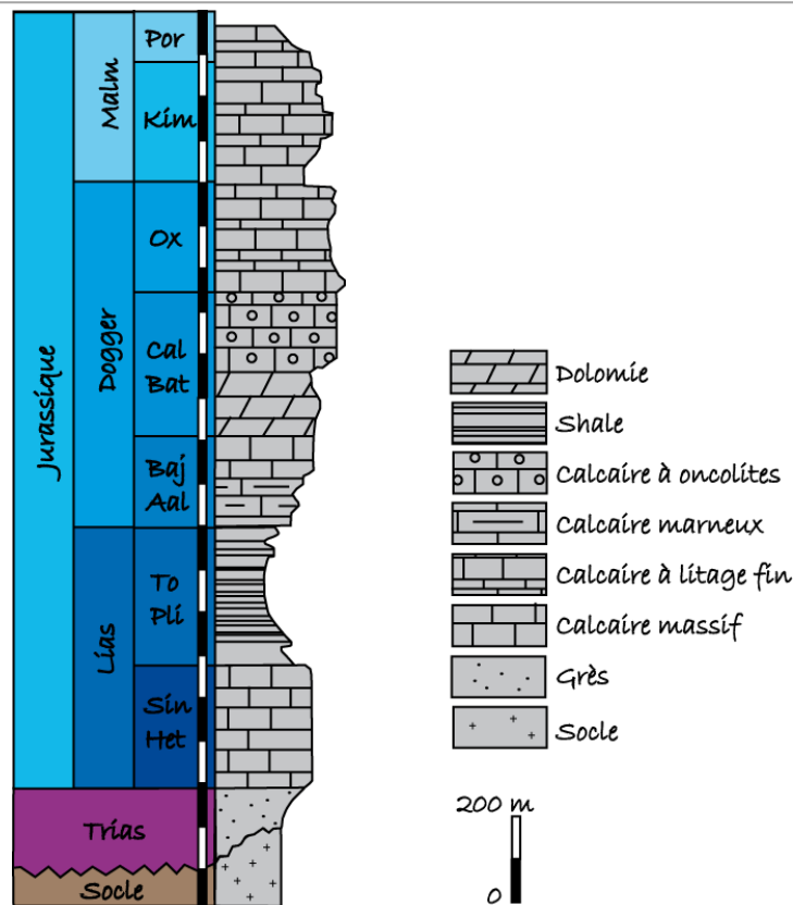
Figure II-10 - Colonne stratigraphique du bassin des Grands Causses d'après Dubois (1985). Het : Hettangien ; Sin : Sinémurien ; Pli : Pliensbachien ; To : Toarciens ; Aal : Aalénien ; Baj : Bajocien ; Bat : Bathonien ; Cal : Callovien ; Ox : Oxfordien ; Kim : Kimméridgien ; Por : Portlandien
