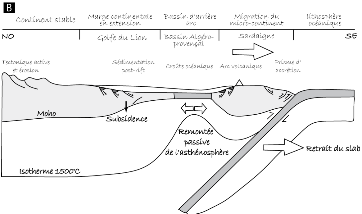
Figure II-19 - Le rifting priabo-aquitainien A. Schéma structural de la marge du Golfe du Lion : mise en évidence des structures extensives liées au rifting. La localisation des structures provient de Séranne et al. (2021). B. Le golfe du Lion perçu comme un bassin d'arrière-arc issu du retrait du slab vers le SE (modifié d'après Séranne et al. (1999)).
