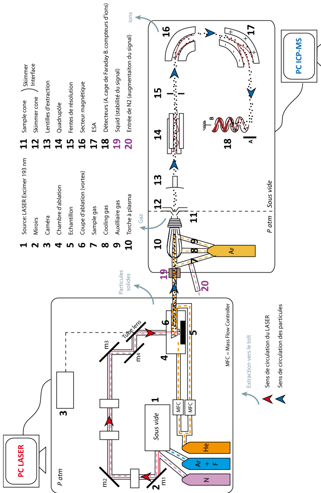
Figure I-11 – Représentation schématique du LA-ICP-MS au laboratoire GEOPS (Orsay)
