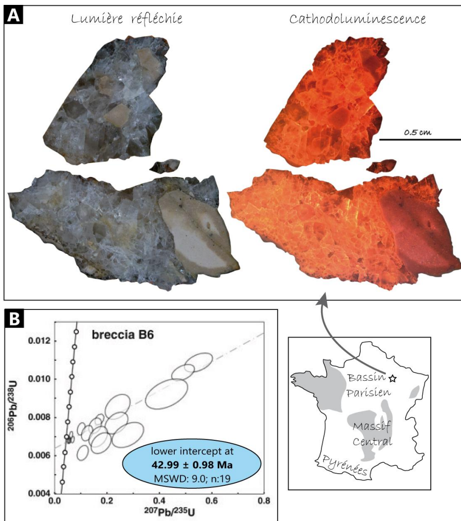
Figure III-4 - Le matériel de référence secondaire interne B6. A. Observations à la lumière réfléchie et au microscope à cathodoluminescence de la brèche B6 du laboratoire GEOPS. B. Diagramme Concordia et âge obtenu pour B6 par LA-ICP-MS, d'après Pagel et al. (2018).
