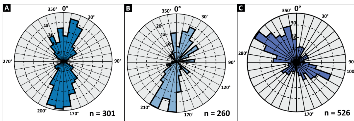
Figure VII-7 - Diagrammes en rosace illustrant l'orientation de la contrainte principale \sigma_1 associée aux plans de faille inverses et décrochants mesurés dans A. les Grands Causses, B. le Languedoc, C. les Corbières.
