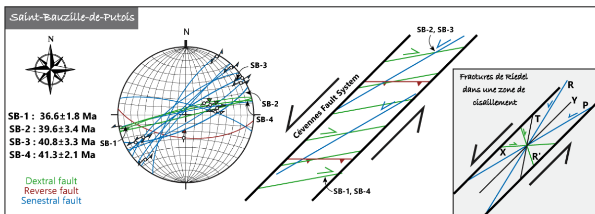
Figure V-13 - Représentation stéréographique des données microtectoniques (hémisphère inférieure, canevas de Schmidt) de la lentille Jurassique de Saint-Bauzille-de-Putois et représentation des données microtectoniques dans le contexte de la zone de Faille des Cévennes. Comparaison avec les fractures de Riedel dans une zone de cisaillement (R, P et Y fractures synthétiques ; R' et X fractures antithétiques ; T fracture par traction) d'après Logan et al. (1992).
