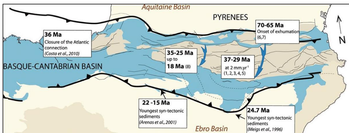
Figure II-22 - Compilation de données issues de la thermochronologie basse température montrant la propagation de l'exhumation du Nord au Sud dans les Pyrénées (Fillon, 2016). Les données proviennent de 1. Fitzgerald et al. (1999) 2. Gibson et al. (2007) 3. Sinclair (2005) 4. Metcalf et al. (2009) 5. Fillon et Van der Beek (2012) 6. Yelland (1991) 7. Morris et al. (1998) 8. Jolivet et al. (2007) ; et Meigs et al. (1996), Arenas et al. (2001), Costa et al. (2010).
