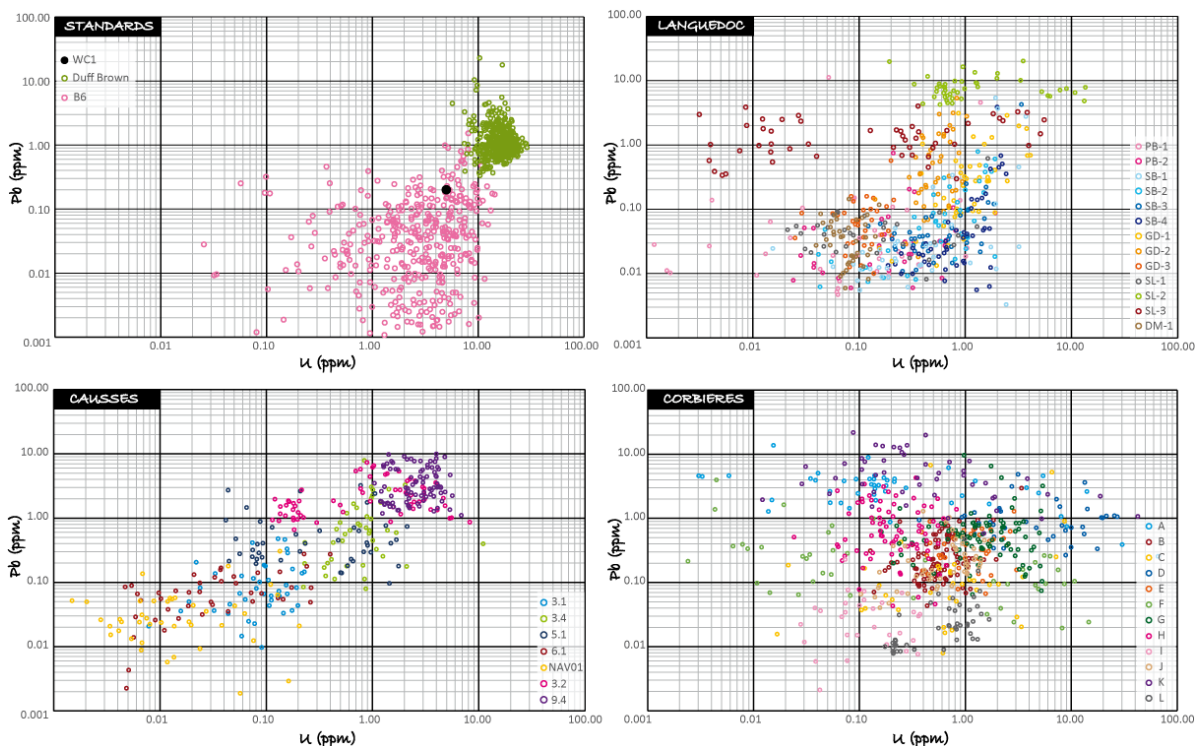
Figure VII-2 - Teneurs en U et Pb des calcites de faille ayant obtenu un âge U-Pb au cours de ce travail. Les teneurs ont été calibrées à partir du matériel de référence primaire WC-1 (5 ppm d'uranium et 0.2 ppm de plomb). Les incertitudes pour chacune des analyses, bien qu'existantes, n'ont pas été figurées sur les graphes par soucis de lisibilité. Le pourcentage d'incertitude sur la teneur en uranium de chacune des analyses est en moyenne de l'ordre de 5-10%, et sur la teneur en plomb de l'ordre de, en moyenne, 15-20%.
