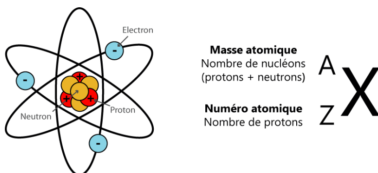
Figure I-8 - Rappel sur la composition et nomenclature d'un atome
