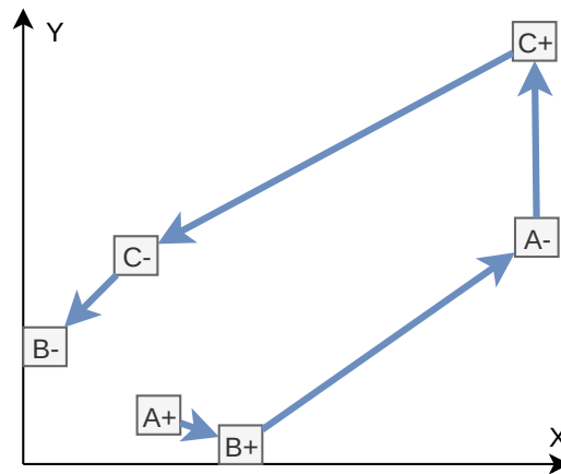
Figure 7.2 – A gauche, un tableau indiquant les coordonnées spatiales de l'origine et la destination de 3 requêtes. A droite, les coordonnées spatiales d'un taxi durant une course partagée de longueur minimale traitant ces requêtes. La course commence au stop A+ (origine de A) et finit à B- (destination de B).
