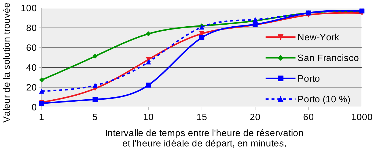
Figure 9.8 – Valeur des solutions trouvée par l'algorithme glouton en fonction de l'avance avec laquelle les clients réservent. (10%) signifie dans ce tableau "Avec 10% des requêtes ayant été formulées un jour en avance". Les clients acceptent toujours un retard égal à exactement 20% de la durée prévue de leur trajet, ce qui signifie généralement un peu plus de 2 minutes. Il n'y a pas de retard fixe toléré. Les taxis ont une batterie infinie.
