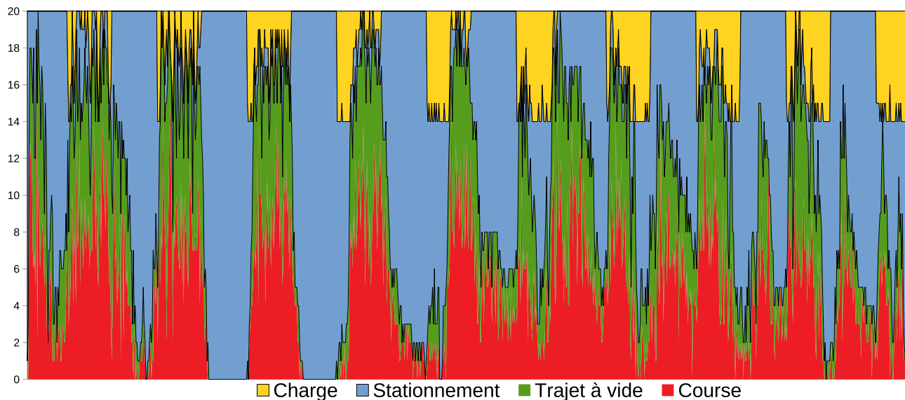
Figure 9.7 – Ici, les edtt sont générés par SLC.
