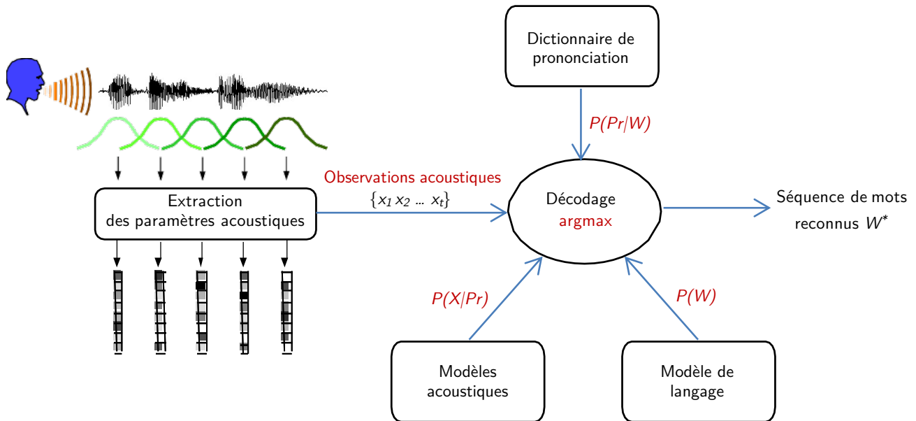
Schéma 1 - Architecture d'un système de reconnaissance de la parole adapté de Ghannay (Ghannay, 2017)
