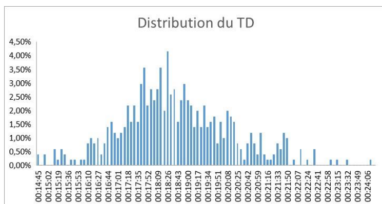
Figure 80 : Distribution du temps de parcours de Foch vers Porte de Vertou
