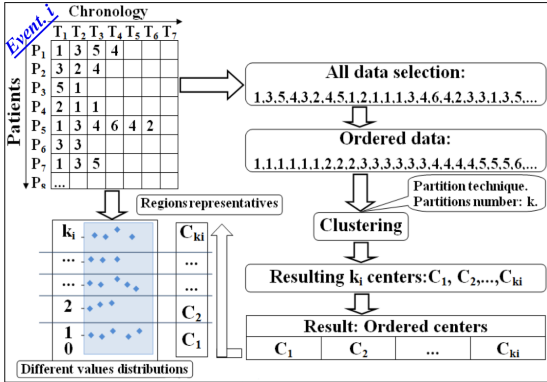
Figure 5.2. Processus de clustering d'un événement numérique E_i .
