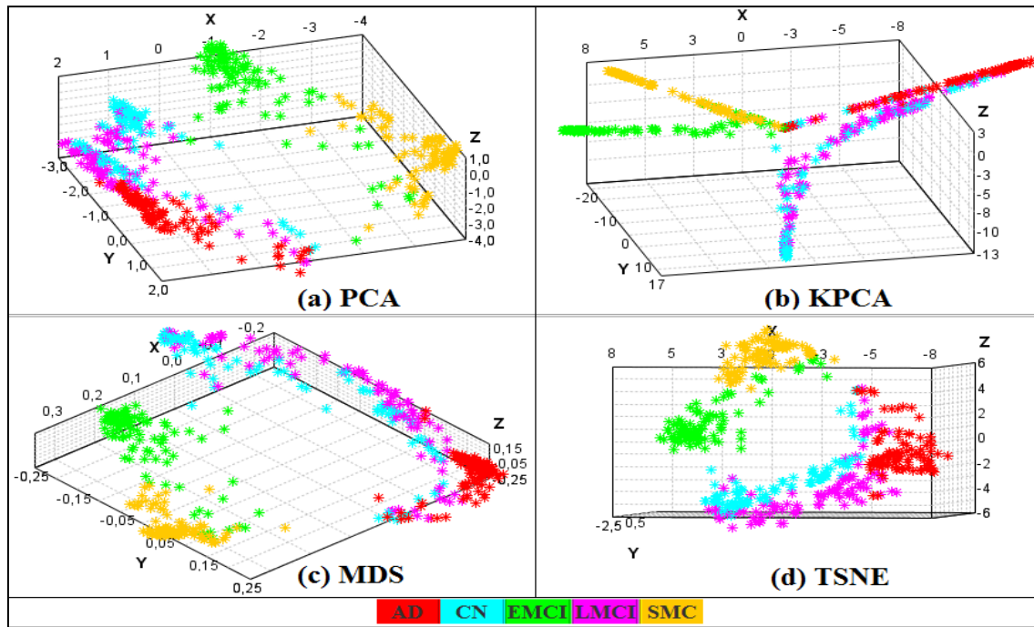
Figure 6.4. Visualisation de la réduction 3D. (a)PCA, (b)KPCA, (c)MDS, (d)TSNE.
