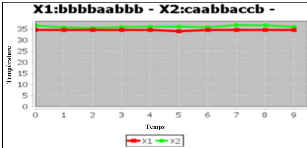
Figure 4.1. Représentation SAX de X1 et X2 sans normalisation.
