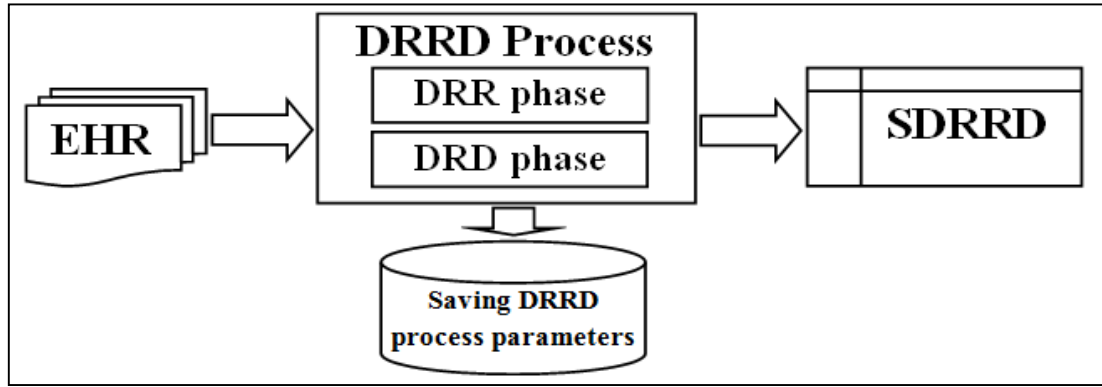
Figure 6.2. Processus de représentation de données.
