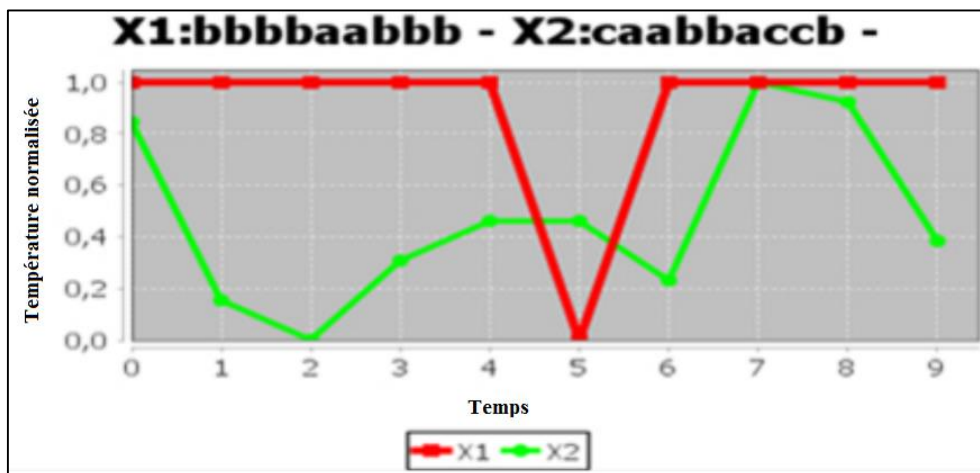
Figure 4.2. Représentation SAX de X1 et X2 avec normalisation.
