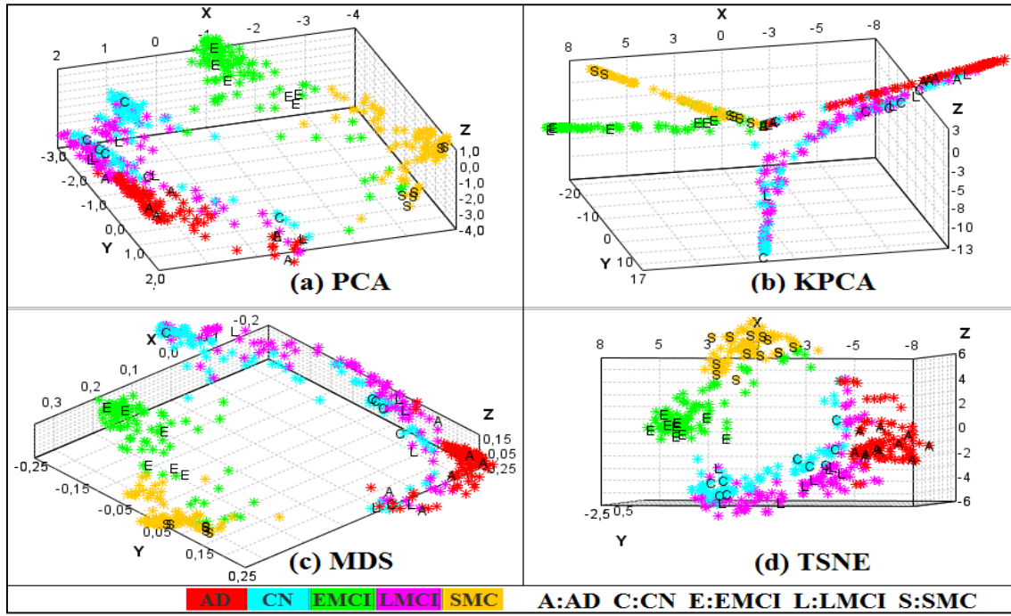
Figure 6.5. Visualisation de la réduction 3D du dernier fold de test. (a)PCA, (b)KPCA, (c)MDS et (d)TSNE.
