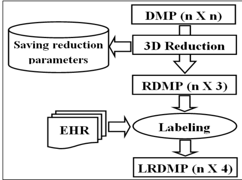
Figure 6.3. Processus de réduction de dimensionnalité.
