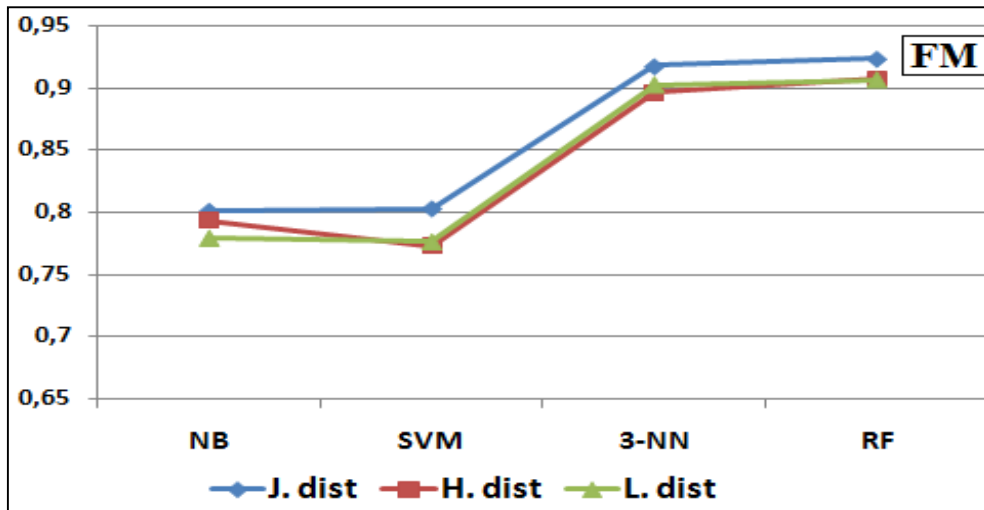
Figure 6.6. Comparaison de FM des classifications sur les données LRTSNE en fonction des distances choisies.
