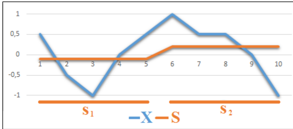
Figure 3.2. Exemple illustratif de la technique PAA.
