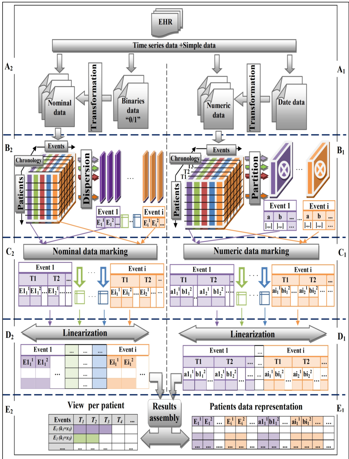
Figure 5.1. Modèle de représentation de données de la MP.
