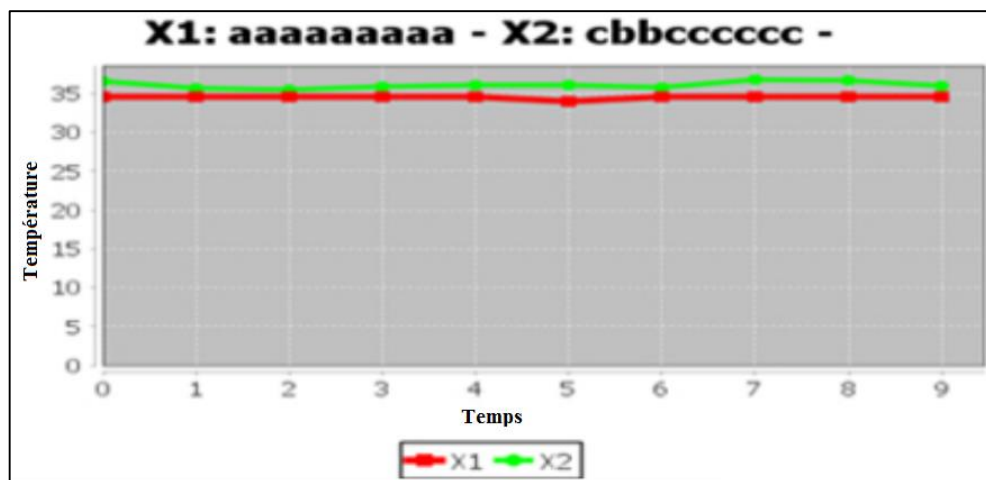
Figure 4.3. Représentation Multi-séries SAX de X1 et X2 sans normalisation.
