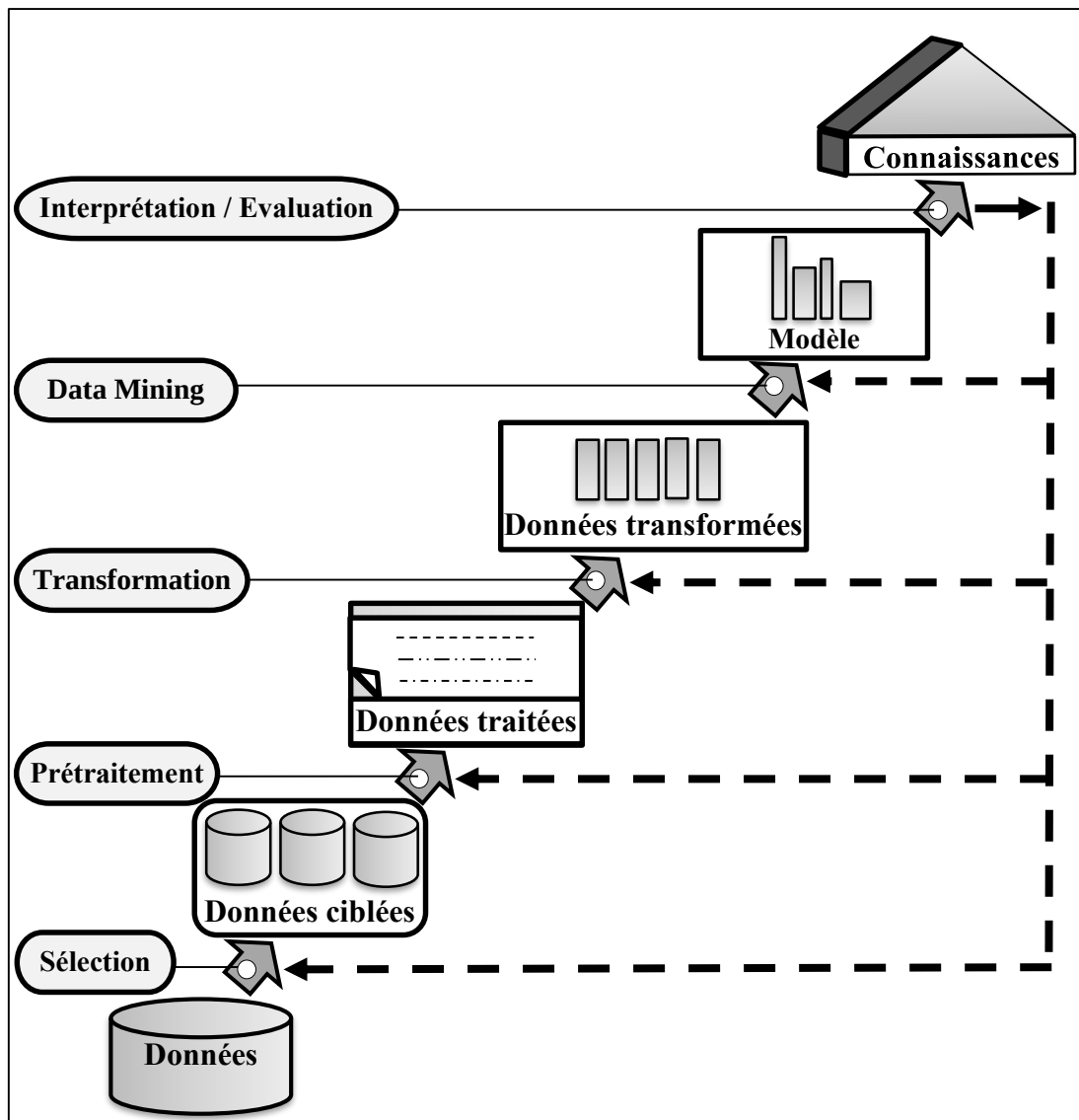
Figure 2.1. Étapes de processus de DM. (Fayyad et al., 1996).
