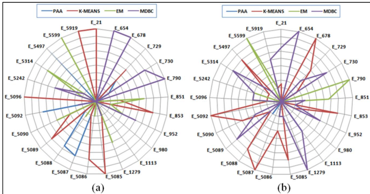
Figure 5.3. Illustration des techniques de clustering appropriées correspondant aux statistiques de : (a) l'inertie intraclasse, (b) l'inertie interclasse.
