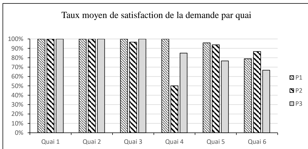
Figure 5. 15- Taux de satisfaction de la demande par quai en sortie de la simulation sur l'horizon de 3 mois
