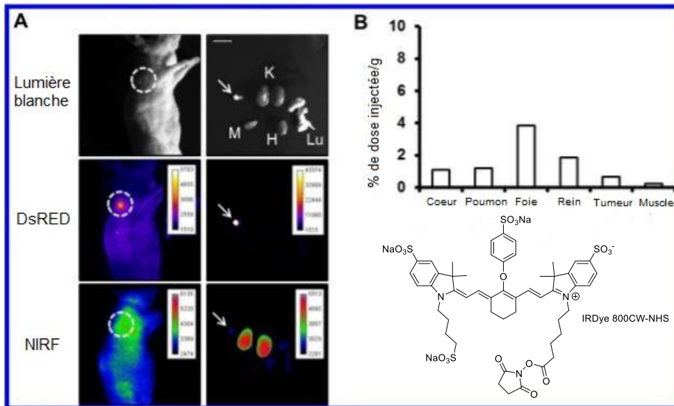
Figure 35 : A- Images à la lumière blanche, DSrED et proche IR 40h après l'injection de la sonde. B- Quantification de la sonde dans différents tissus. La flèche montre la tumeur excisée. K=rein, Lu=poumon, H=cœur et M=muscle. Echelle=1.6 cm
