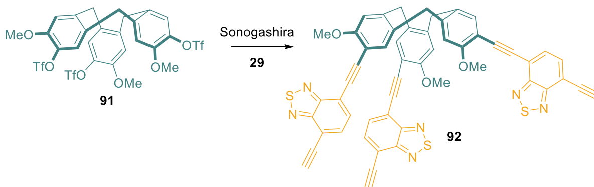
Schéma 66 : Synthèse composé 92
