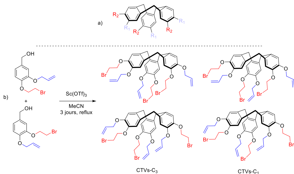
Figure 43 : a) CTV- C_1 avec inversion des groupements R_1 et R_2 - b) Synthèse des 4 stéréoisomères
