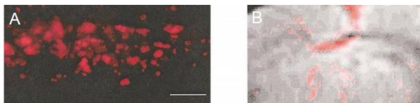
Figure 34 : A- Migration des cellules le long du corps calleux après une transplantation marquée avec la sonde GRID (50 \mu m). B- Superposition des images d'IRM et d'IO du site d'injection vers le corps calleux.
