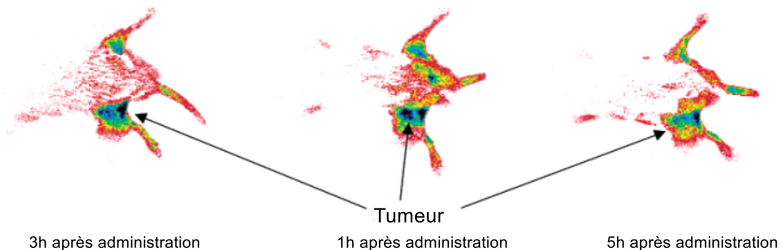
Figure 23 : Image optique de la sonde dérivée de la fluoescéine sur un rat porteur d'une tumeur CA20948
