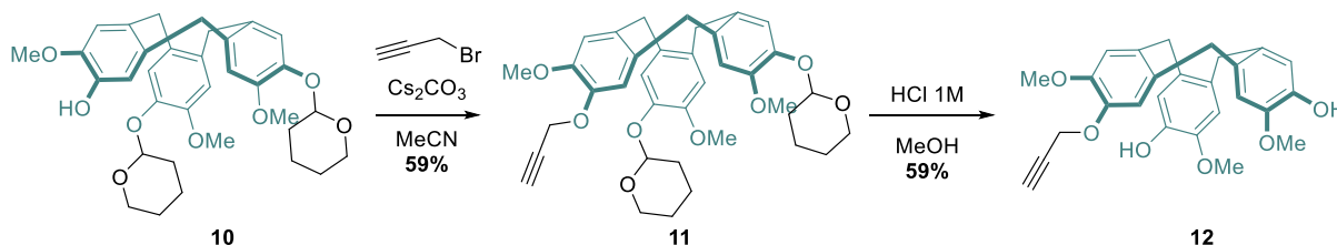
Schéma 44 : Synthèse des composés 11 et 12
