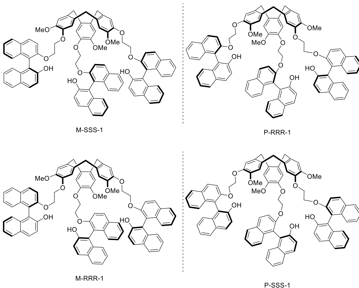
Figure 38 : Structure des CTVs couplés aux binaphtoles
