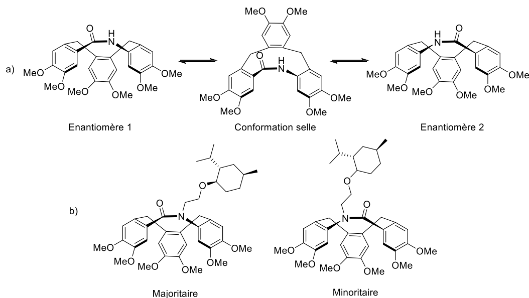
Figure 42 : a) Racémisation du CTV- C_1 lactame via les changements de conformation - b) Les deux diastéréoisomères du menthoxyimide
