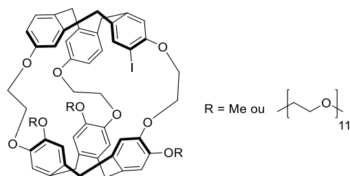
Schéma 23 : Cryptophane monofonctionné hydro-soluble
