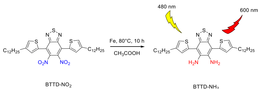
Schéma 8 : Réduction du BTTD-NO 2 et déclenchement de sa fluorescence
