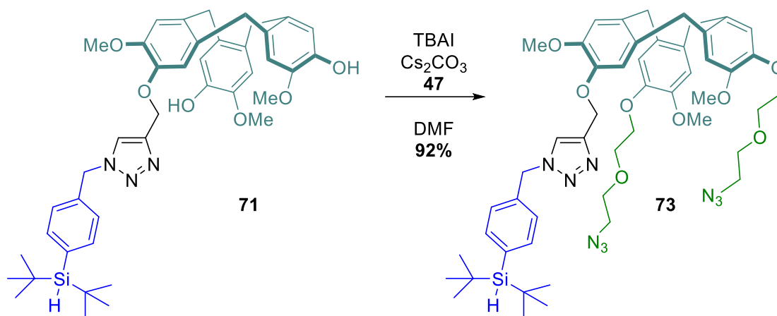
Schéma 59 : Synthèse du composé 73
