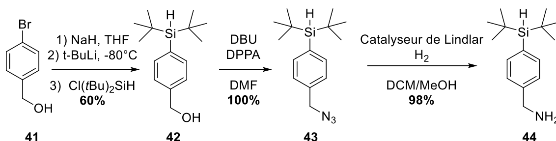
Schéma 28 : Synthèse de l'arylsilane NH 2 44
