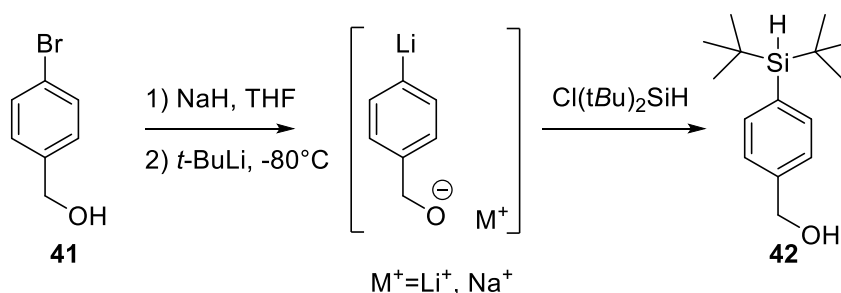
Schéma 29 : Synthèse du composé silylé 42
