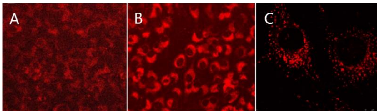
Figure 30 : Micrographie de fluorescence de cellules MG63 incubées avec le BTTD-NO 2 pendant 24 h dans des conditions normoxyques (A) et hypoxiques (B et C)
