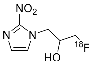
Figure 15 : Structure du [ 18 F]-FMISO
