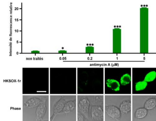
Figure 22 : Image représentative de cellules RAW267.7 co-incubées avec la sonde dérivée de la fluoescéine HXSOX-1r, avec un ajout graduel d'antimycine A pendant 30 min. Echelle = 10 μm
