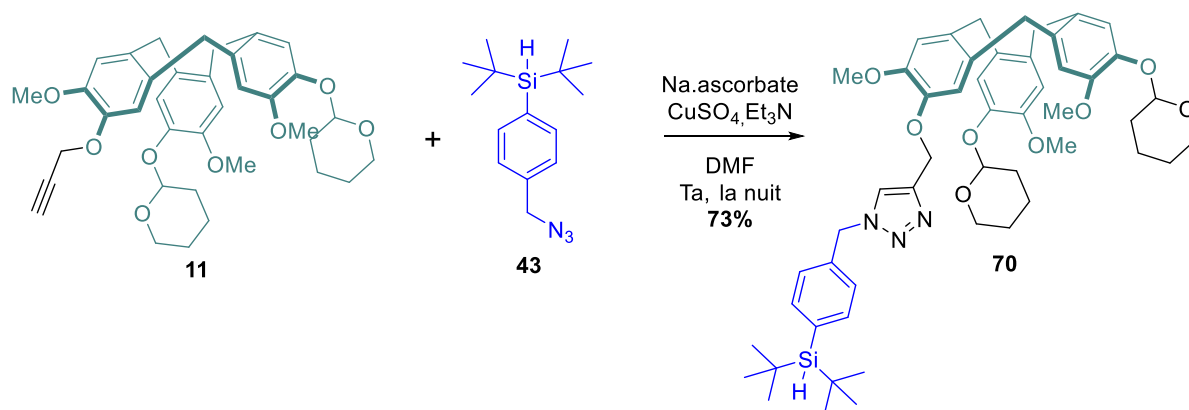
Schéma 55 : Synthèse du composé 70
