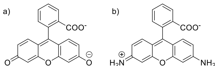
Figure 21 : a) Fluorescéine - b) Rhodamine
