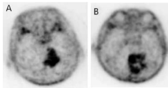
Figure 16 : Imagerie TEP avec la sonde [^{18}\text{F}] -FLT : A- gangliogliome du cervelet B- astrocytome pilocytaire
