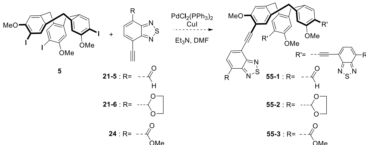
Schéma 38 : Couplage des BTDs sur le CTV I 5
