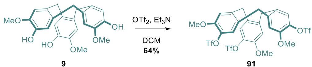
Schéma 65 : Synthèse du composé 91
