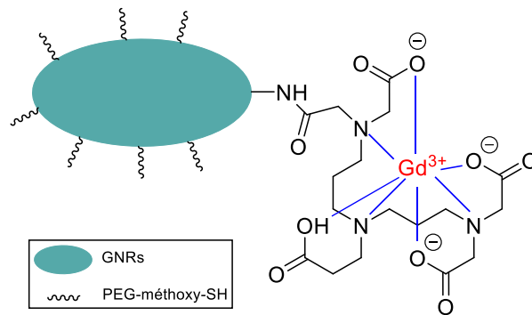
Schéma 9 : Structure de la sonde Gd III -GNRs
