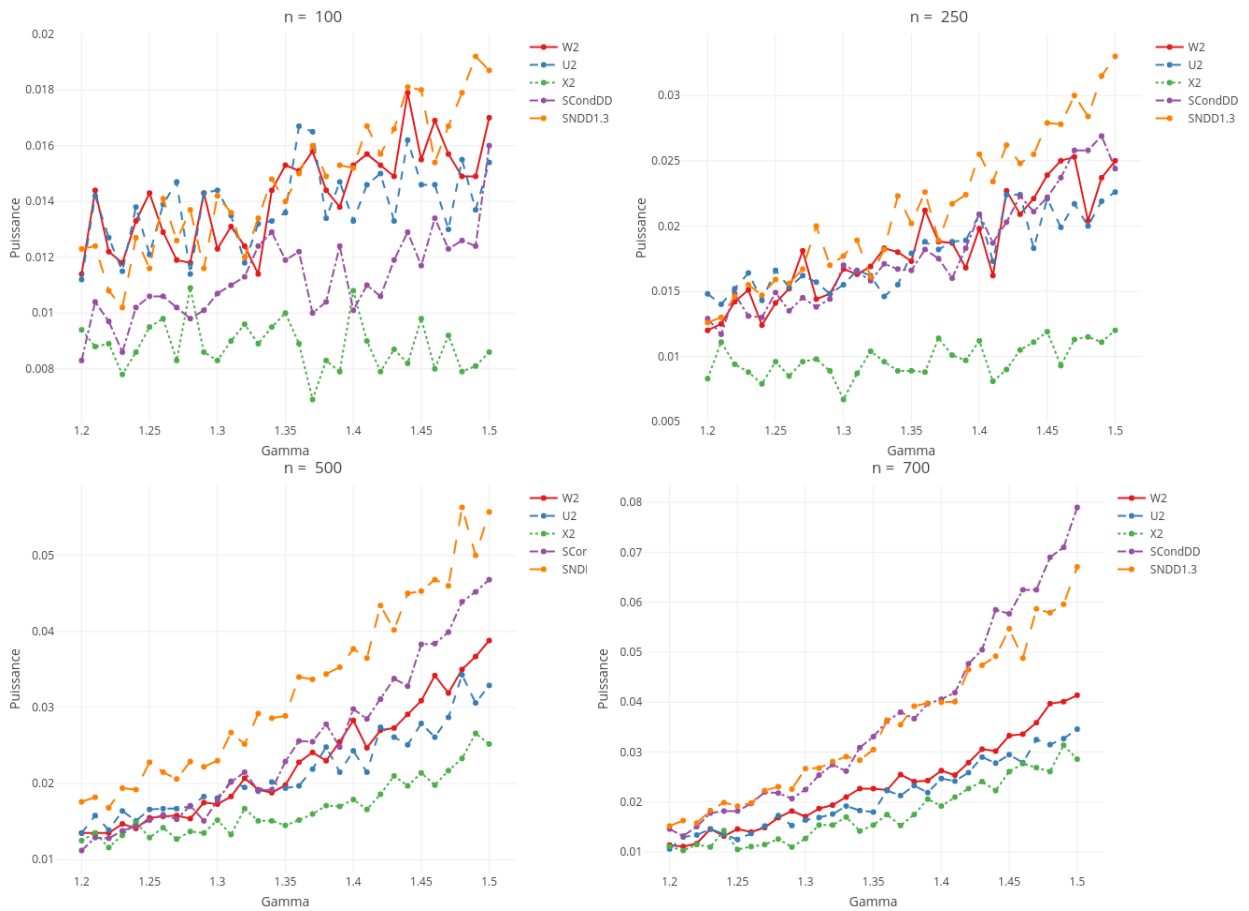
FIGURE 3.3.38 – Famille de Wong multiplicative : Courbes de puissance, en fonction du paramètre \gamma , de divers tests (basés sur 10000 répétitions) au niveau 5% pour l’hypothèse nulle de la loi \mathcal{B}_{(1,2)} . Les tests représentés sont : W^2 (couleur rouge), \chi^2 (couleur verte), U^2 (couleur bleue), \mathcal{S}_{NDD} (couleur orange) et \mathcal{S}_{Cond,DD} (couleur violette) dont les expressions se trouvent à la Section 3.3.3. Les quantiles de référence sont approximés par Monte-Carlo en utilisant 1000000 répétitions.
