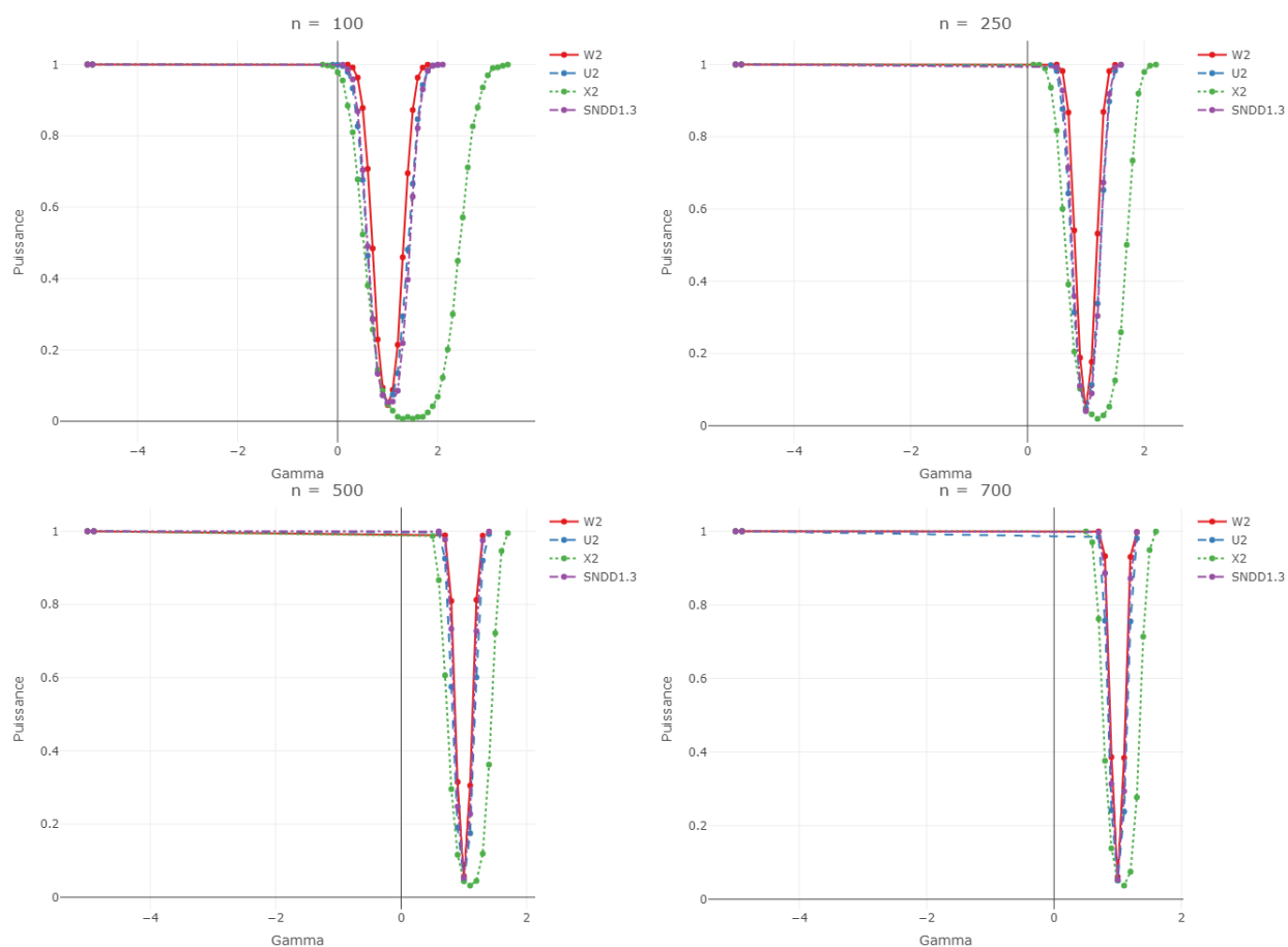
FIGURE A.2.11 – Newcomb-Benford Généralisée sachant Benford (\mathcal{GB}_1(\gamma), \mathcal{B}_{(2|1)}) : Courbes de puissance en fonction du paramètre \gamma , des tests \mathcal{S}_{NDD} , U^2 , \chi^2 , W^2 (basés sur 10000 répliquations) au niveau 5% pour l’hypothèse nulle de la loi \mathcal{B}_{(1,2)} . Les tests représentés sont : W^2 (couleur rouge), \chi^2 (couleur verte), U^2 (couleur bleue), \mathcal{S}_{NDD} (couleur violette) dont les expressions se trouvent à la Section 3.3.3. Les quantiles de référence sont approximés par Monte-Carlo en utilisant 1000000 répétitions.
