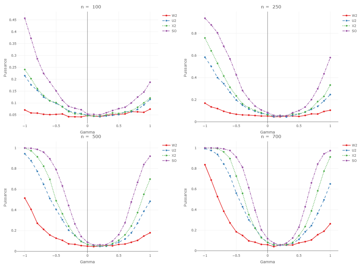
FIGURE 3.3.44 – Famille des copules : Copule Benford Benford C(\gamma, \mathcal{B}_1, \mathcal{B}_2) : Courbes de puissance en fonction du paramètre \gamma , de divers tests (basés sur 10000 répétitions) au niveau 5% pour l'hypothèse nulle de la loi Newcomb-Benford \mathcal{B}_{(1,2)} . Les tests représentés sont : W^2 (couleur rouge), \chi^2 (couleur verte), U^2 (couleur bleue) et STO (couleur violette) dont les expressions se trouvent respectivement aux Sections 3.3.3 et 3.3.18. Les quantiles de référence sont approximés par Monte-Carlo en utilisant 1000000 répétitions.
