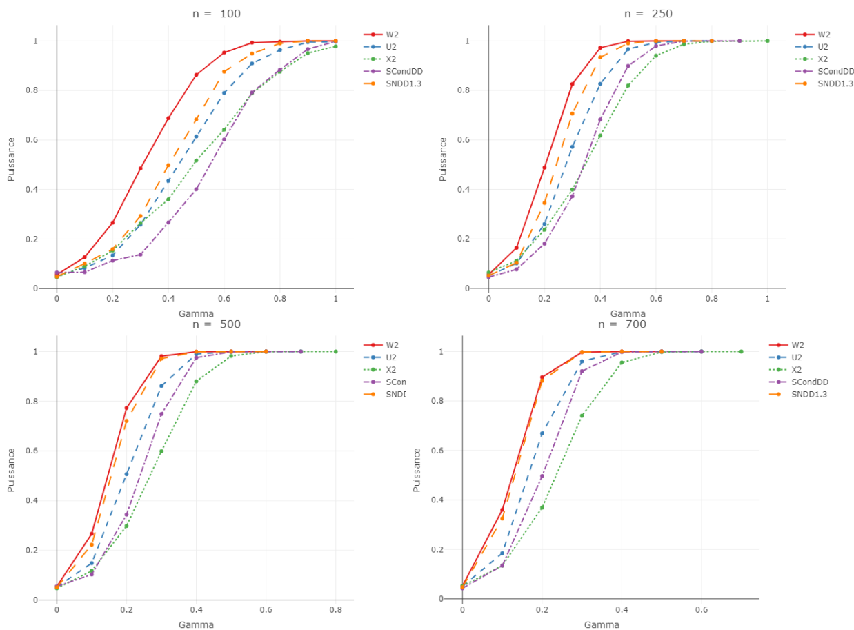
FIGURE 3.3.29 – Mixture Benford Uniforme (1 - \gamma)\mathcal{B}_{(1,2)} + \gamma U_{[10,99]} : Courbes de puissance, en fonction du paramètre \gamma , de divers tests (basés sur 10000 répliques) au niveau 5% pour l'hypothèse nulle de la loi \mathcal{B}_{(1,2)} . Les tests représentés sont : W^2 (couleur rouge), \chi^2 (couleur verte) , U^2 (couleur bleue), \mathcal{S}_{NDD} (couleur orange) et \mathcal{S}_{Cond,DD} (couleur violette) dont les expressions se trouvent à la Section 3.3.3. Les quantiles de référence sont approximés par Monte-Carlo en utilisant 1000000 répétitions.
