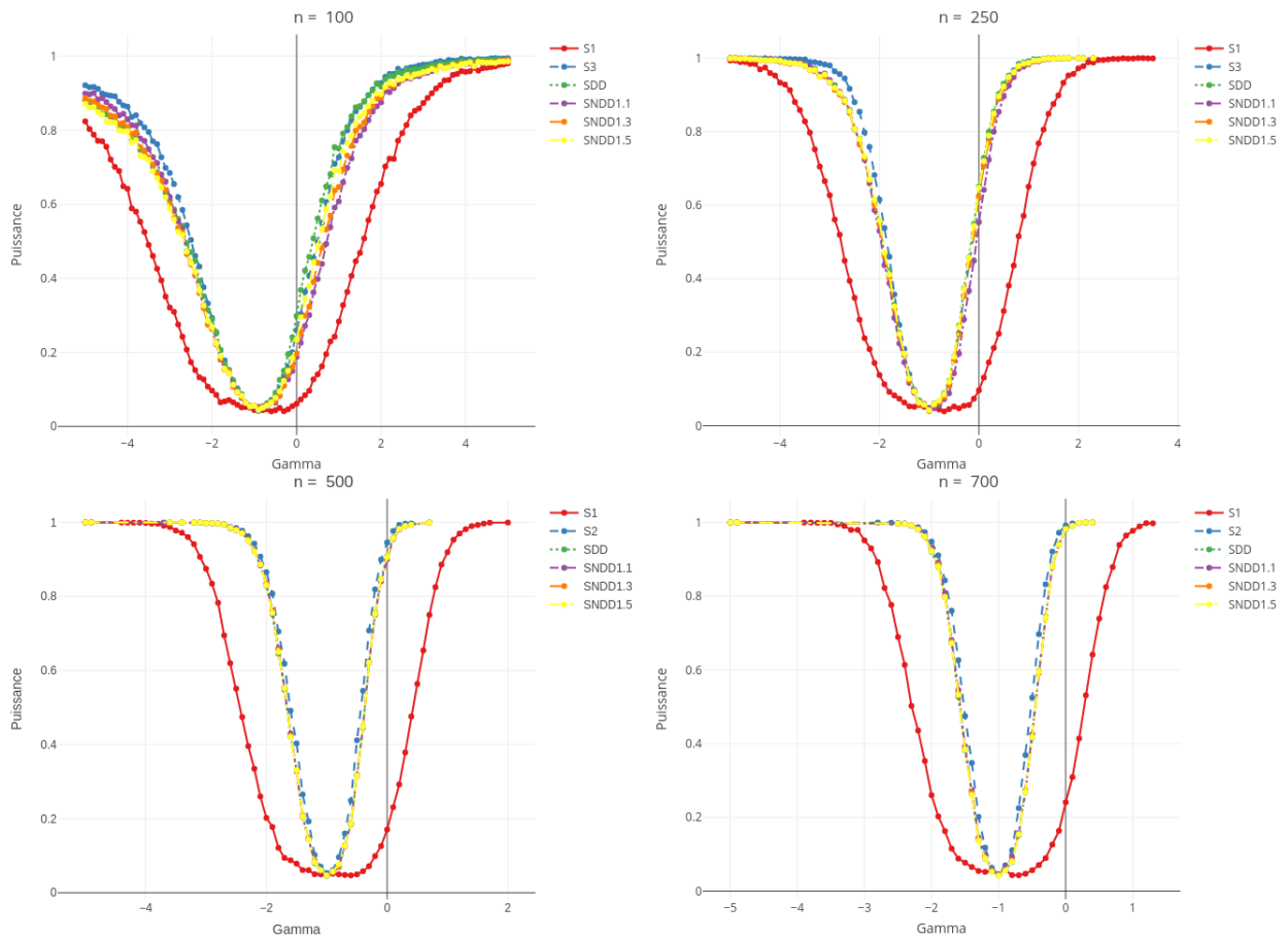
FIGURE A.1.10 – Rodriguez sachant Rodriguez (\mathcal{R}_1(\gamma), \mathcal{R}_{(2|1)}(\gamma)) : Courbes de puissance en fonction du paramètre \gamma , de divers tests (basés sur 10000 réplifications) au niveau 5% pour l’hypothèse nulle de loi Newcomb - Benford \mathcal{B}_{(1,2)} . Les tests représentés sont : le meilleur entre \mathcal{S}_i, i \in \{1, \dots, 5\} (couleur rouge), \mathcal{S}_{DD} (couleur verte), le pire entre \mathcal{S}_i, i \in \{1, \dots, 5\} (couleur bleue), \mathcal{S}_{NDD1,1} avec c = 1.1 (couleur violette), \mathcal{S}_{NDD1,3} avec c = 1.3 (couleur orange) et \mathcal{S}_{NDD1,5} avec c = 1.5 (couleur jaune), dont les expressions se trouvent à la Section 3.3.3. Les quantiles de référence sont approximés par Monte-Carlo en utilisant 1000000 répétitions. Lorsque \gamma = 0 , on retombe sur la loi \mathcal{B}_{(1,2)} sous l’hypothèse H_0 .
