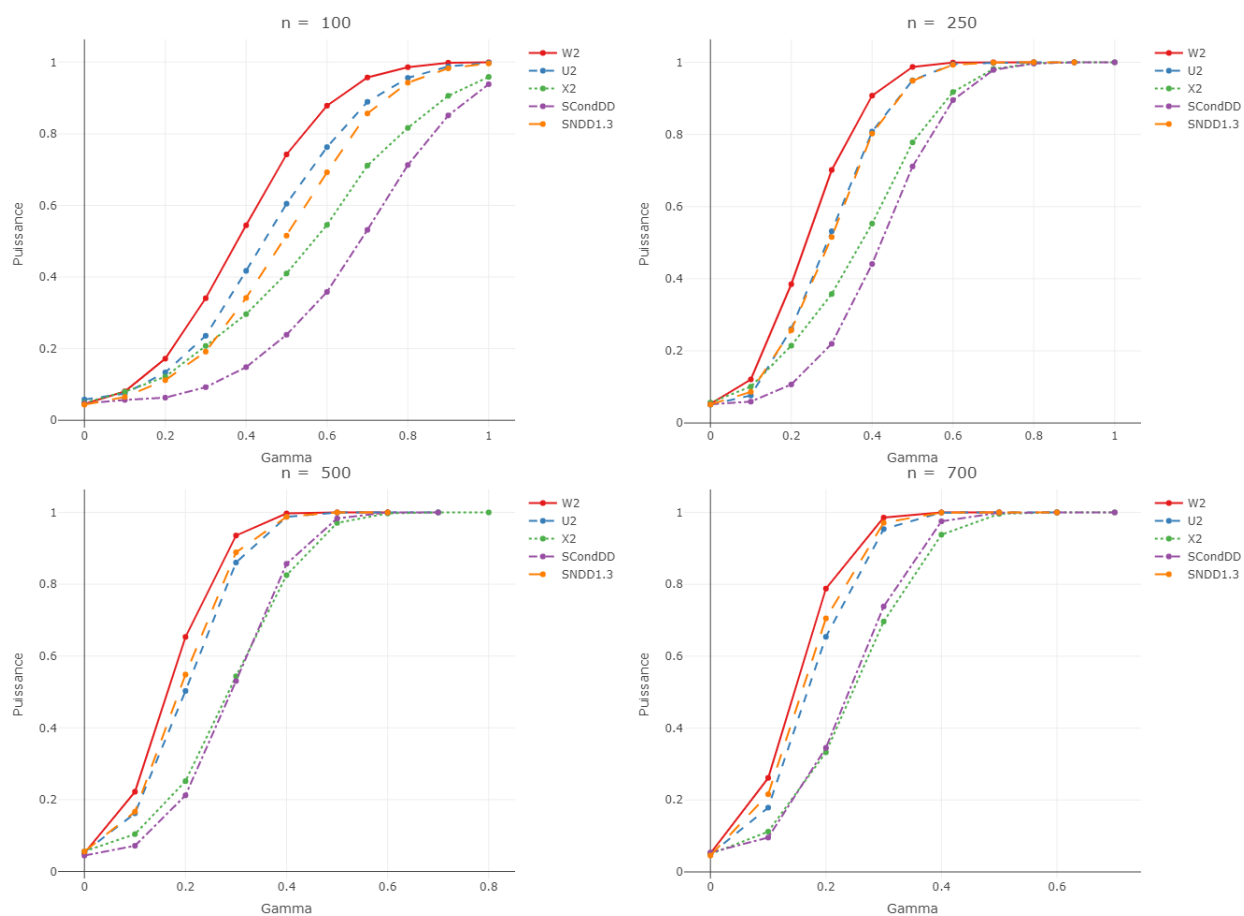
FIGURE A.4.1 – Mixture Benford Hill (1 - \gamma)\mathcal{B}_{(1,2)} + \gamma\mathcal{H}_{(1,2)} : Courbes de puissance, en fonction du paramètre \gamma , de divers tests (basés sur 10000 répliquions) au niveau 5% pour l’hypothèse nulle de la loi \mathcal{B}_{(1,2)} . Les tests représentés sont : W^2 (couleur rouge), \chi^2 (couleur verte) , U^2 (couleur bleue), \mathcal{S}_{NDD} (couleur orange) et \mathcal{S}_{Cond,DD} (couleur violette) dont les expressions se trouvent à la Section 3.3.3. Les quantiles de référence sont approximés par Monte-Carlo en utilisant 1000000 répétitions.
