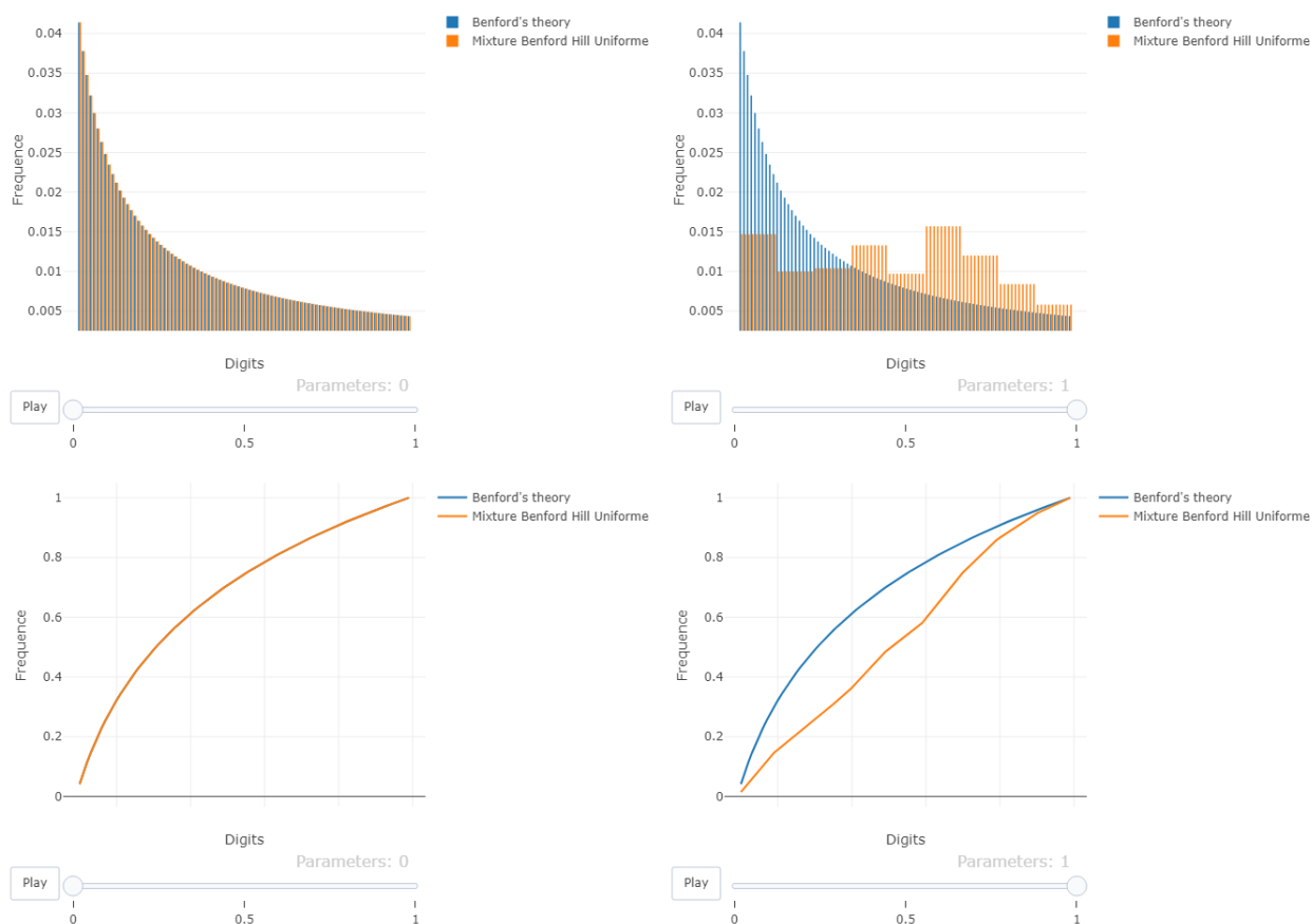
FIGURE A.3.4 – Mixture Benford Hill Uniforme (1 - \gamma)\mathcal{B}_{(1,2)} + \gamma \mathcal{H}_1 \otimes U_{[0,9]} : Figures de hauts : Comparaison des fonctions de densités de \mathcal{B}_{(1,2)} (en bleu) et de la loi alternative (en orange) pour \gamma = 0 à gauche et \gamma = 1 à droite. Figures de bas : Comparaison des fonctions de répartition de \mathcal{B}_{(1,2)} (en bleu) et de la loi alternative (en orange) pour \gamma = 0 à gauche et \gamma = 1 à droite.
