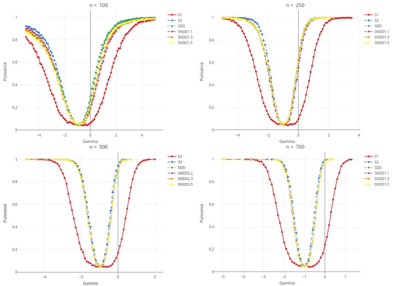
FIGURE A.1.10 – Rodriguez sachant Rodriguez ( \mathcal{R}_1(\gamma), \mathcal{R}_{(2|1)}(\gamma) ) : Courbes de puissance en fonction du paramètre \gamma , de divers tests (basés sur 10000 réplifications) au niveau 5% pour l’hypothèse nulle de loi Newcomb - Benford \mathcal{B}_{(1,2)} . Les tests représentés sont : le meilleur entre \mathcal{S}_i, i \in \{1, \dots, 5\} (couleur rouge), \mathcal{S}_{DD} (couleur verte), le pire entre \mathcal{S}_i, i \in \{1, \dots, 5\} (couleur bleue), \mathcal{S}_{NDD1.1} avec c = 1.1 (couleur violette), \mathcal{S}_{NDD1.3} avec c = 1.3 (couleur orange) et \mathcal{S}_{NDD1.5} avec c = 1.5 (couleur jaune), dont les expressions se trouvent à la Section 3.3.3. Les quantiles de référence sont approximés par Monte-Carlo en utilisant 1000000 répétitions. Lorsque \gamma = 0 , on retombe sur la loi \mathcal{B}_{(1,2)} sous l’hypothèse H_0 .
