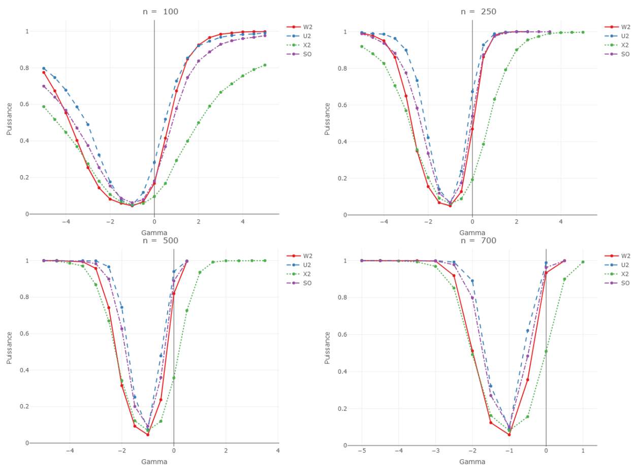
FIGURE 3.3.42 – Famille des indépendances : Indépendance Rodriguez Rodriguez ( \mathcal{R}_1(\gamma) \perp \mathcal{R}_2(\gamma) ) : Courbes de puissance en fonction du paramètre \gamma , de divers tests (basés sur 10000 répétitions) au niveau 5% pour l'hypothèse nulle de la loi Newcomb-Benford \mathcal{B}_{(1,2)} . Les tests représentés sont : W^2 (couleur rouge), \chi^2 (couleur verte), U^2 (couleur bleue) et STO (couleur violette) dont les expressions se trouvent respectivement aux Sections 3.3.3 et 3.3.18. Les quantiles de référence sont approximés par Monte-Carlo en utilisant 1000000 répétitions.
