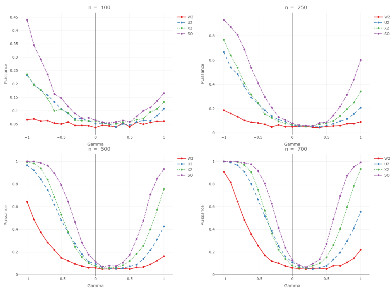
FIGURE 3.3.54 – Copule Benford Stigler C(\gamma, \mathcal{B}_1, S_2) : Courbes de puissance, en fonction du paramètre \gamma , de divers tests (basés sur 10000 répétitions) au niveau 5% pour l'hypothèse nulle de la loi Newcomb-Benford \mathcal{B}_{(1,2)} . Les tests représentés sont : W^2 (couleur rouge), \chi^2 (couleur verte), U^2 (couleur bleue) et STO (couleur violette) dont les expressions se trouvent respectivement aux Sections 3.3.3 et 3.3.18. Les quantiles de référence sont approximés par Monte-Carlo en utilisant 1000000 répétitions.
