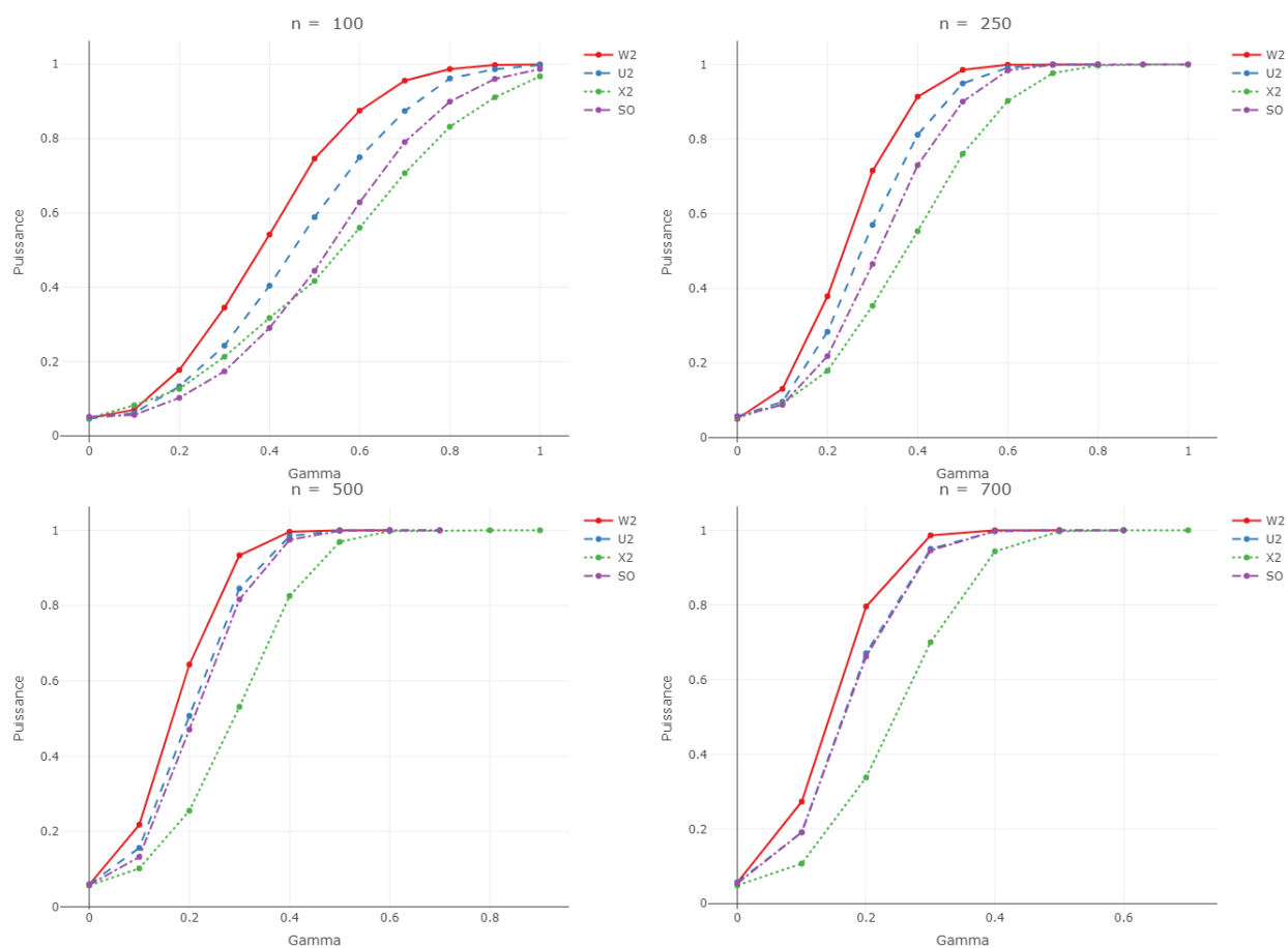
FIGURE 3.3.49 – Mixture Benford Hill (1 - \gamma)\mathcal{B}_{(1,2)} + \gamma\mathcal{H}_{(1,2)} : Courbes de puissance, en fonction du paramètre \gamma , de divers tests (basés sur 10000 répliquions) au niveau 5% pour l'hypothèse nulle de la loi Newcomb-Benford \mathcal{B}_{(1,2)} . Les tests représentés sont : W^2 (couleur rouge), \chi^2 (couleur verte), U^2 (couleur bleue) et STO (couleur violette) dont les expressions se trouvent respectivement aux Sections 3.3.3 et 3.3.18. Les quantiles de référence sont approximés par Monte-Carlo en utilisant 1000000 répétitions.
