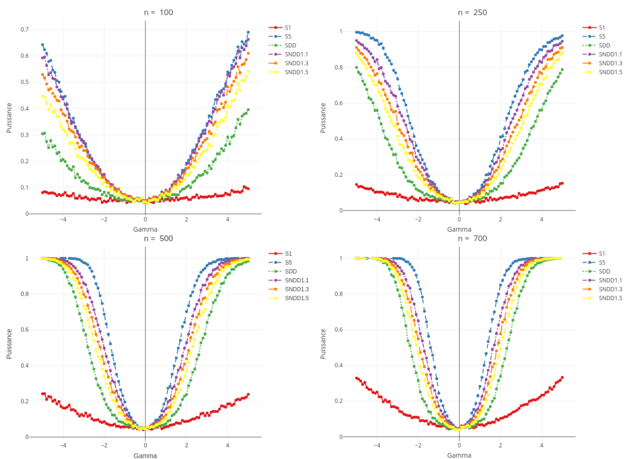
FIGURE A.1.12 – Benford sachant Newcomb-Benford Généralisée (\mathcal{B}_1, \mathcal{GB}_{(2|1)}(\gamma)) : Courbes de puissance en fonction du paramètre \gamma , de divers tests (basés sur 10000 répétitions) au niveau 5% pour l'hypothèse nulle de loi Newcomb - Benford \mathcal{B}_{(1,2)} . Les tests représentés sont : le meilleur entre \mathcal{S}_i, i \in \{1, \dots, 5\} (couleur rouge), \mathcal{S}_{DD} (couleur verte), le pire entre \mathcal{S}_i, i \in \{1, \dots, 5\} (couleur bleue), \mathcal{S}_{NDD1,1} avec c = 1.1 (couleur violette), \mathcal{S}_{NDD1,3} avec c = 1.3 (couleur orange) et \mathcal{S}_{NDD1,5} avec c = 1.5 (couleur jaune), dont les expressions se trouvent à la Section 3.3.3. Les quantiles de référence sont approximés par Monte-Carlo en utilisant 1000000 répétitions. Lorsque \gamma = 0 , on retombe sur la loi \mathcal{B}_{(1,2)} sous l'hypothèse H_0 .
