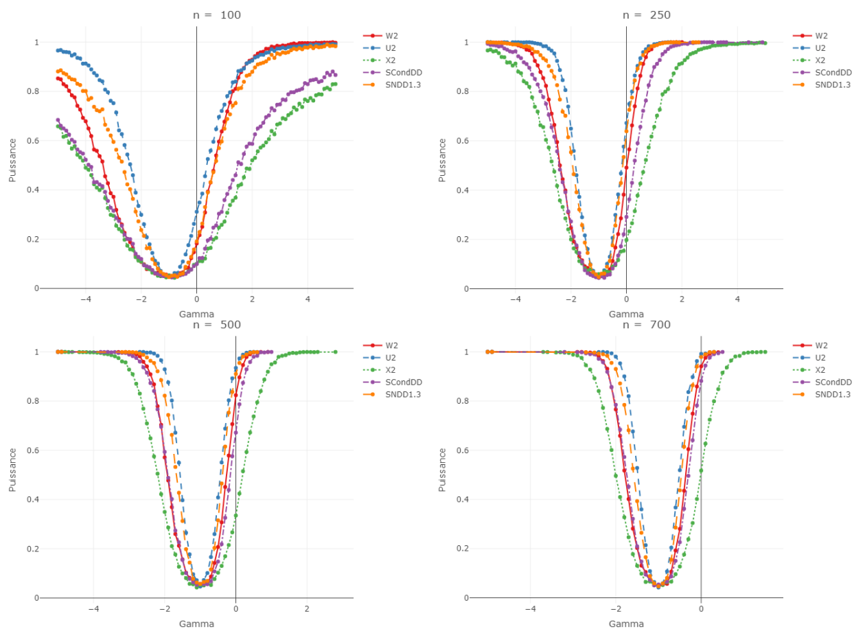
FIGURE A.4.10 – Rodriguez sachant Rodriguez (\mathcal{R}_1(\gamma), \mathcal{R}_{(2|1)}(\gamma)) : Courbes de puissance, en fonction du paramètre \gamma , de divers tests (basés sur 10000 répliquions) au niveau 5% pour l’hypothèse nulle de la loi \mathcal{B}_{(1,2)} . Les tests représentés sont : W^2 (couleur rouge), \chi^2 (couleur verte), U^2 (couleur bleue), \mathcal{S}_{NDD} (couleur orange) et \mathcal{S}_{Cond,DD} (couleur violette) dont les expressions se trouvent à la Section 3.3.3. Les quantiles de référence sont approximés par Monte-Carlo en utilisant 1000000 répétitions.
