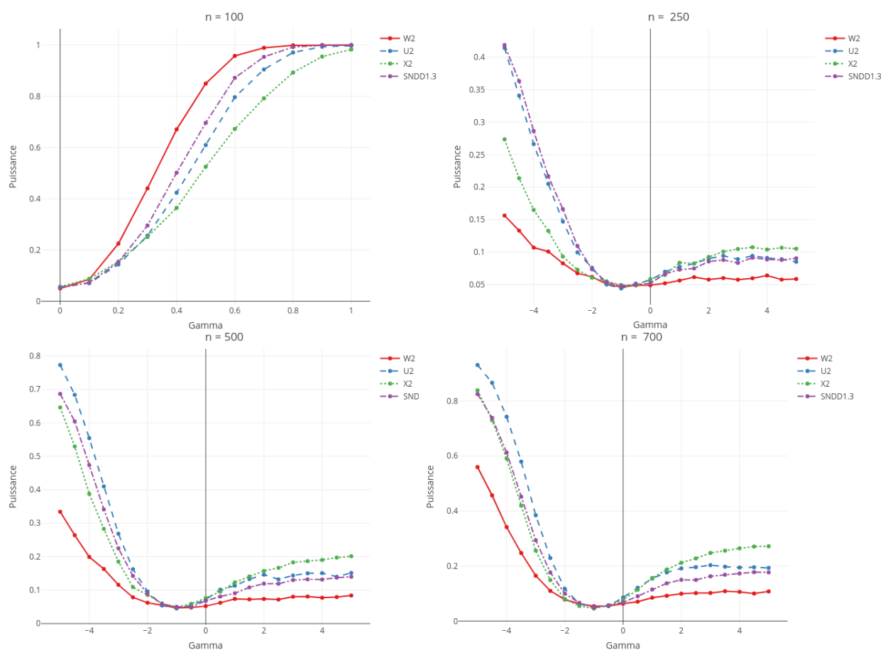
FIGURE 3.3.15 – Famille des conditionnelles : Rodriguez sachant Benford (\mathcal{B}_1, \mathcal{R}_{(2|1)}(\gamma)) : Courbes de puissance en fonction du paramètre \gamma , des tests \mathcal{S}_{NDD} , U^2 , \chi^2 , W^2 (basés sur 10000 répliquions) au niveau 5% pour l'hypothèse nulle de la loi \mathcal{B}_{(1,2)} . Les tests représentés sont : W^2 (couleur rouge), \chi^2 (couleur verte), U^2 (couleur bleue), \mathcal{S}_{NDD} (couleur violette) dont les expressions se trouvent à la Section 3.3.3. Les quantiles de référence sont approximés par Monte-Carlo en utilisant 1000000 répétitions.
