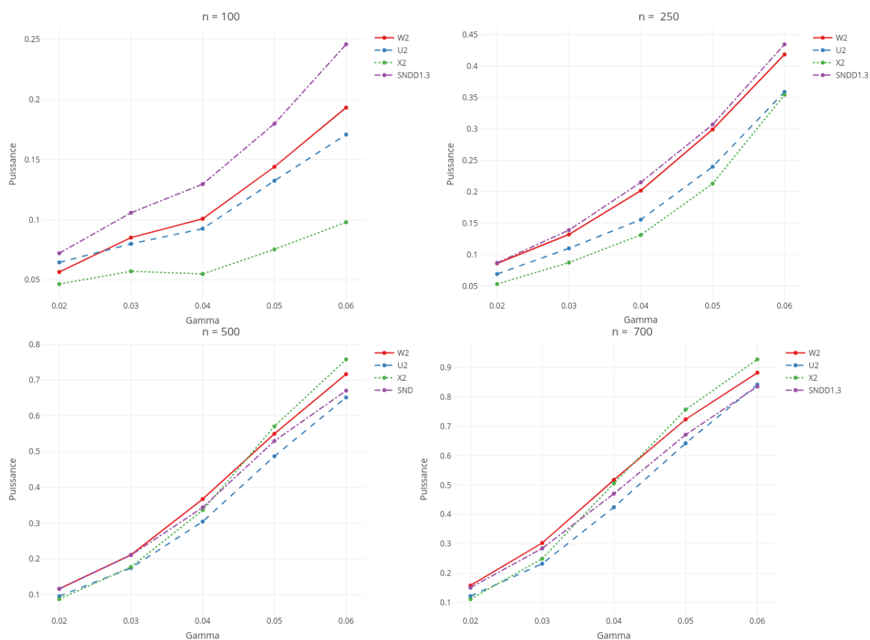
FIGURE 3.3.17 – Famille de Wong additive : Courbes de puissance en fonction du paramètre \gamma , des tests \mathcal{S}_{NDD} , U^2 , \chi^2 , W^2 (basés sur 10000 répétitions) au niveau 5% pour l'hypothèse nulle de la loi \mathcal{B}_{(1,2)} . Les tests représentés sont : W^2 (couleur rouge), \chi^2 (couleur verte), U^2 (couleur bleue), \mathcal{S}_{NDD} (couleur violette) dont les expressions se trouvent à la Section 3.3.3. Les quantiles de référence sont approximés par Monte-Carlo en utilisant 1000000 répétitions.
