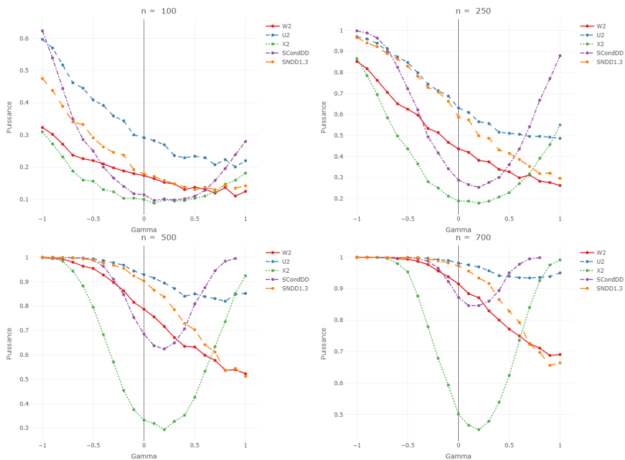
FIGURE A.4.7 – Copule Stigler Benford C(\gamma, \mathcal{S}_1, \mathcal{B}_2) : Courbes de puissance, en fonction du paramètre \gamma , de divers tests (basés sur 10000 répliquions) au niveau 5% pour l’hypothèse nulle de la loi \mathcal{B}_{(1,2)} . Les tests représentés sont : W^2 (couleur rouge), \chi^2 (couleur verte) , U^2 (couleur bleue), \mathcal{S}_{NDD} (couleur orange) et \mathcal{S}_{Cond,DD} (couleur violette) dont les expressions se trouvent à la Section 3.3.3. Les quantiles de référence sont approximés par Monte-Carlo en utilisant 1000000 répétitions.
