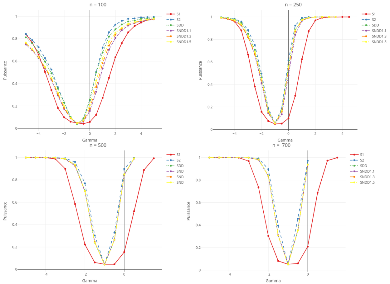
FIGURE 3.3.8 – Benford sachant Rodriguez (\mathcal{R}_1(\gamma), \mathcal{B}_{(2|1)}(\gamma)) : Courbes de puissance en fonction du paramètre \gamma , de divers tests (basés sur 10000 répétitions) au niveau 5% pour l'hypothèse nulle de loi Newcomb - Benford \mathcal{B}_{(1,2)} . Les tests représentés sont : le meilleur entre \mathcal{S}_i , i \in \{1, \dots, 5\} (couleur rouge), \mathcal{S}_{DD} (couleur verte), le pire entre \mathcal{S}_i , i \in \{1, \dots, 5\} (couleur bleue), \mathcal{S}_{NDD1,1} avec c = 1.1 (couleur violette), \mathcal{S}_{NDD1,3} avec c = 1.3 (couleur orange) et \mathcal{S}_{NDD1,5} avec c = 1.5 (couleur jaune), dont les expressions se trouvent à la Section 3.3.3. Les quantiles de référence sont approximés par Monte-Carlo en utilisant 1000000 répétitions. Lorsque \gamma = 0 , on retombe sur la loi \mathcal{B}_{(1,2)} sous l'hypothèse H_0 .
