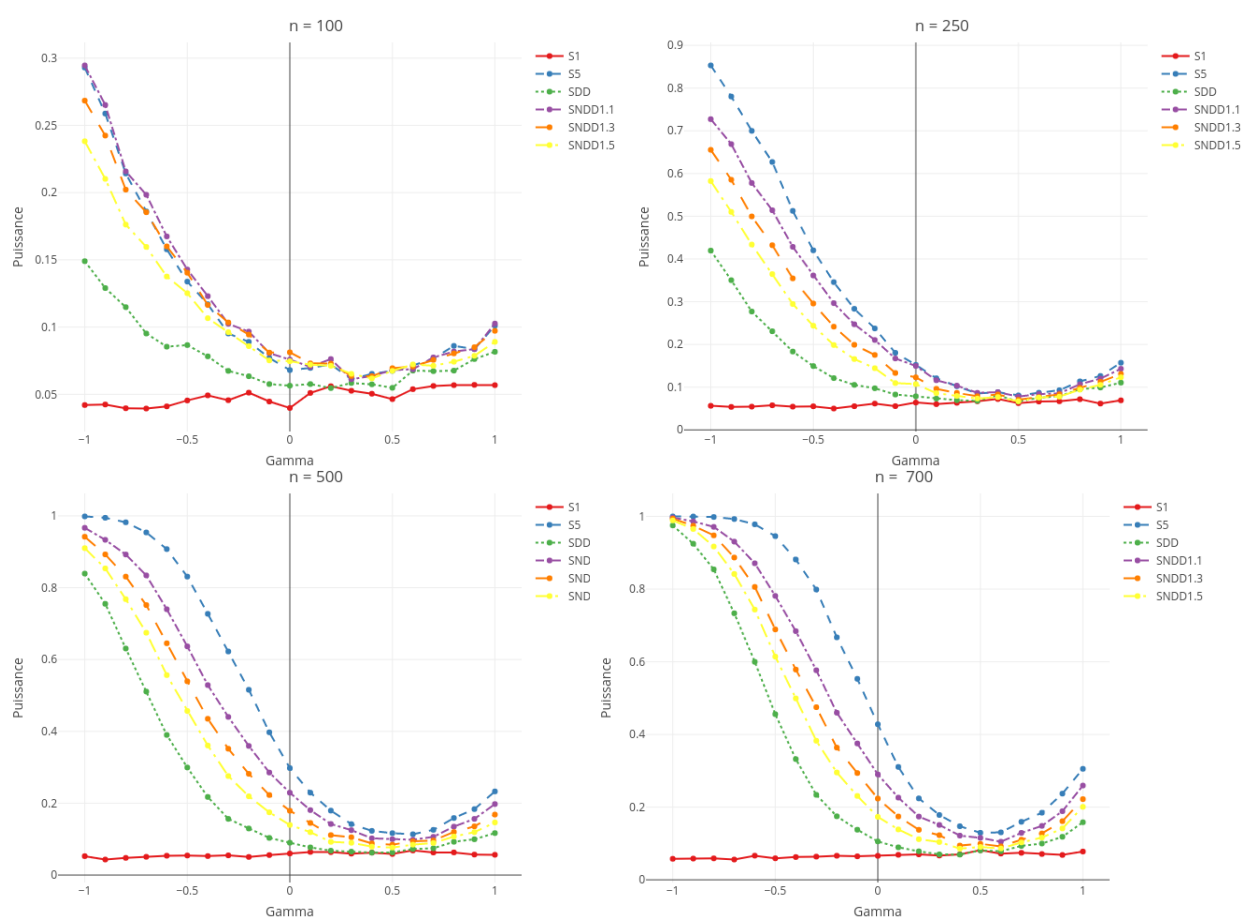
FIGURE 3.3.5 – Copule Benford Hill C(\gamma, \mathcal{B}_1, H_2) : Courbes de puissance en fonction du paramètre \gamma , de divers tests (basés sur 10000 répétitions) au niveau 5% pour l'hypothèse nulle de loi Newcomb - Benford \mathcal{B}_{(1,2)} . Les tests représentés sont : le meilleur entre \mathcal{S}_i, i \in \{1, \dots, 5\} (couleur rouge), \mathcal{S}_{DD} (couleur verte), le pire entre \mathcal{S}_i, i \in \{1, \dots, 5\} (couleur bleue), \mathcal{S}_{NDD1.1} avec c = 1.1 (couleur violette), \mathcal{S}_{NDD1.3} avec c = 1.3 (couleur orange) et \mathcal{S}_{NDD1.5} avec c = 1.5 (couleur jaune), dont les expressions se trouvent à la Section 3.3.3. Les quantiles de référence sont approximés par Monte-Carlo en utilisant 1000000 répétitions. Lorsque \gamma = 0 , on retombe sur la loi \mathcal{B}_{(1,2)} sous l'hypothèse H_0 .
