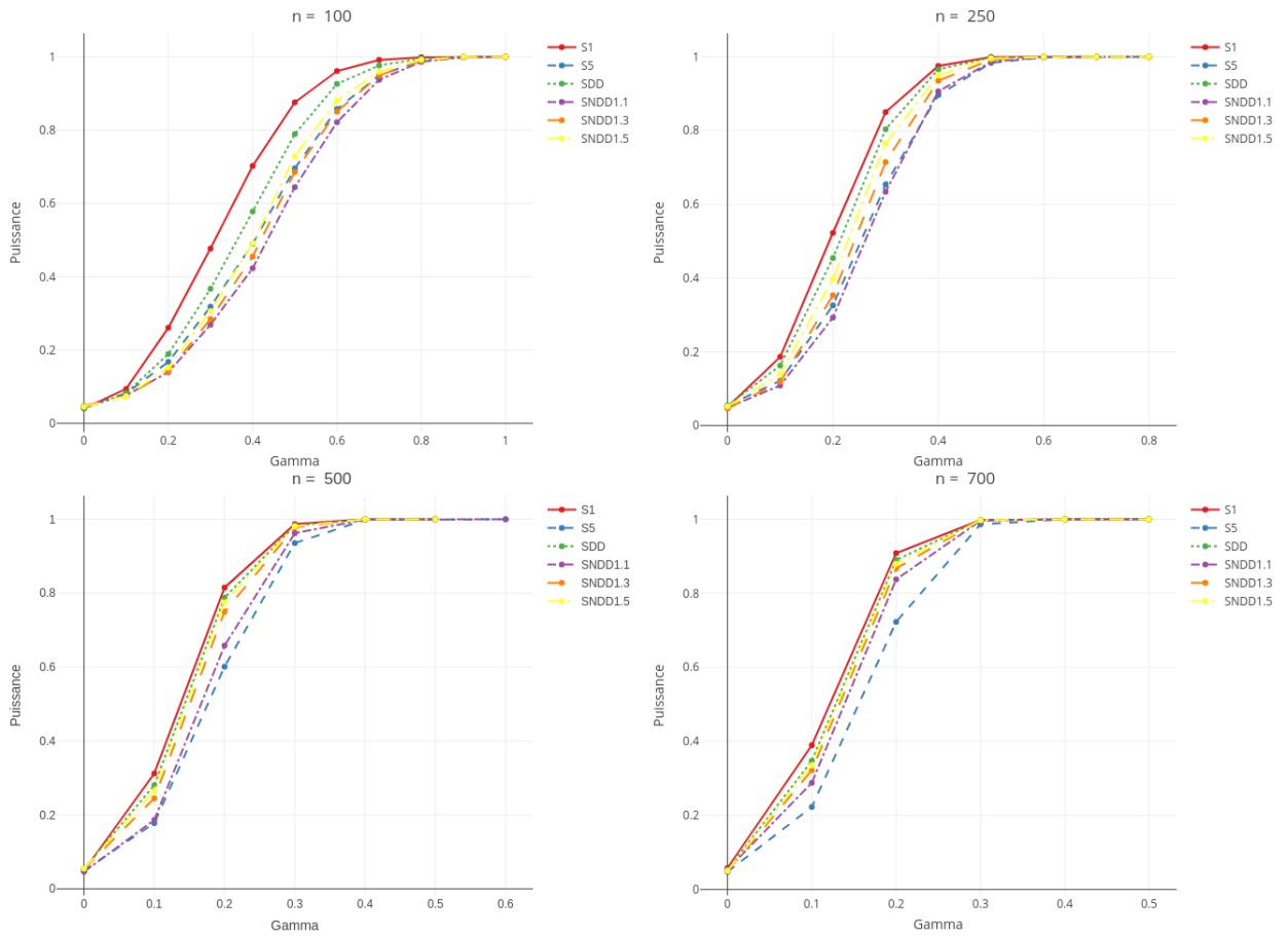
FIGURE A.1.5 – Mixture Benford Uniforme Hill (1-\gamma)\mathcal{B}_{(1,2)}+\gamma(1-\gamma)U_{[1,9]}\otimes\mathcal{H}_2 : Courbes de puissance en fonction du paramètre \gamma , de divers tests (basés sur 10000 répétitions) au niveau 5% pour l’hypothèse nulle de loi Newcomb - Benford \mathcal{B}_{(1,2)} . Les tests représentés sont : le meilleur entre \mathcal{S}_i, i \in \{1, \dots, 5\} (couleur rouge), \mathcal{S}_{DD} (couleur verte) , le pire entre \mathcal{S}_i, i \in \{1, \dots, 5\} (couleur bleue), \mathcal{S}_{NDD1,1} avec c = 1.1 (couleur violette) , \mathcal{S}_{NDD1,3} avec c = 1.3 (couleur orange) et \mathcal{S}_{NDD1,5} avec c = 1.5 (couleur jaune), dont les expressions se trouvent à la Section 3.3.3. Les quantiles de référence sont approximés par Monte-Carlo en utilisant 1000000 répétitions. Lorsque \gamma = 0 , on retombe sur la loi \mathcal{B}_{(1,2)} sous l’hypothèse H_0 .
