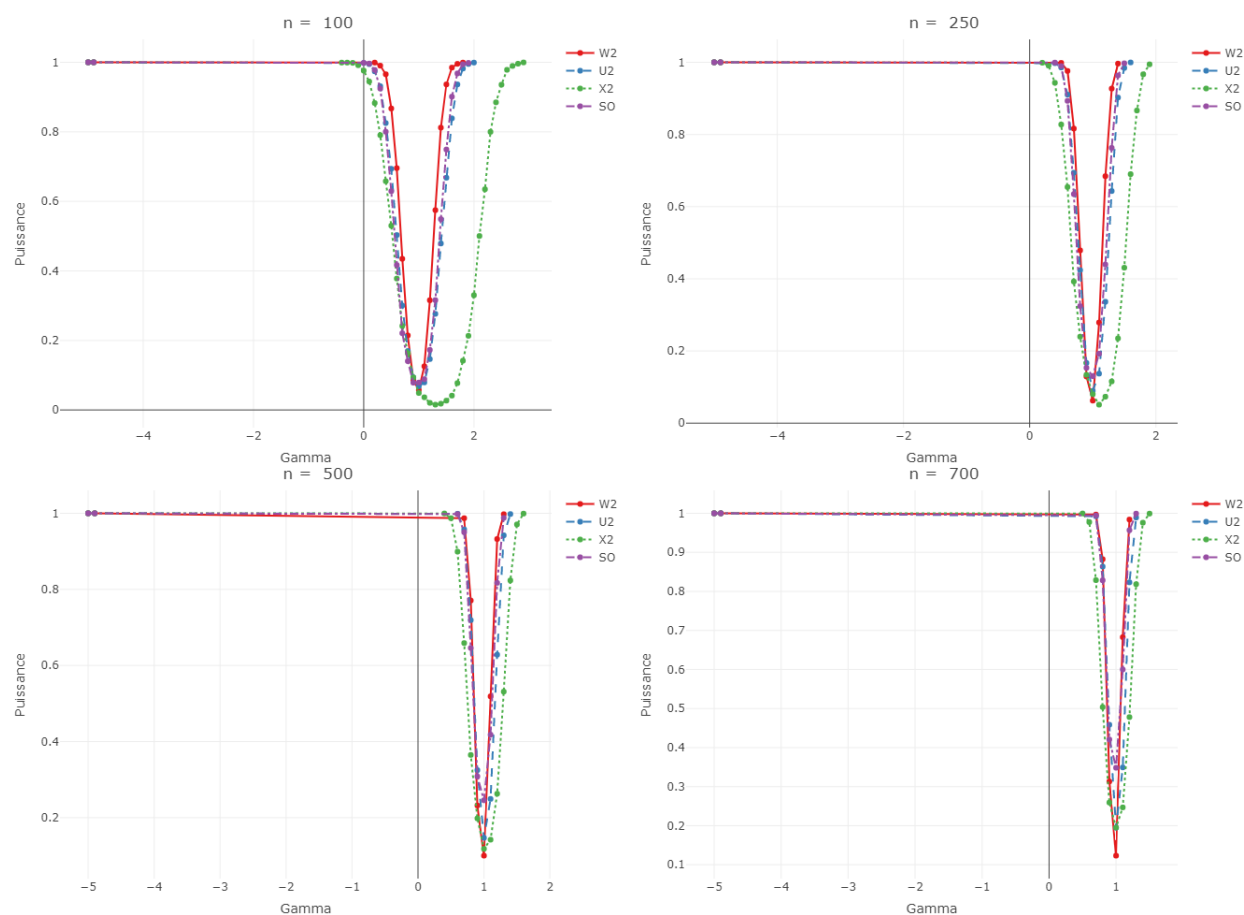
FIGURE 3.3.61 – Newcomb-Benford Généralisée sachant Newcomb-Benford Généralisée (\mathcal{GB}_1(\gamma), \mathcal{GB}_{(2|1)}(\gamma)) : Courbes de puissance, en fonction du paramètre \gamma , de divers tests (basés sur 10000 répliquations) au niveau 5% pour l'hypothèse nulle de la loi Newcomb-Benford \mathcal{B}_{(1,2)} . Les tests représentés sont : W^2 (couleur rouge), \chi^2 (couleur verte), U^2 (couleur bleue) et STO (couleur violette) dont les expressions se trouvent respectivement aux Sections 3.3.3 et 3.3.18. Les quantiles de référence sont approximés par Monte-Carlo en utilisant 1000000 répétitions.
