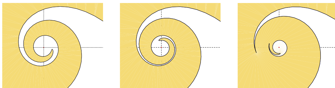
FIGURE 4.12 – Trois boules avec un zoom autour du vortex (point rouge) aux temps t \in \{2.86, 2.88, 2.9\} . Comparez avec la Figure 4.11. Pour t = 2,9 la boule \mathbb{B}(x_0, t) est de type B et possède un petit trou en forme de fœtus.
