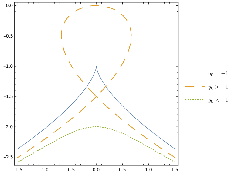
FIGURE 2.7 – Exemple historique de Carathéodory-Zermelo, "Plus rapide chemin nautique", comme un déploiement de la singularité générique du cusp le long de géodésiques anormales.
