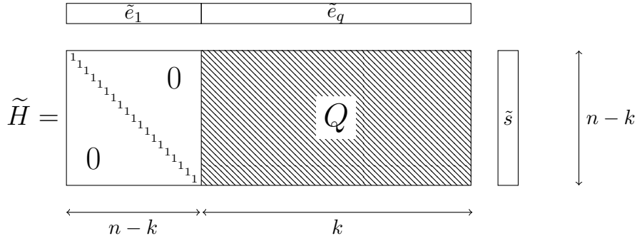
FIGURE 4.7 – Un cadre algorithmique pour l' Information Set Decoding .
