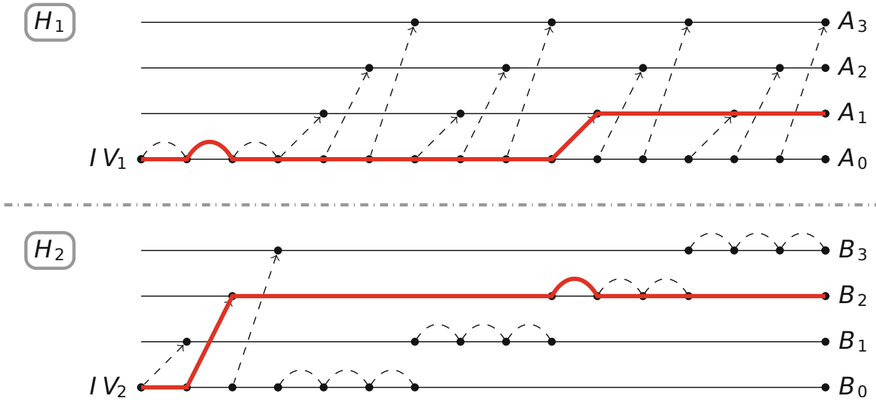
FIGURE 5.8 – « Interchange Structure » utilisée dans l’attaque de Leurent et Wang [150]. Avec N^2 collisions, on peut atteindre chacune des N^2 paires d’états internes (A_i, B_j) avec H_1 et H_2 . Image : [150].
