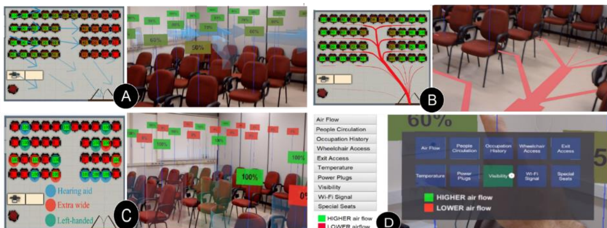
Figure 2.8 – Les différentes visualisations de données situées pour faciliter l'accès à un siège dans une pièce (Guarese et al., 2020)
