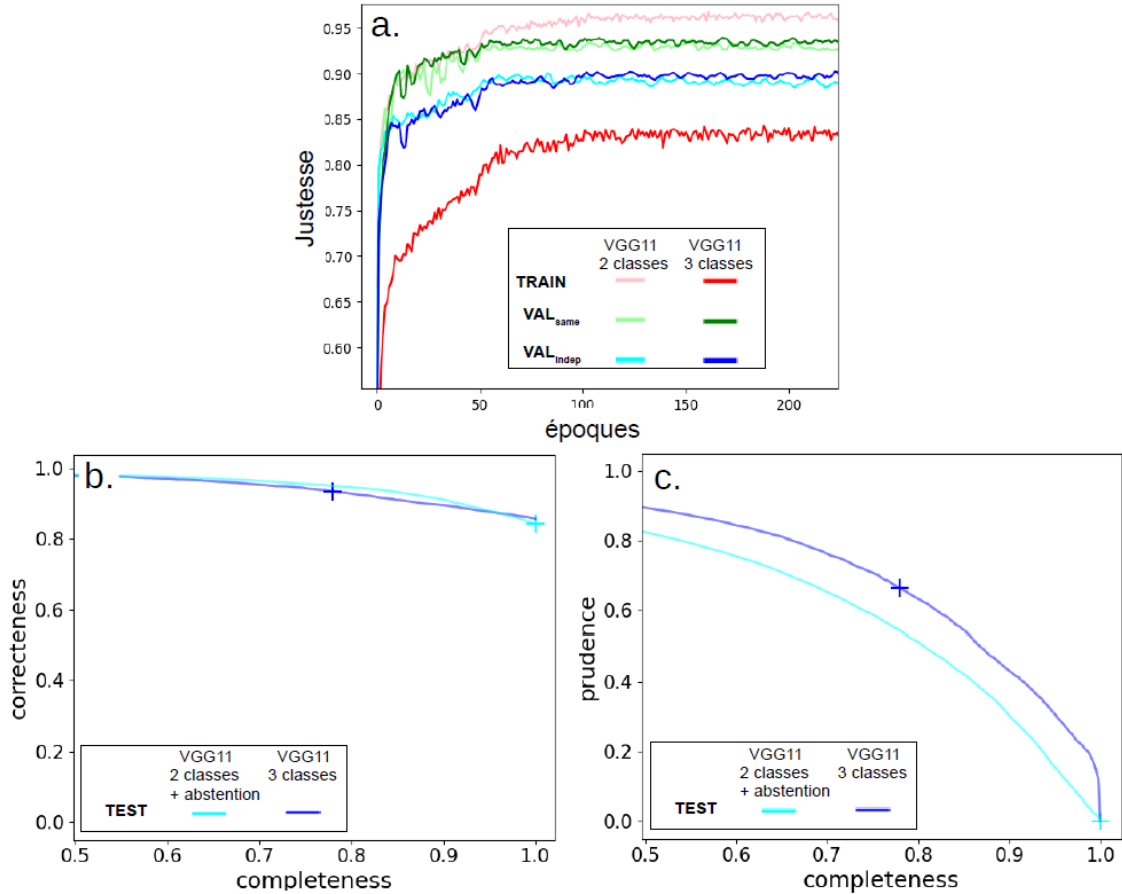
FIGURE 3.6 – Comparaison entre deux classifieurs VGG11 entraînés à la prédiction par paire. Le premier est entraîné sur \mathcal{G}_0^v à classer les paires d’images parmi \{\succ, \prec\} . Le second est entraîné sur \mathcal{G}_0^v et \mathcal{U}_0^v à classer parmi \{\succ, \prec, \perp\} . En a., on a désactivé la prédiction d’incomparabilité pour comparer les justesses sur VAL_{same} et VAL_{indep} . En c. et d., on compare sur le jeu de test les classifieurs après épaississement (voir encadré 3.1). Les courbes sont obtenues en faisant varier le paramètre \lambda .
