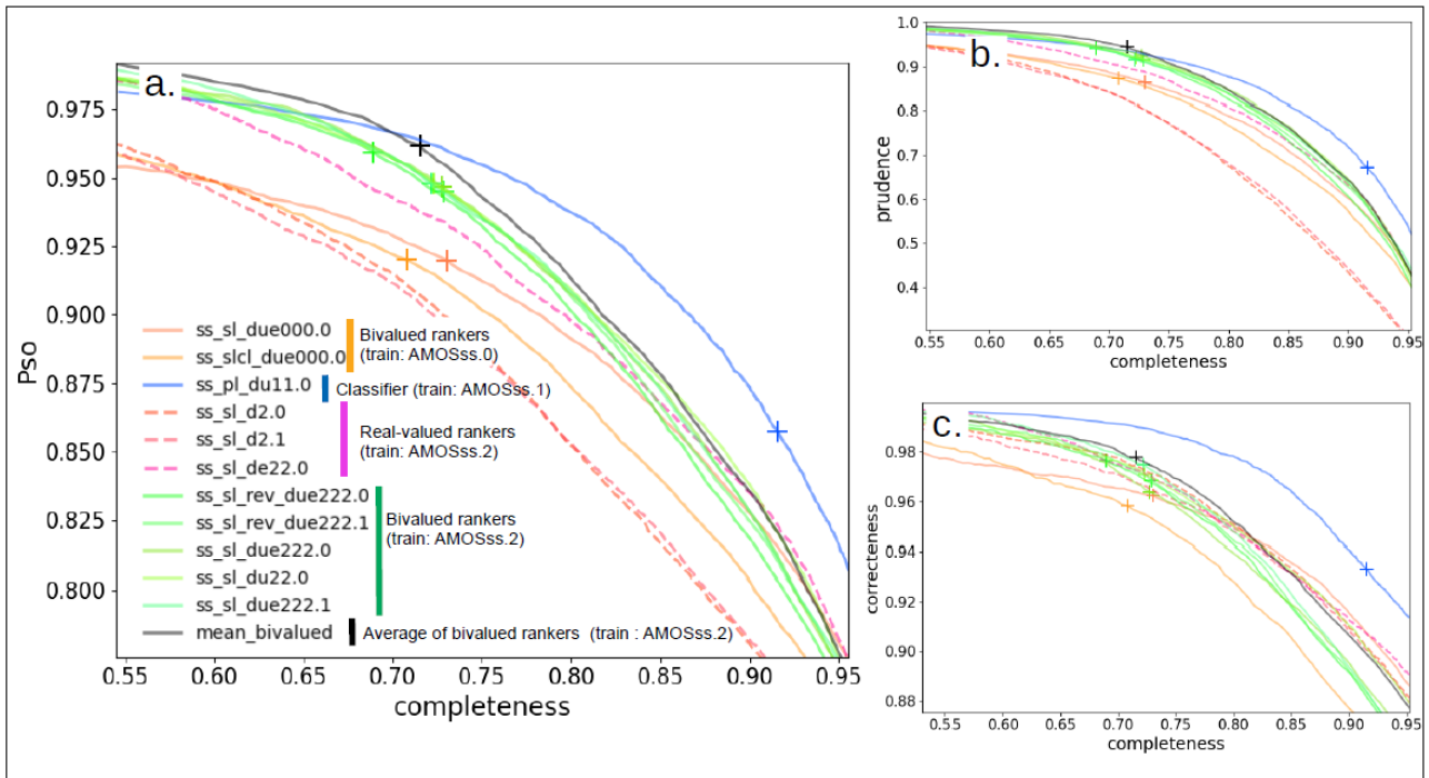
FIGURE 5.5 – Performances des fonctions de rang semi-supervisées pour l'estimation relative de l'étendue. Les P_{so} , prudence, completeness et correctness ont été calculées sur les paires du jeu de test d'AMOSss.1. La courbe bleue marque les performances du classifieur utilisé pour construire le jeu AMOSssExt. Les courbes vertes représentent les fonctions de rang bivaluées apprises sur AMOSssExt. Le moyennage de ces cinq fonctions donne la courbe noire. Les courbes pointillées correspondent à des fonctions de rang à valeurs réelles apprises sur AMOSssExt tandis que les courbes oranges continues représentent les meilleures fonctions de rang bivaluées apprises sur AMOSss.0.
