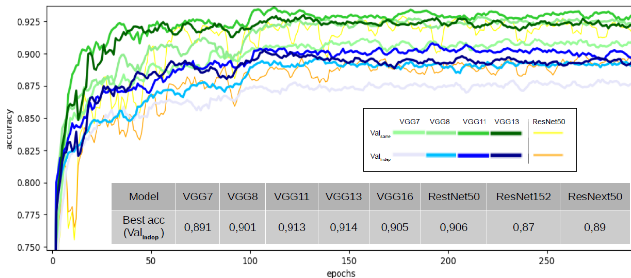
FIGURE A-1 – Apprentissage des préférences sur AMOSv. Performances en validation de la prédiction par paire. Les modèles VGG7 et VGG8 contiennent respectivement 4 et 5 couches de convolution. Les courbes ont été lissées par moyenne mobile (largeur : 5 époques).
