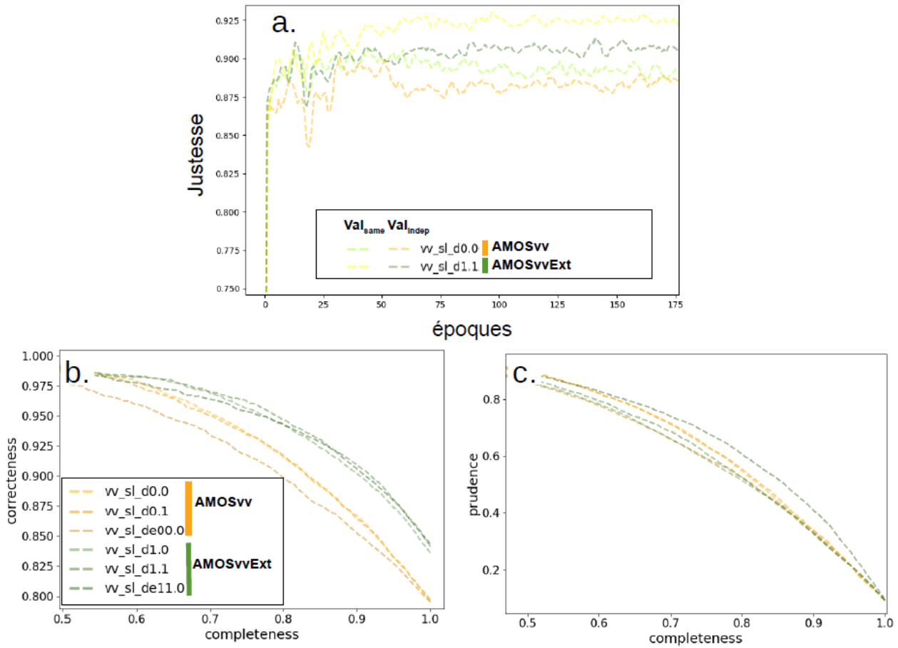
FIGURE 4.1 – Comparaison entre des fonctions de rang implémentées sur des ResNet50 et apprises soit sur AMOSvv (méthode supervisée) soit sur AMOSvvExt (méthode semi-supervisée). a. Courbes d'apprentissage représentatives pour chacune des deux méthodes. b. Comparaison sur le jeu de test à partir des métriques définies en section 3.2.1.2. Pour chaque méthode, deux fonctions de rang ont été apprises sur les paires strictement ordonnées. L'apprentissage de la troisième fonction de rang fait intervenir les équivalences (voir l'annexe C).
