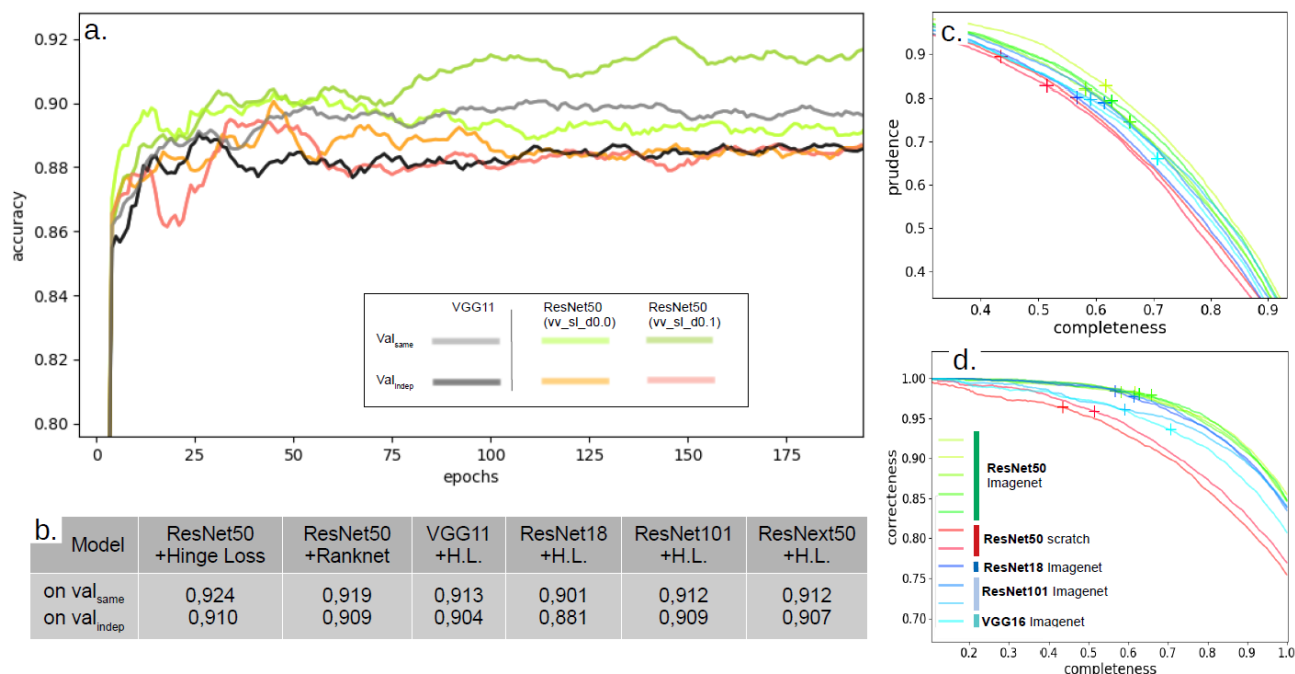
FIGURE A-2 – Apprentissage des préférences sur MAMOSv. Performances en validation de la prédiction par image. a. Courbes d'apprentissage (après lissage) sur AMOSv. b.meilleures performances sur le jeu de validation. c-d. Séparation des différentes architectures sur le jeu de test, après apprentissage sur AMOSvExt.
