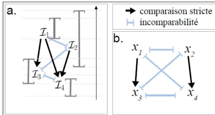
FIGURE 4.2 – a. L'ordre partiel défini sur l'ensemble des \mathcal{I}_k est un ordre d'intervalles. L'incomparabilité correspond au chevauchement. b. Les éléments x_1; x_2; x_3; x_4 ne peuvent pas être représentés sous la forme d'intervalles. C'est un ensemble ordonné de type “2+2”.
