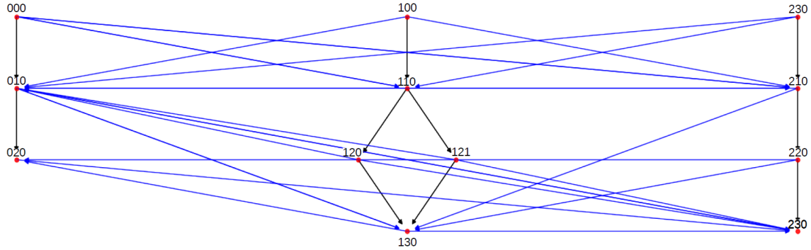
FIGURE 2.13 – Relation d’ordre partiel entre douze images (nœuds du graphe) triées suivant le critère de la visibilité. Les nombres associés aux images sont composés de trois numéros : le premier indique l’indice de la chaîne dans la décomposition, le second indique la situe dans la chaîne, le dernier la situe dans la classe d’équivalence de l’image (seule une classe comporte deux images : 120,121). Les arêtes noires figurent la décomposition en chaînes obtenue par poset-mergesort .
