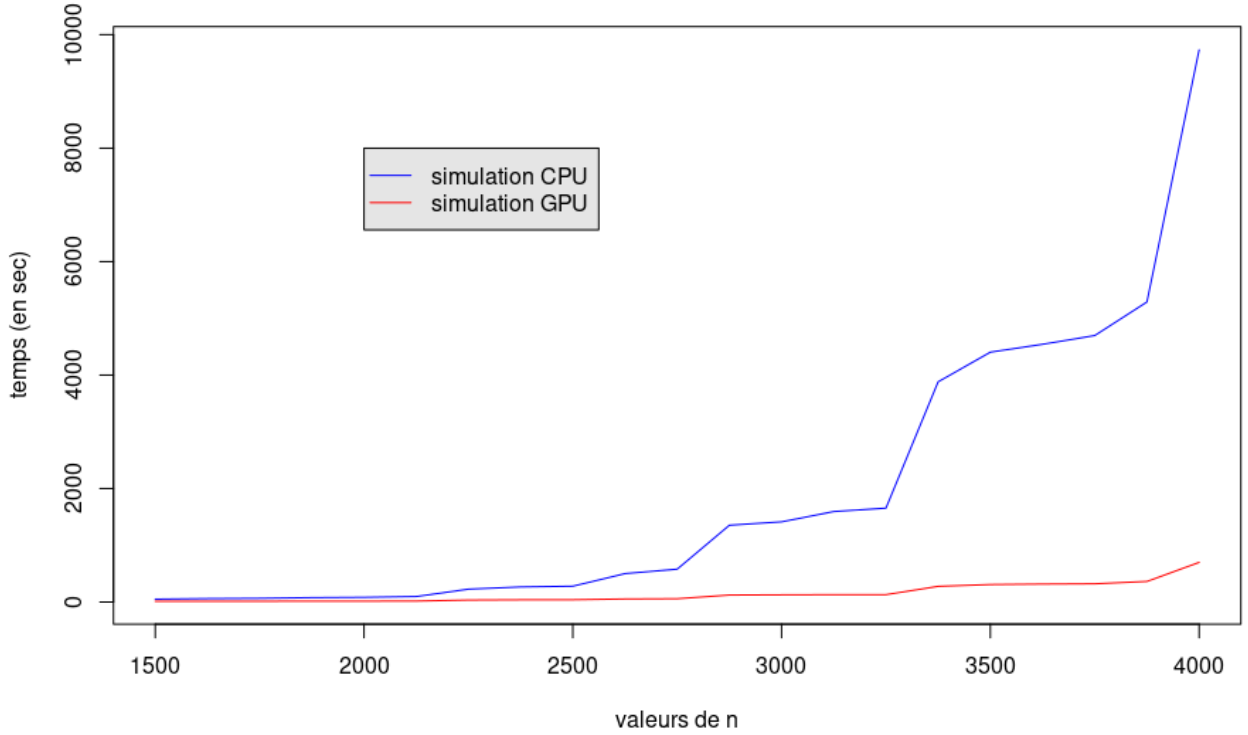
FIGURE 4.6 – Évolution du temps de simulation d’une réalisation de la \tau -cohérence en fonction des valeurs de n pour la méthode de simulation CPU et GPU
