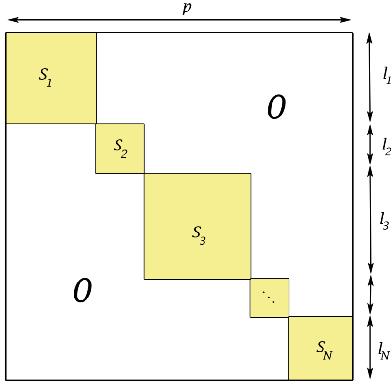
FIGURE 3.1 – Structure de la matrice \Sigma de covariance par blocs.
