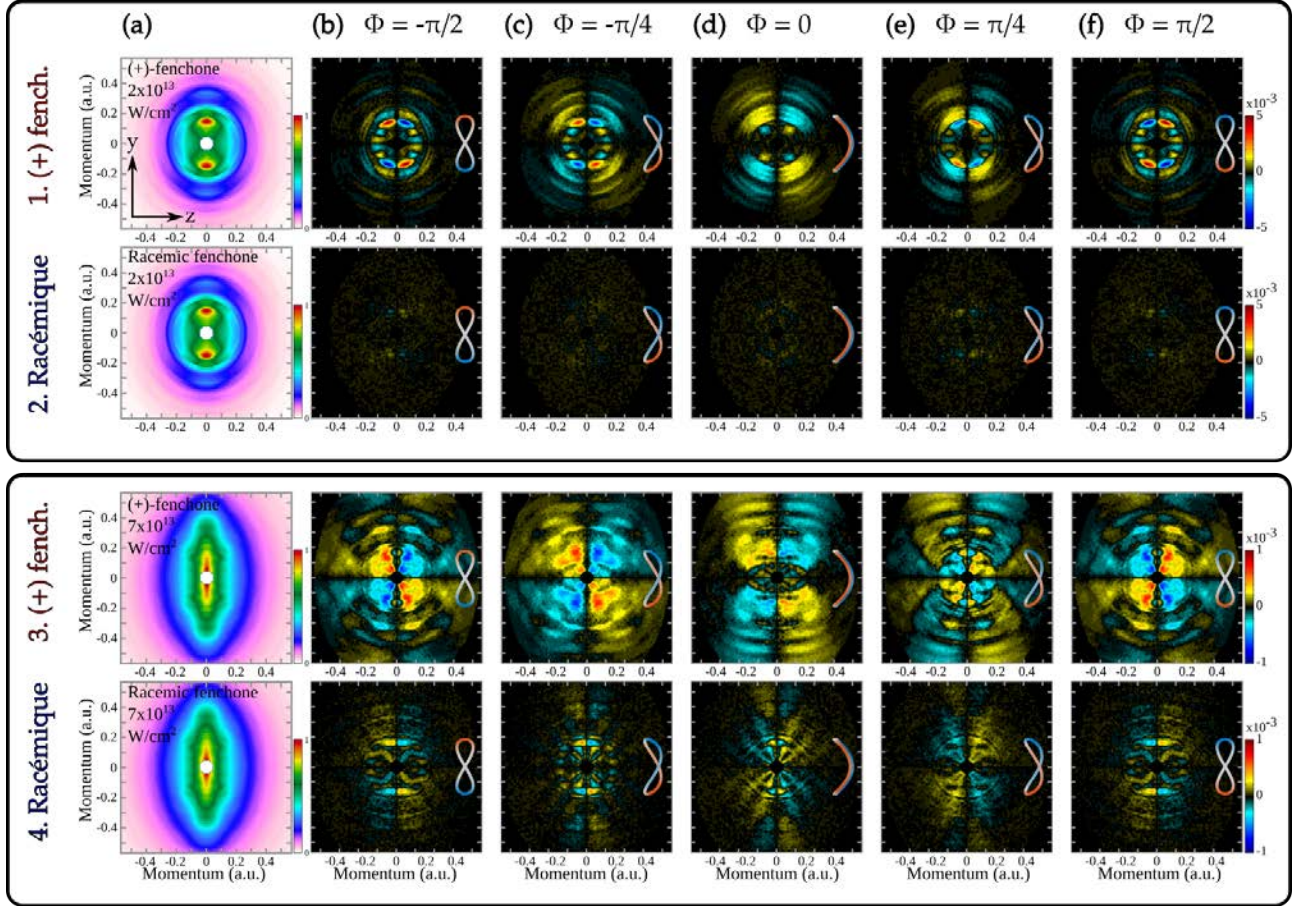
FIGURE 4.9 – Résultats expérimentaux. La première colonne (a) représente la projection normalisée de la distribution angulaire de photoélectrons dans le plan (y,z) du détecteur. Les colonnes (b) à (f) représentent le signal asymétrique ESCARGOT pour les phases relatives \phi = -\pi/2, -\pi/4, 0, \pi/4, \pi/2 respectivement. Pour chaque phase relative, le profil du champ OTC est indiqué dans le plan de polarisation (y,x) . Les deux premières lignes sont mesurées à 2 \times 10^{13} \text{ W/cm}^2 dans la (+)-fenchone (1) et dans un mélange racémique. Idem pour les lignes 3 et 4 à I = 7 \times 10^{13} \text{ W/cm}^2 . Chaque image d’asymétrie est antisymétrisée haut/bas pour compenser d’éventuels défauts de détecteur ou d’imagerie.
