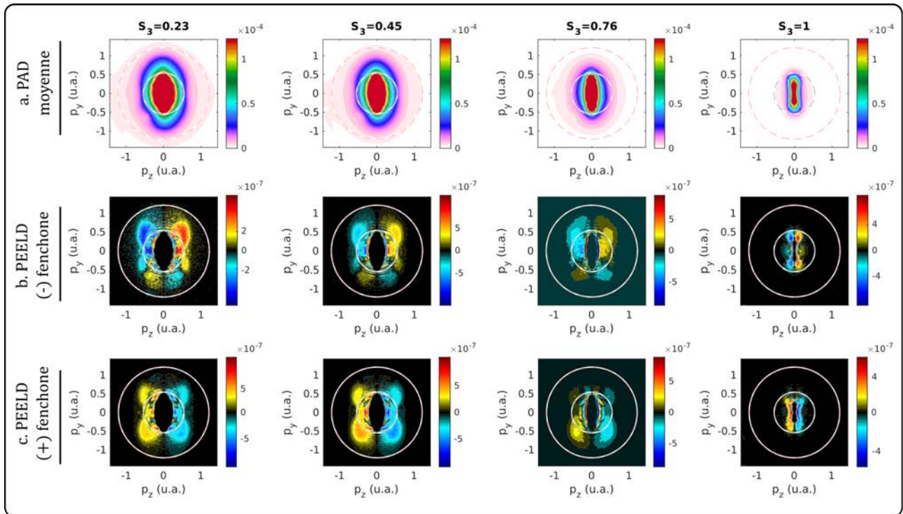
FIGURE 3.13 – PAD (a) et PEELD brutes (b-c) dans la fenêtrone à 1030 nm pour I = 2.34 \times 10^{13} W/cm 2 et pour différentes valeurs de S_3 ( \gamma = 1.35 et U_p = 2.32 eV).
