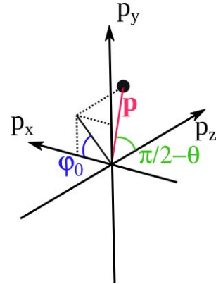
– Repère utilisé et définitions des angles \varphi_0 et \theta pour un électron d'impulsion finale p .
