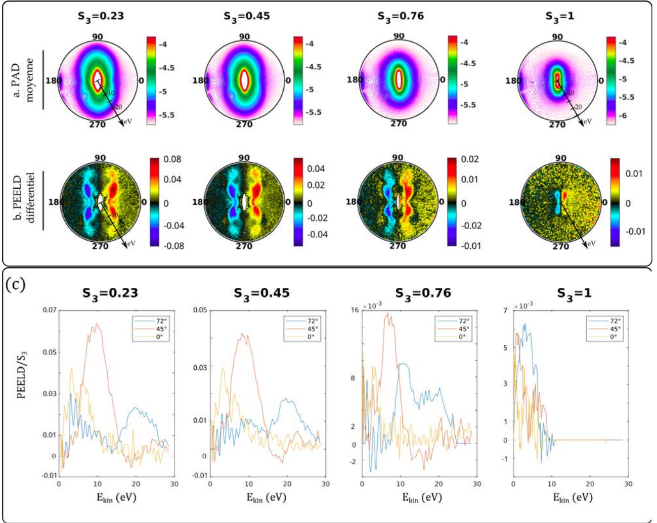
FIGURE 3.15 – Représentation en énergie pour différentes valeurs de S_3 avec I = 2.34 \times 10^{13} \text{ W/cm}^2 ( \gamma = 1.35 et U_p = 2.32 \text{ eV} ). (a) La PAD est obtenue par la moyenne des PAD entre les deux énantiomères et est représentée ici en échelle logarithmique. (b) PEELD différentiel de la fençhone à 1030 nm, normalisé par S_3 . (c) Coupes/profils angulaires du PEELD de la fençhone où le PEELD est maximal.
