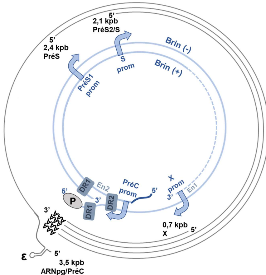
Figure 6 : Organisation génétique du HBV , d'après (McNaughton et al. , 2019). Le génome du HBV, représenté en bleu, est une structure circulaire partiellement double brin de 3,2 kb appelée ADN-rc. Le brin négatif (-) est lié à la polymérase virale P en 5'. Le brin (+) varie en taille et possède une séquence amorce d'ARN de 19 nucléotides représentée en bleu foncé. L'expression du génome est induite par quatre promoteurs nommés PrèC prom, PrèS1 prom, S prom, et X prom. Les séquences redondantes DR1/DR2 jouent un rôle dans la synthèse du génome viral lors de la répllication. En gris sont représentés les quatre ARN viraux synthétisés à partir du génome. L'ARNpg/prèC possède une boucle \epsilon en 5' impliquée dans l'encapsidation du génome lors de la répllication.
