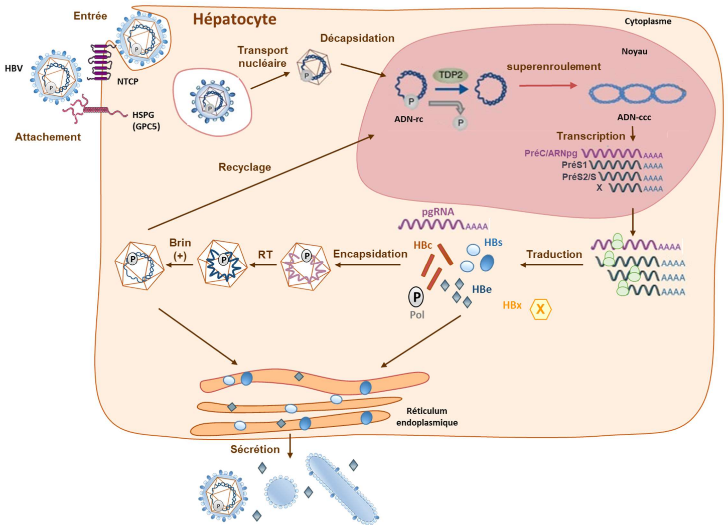
Figure 10 : Représentation schématique du cycle viral du HBV d'après (Baumert et al., 2015). L'attachement de la particule virale à GPC5 et la liaison au récepteur NTCP induit l'endocytose du HBV. La nucléocapside est transportée dans le noyau à travers des pores nucléaires. L'ADN-rc est converti en ADNccc par un processus multi-étape. Les ARN viraux sont transcrits à partir de l'ADNccc et exportés dans le cytoplasme. L'ARNpg est empaqueté dans une néo-nucléocapside avec la polymérase virale où il est rétrotranscrit en ADN. Les nucléocapsides virales matures peuvent être recyclées dans le noyau ou sécrétées, après acquisition de son enveloppe, dans le milieu extracellulaire.
