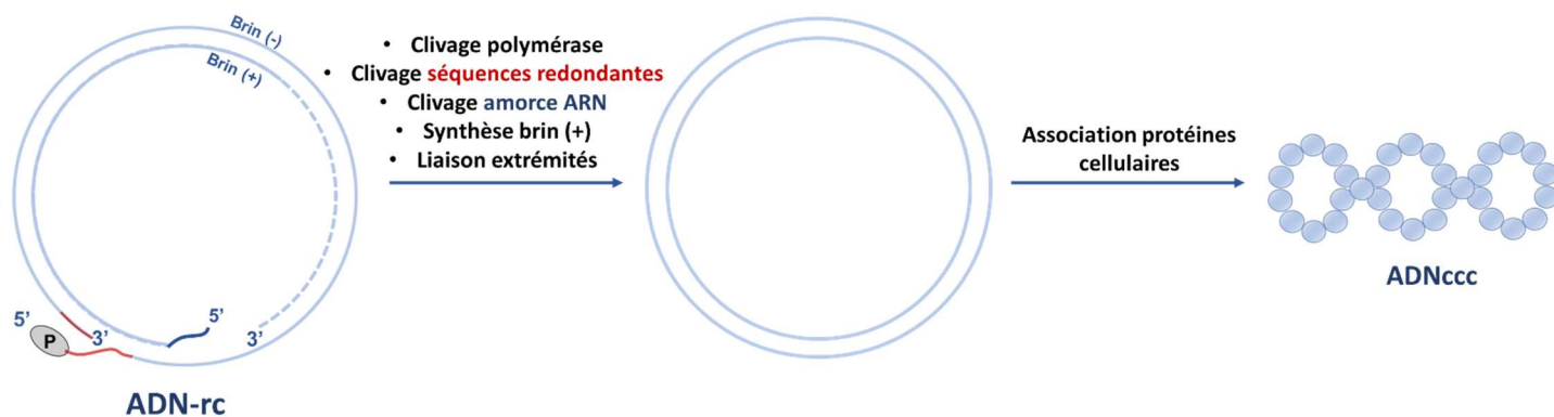
Figure 7 : Représentation schématique de la conversion de l'ADN-rc en ADNccc , d'après (Lucifora et al. , 2016). La formation de l'ADNccc à partir de l'ADN-rc nécessite le clivage de la polymérase en 5' du brin (-), de l'amorce ARN en 5' du brin (+) et des séquences redondantes DR1/2. La liaison des extrémités implique des mécanismes de réparation de l'ADN, de modifications de structure, de synthèse et de liaison. Le surenroulement d'ADN viral implique des protéines cellulaires telles que les histones.
