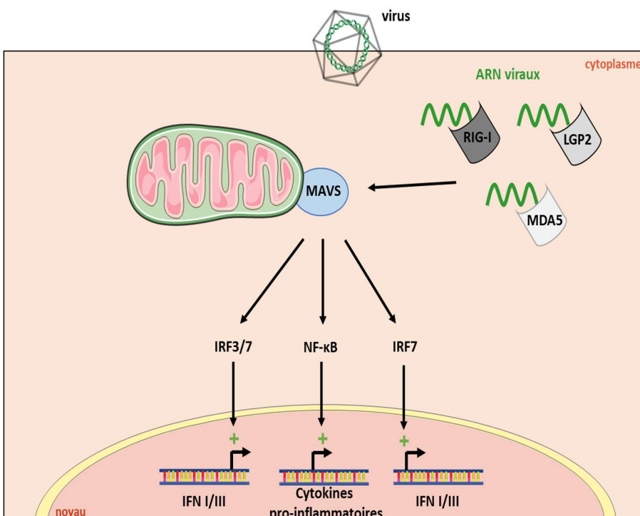
Figure 12 : Représentation schématique des voies d'induction de l'IFN par les hélicases cytosoliques.
