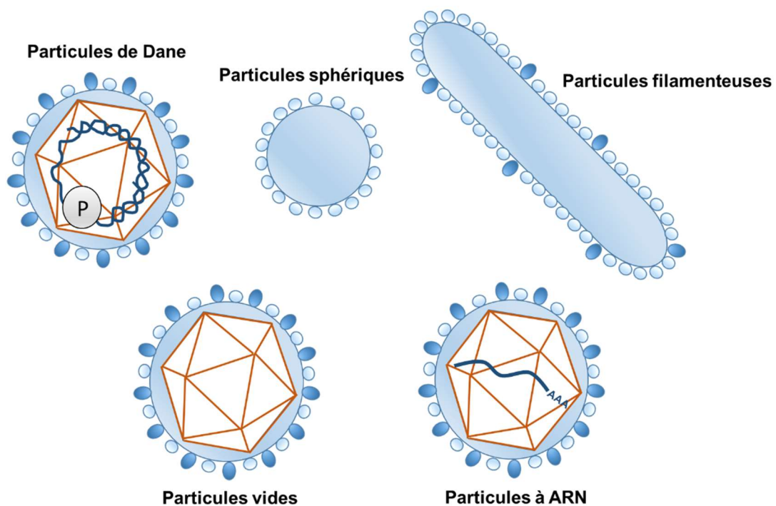
Figure 5 : Représentation schématique des formes infectieuses et non infectieuses du HBV. Les particules infectieuses, aussi appelées particules de Dane, sont enveloppées d'une bicouche lipidique portant les glycoprotéines virales de surface, qui entourent une nucléocapside contenant le génome viral. Les particules non infectieuses correspondent aux particules subvirales sphériques et filamenteuses, aux particules vides et aux particules contenant de l'ARN viral.
