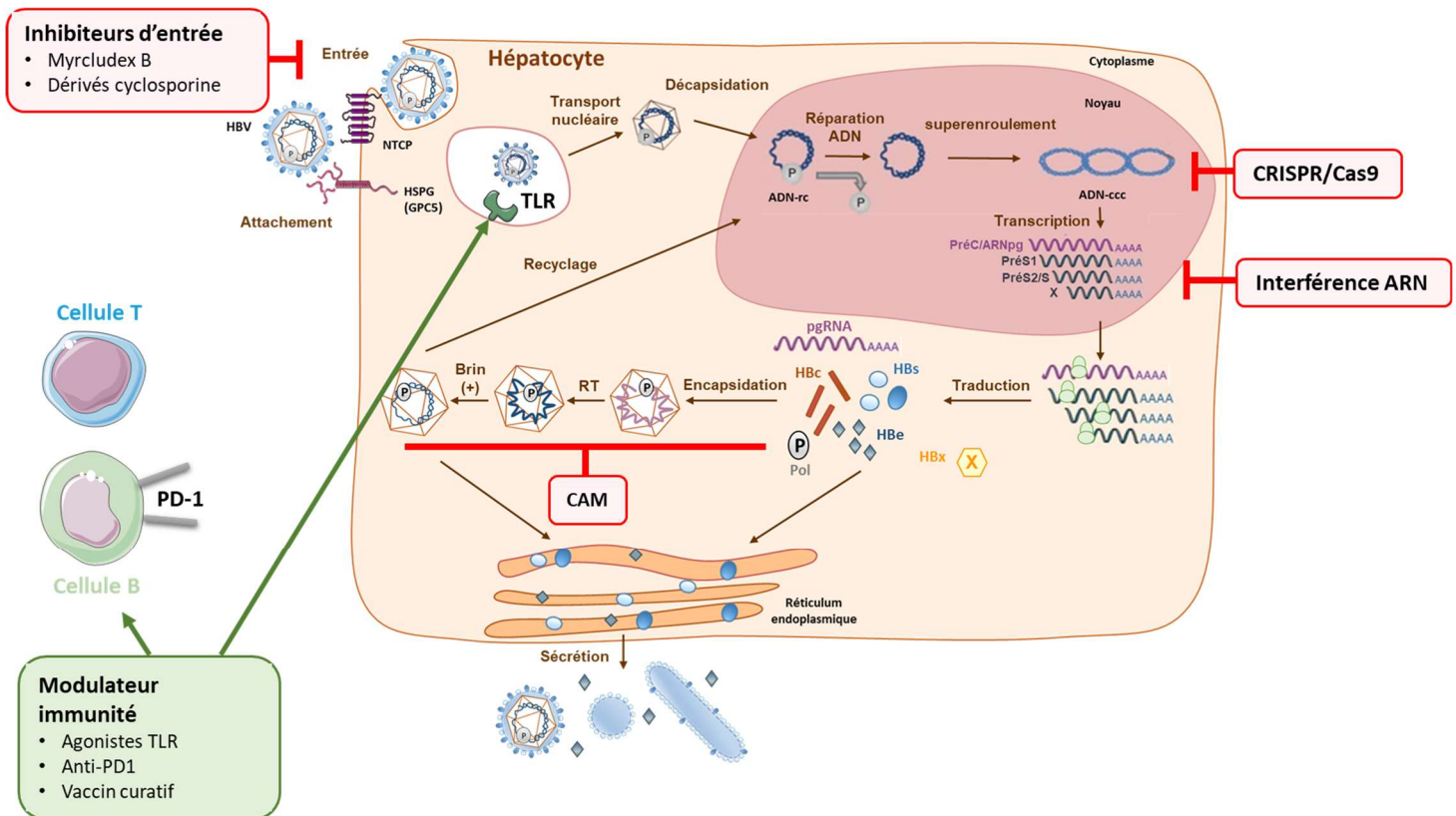
Figure 14 : Schéma des nouvelles stratégies thérapeutiques contre le HBV , d'après (Zoulim et al. , 2016). De nouvelles molécules antivirales sont en cours de développement. Certaines ciblent le virus avec des outils moléculaires de modulation de l'expression des gènes viraux (interférence ARN, CRISPR/Cas9) ou des modulateurs de l'assemblage de la capsid (CAM). D'autres ciblent l'hôte avec des inhibiteurs d'entrée (Myrcludex B/Bulevirdite, dérivés de cyclosporine) ou modulent la réponse immunitaire anti-HBV innée ou adaptative avec les agonistes de TLR, les anticorps anti-PD1 ou le vaccin curatif.
