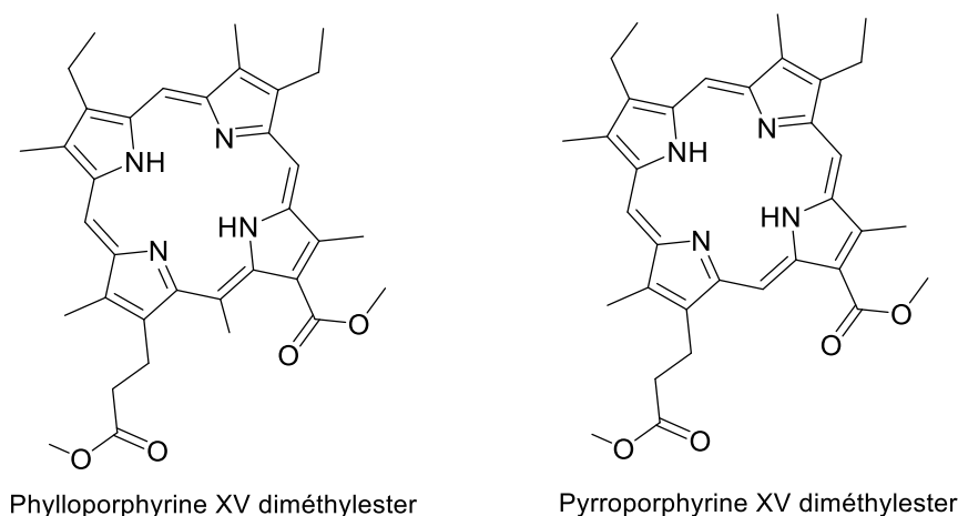
Figure 42 : Porphyrines issus de la chlorophylle a.
