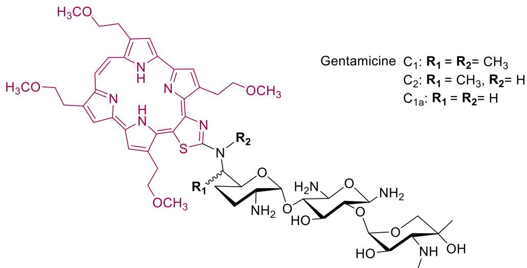
Figure 62 : Structure du conjugué gentamicine - porphycène synthétisé par Nonell et coll. [219].
