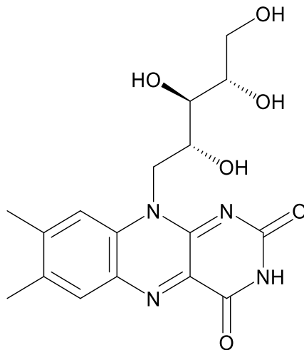
Figure 25 : Structure de la riboflavine
