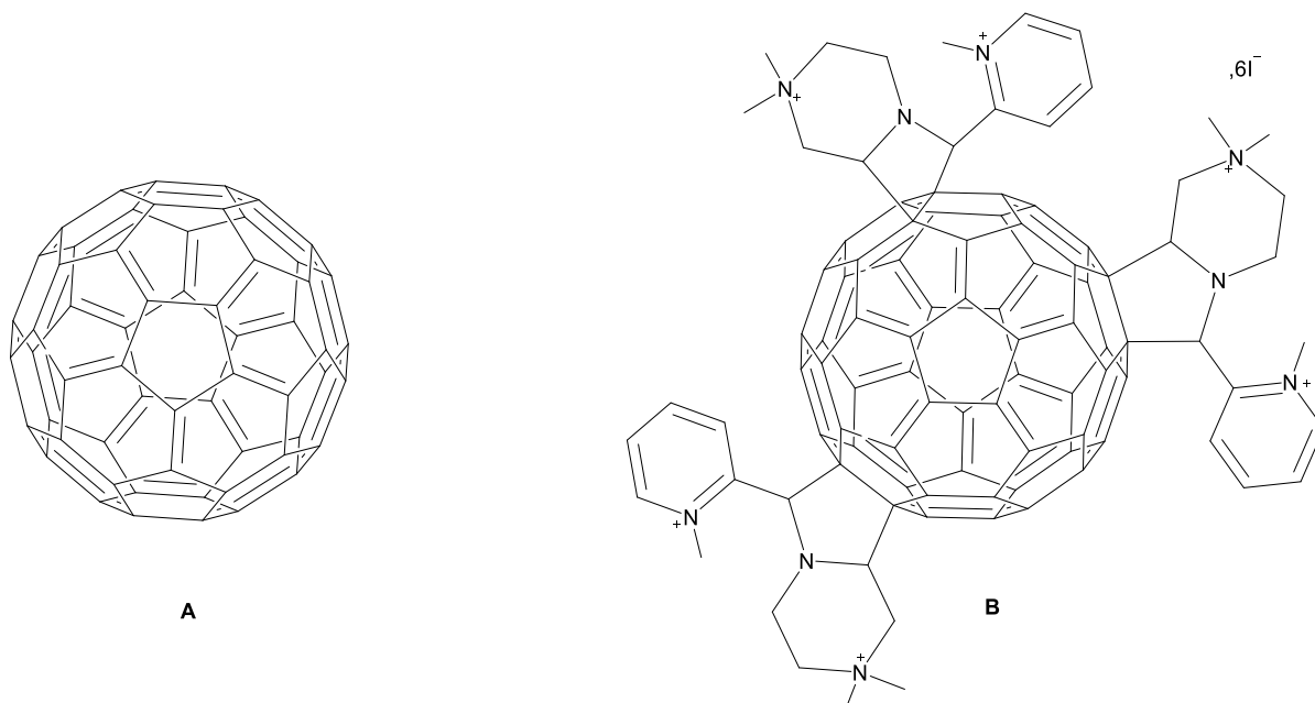
Figure 32 : A : Structure du Buckminsterfullerène (C 60 ), B : Dérivé de fullerène utilisé comme PS antimicrobien.
