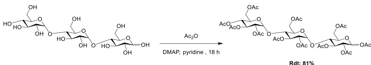
Figure 79 : La peracétylation du maltotriose
