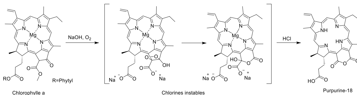
Figure 41 : Synthèse de la purpurine-18 à partir de la chlorophylle a.
