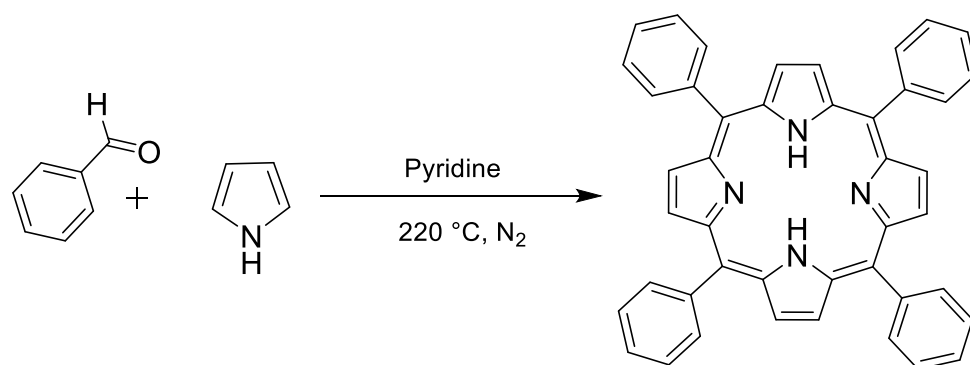
Figure 43 : Synthèse de la TPP selon Rothemund.
