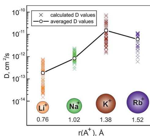
Figure 12. Coefficient de diffusion ionique dans la structure \text{MVPO}_4\text{F} ( \text{M}=\text{Li}, \text{Na} ou \text{K} ). Extrait de la référence [61].
