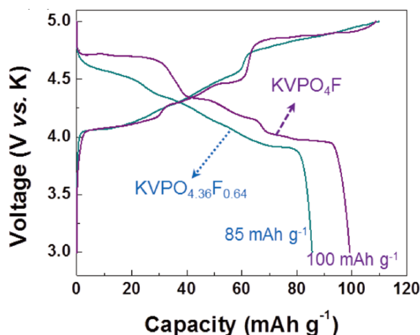
Figure 11. Courbes galvanostatiques des matériaux \text{KVPO}_4\text{F} et \text{KVPO}_{4.36}\text{F}_{0.64}\text{O}_{0.36} . Extrait de la référence [60].
