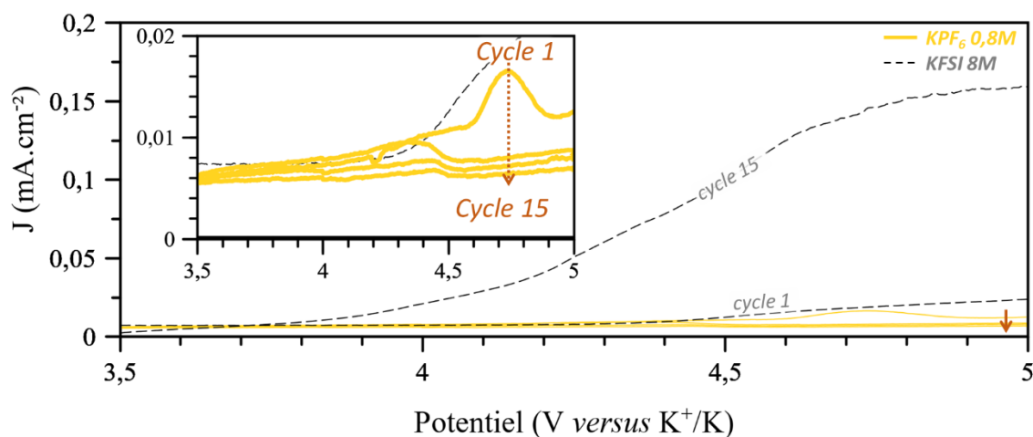
Figure 5. Voltamogrammes du 1 er , 5 e , 10 e et 15 e cycles d'une électrode d'aluminium dans \text{KPF}_6 -EC:DEC à une concentration de 0,8M, et voltamogrammes du 1 er et 15 e cycles d'une électrode d'aluminium dans KFSI-EC:DEC à une concentration de 8M.
