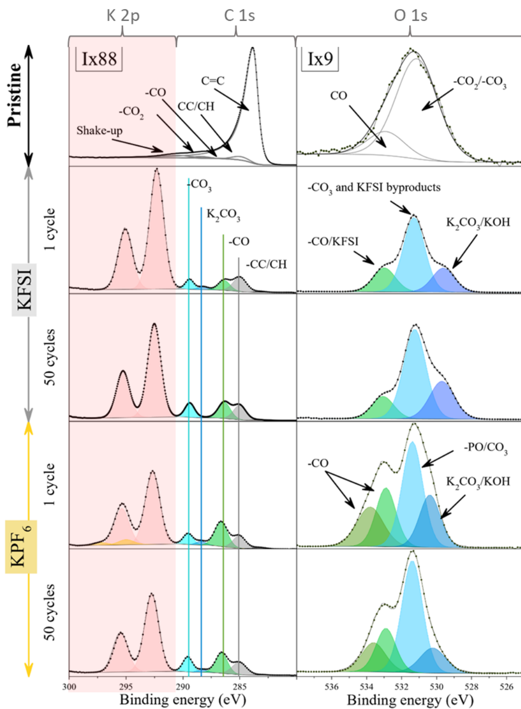
Figure 7. Spectres XPS C 1s, K 2p et O 1s des électrodes de fibres de carbone après 1 cycle et après 50 cycles, pour des électrolytes à base de KPF 6 ou de KFSI- 0,8M EC:DEC. Adapté de la référence [12], annexe II.
