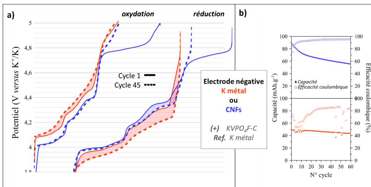
Figure 3. Comparaison pour une configuration 3 électrodes, en fonction de l'électrode négative utilisée, des a) Courbes galvanostatiques de \text{KVPO}_4\text{F-C} normalisées (axe des abscisses) du 1 er et 45 e cycles (polarisation surlignée). b) capacités en décharge et efficacités coulombiques.
