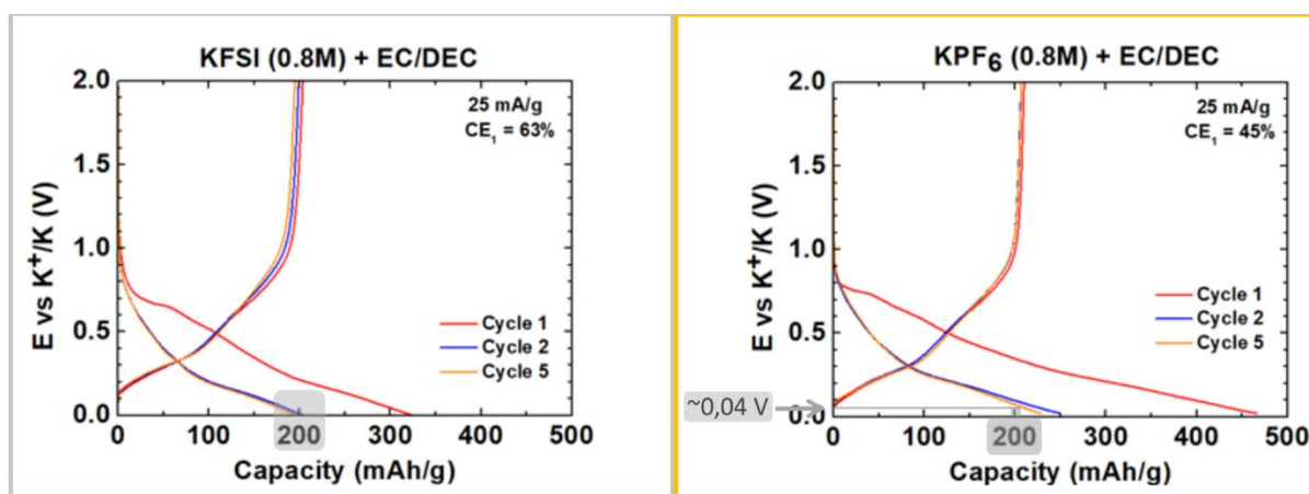
Figure 5. Courbes galvanostatiques des électrodes CNFs en fonction de l'électrolyte. Adapté de la référence [12], annexe II.
