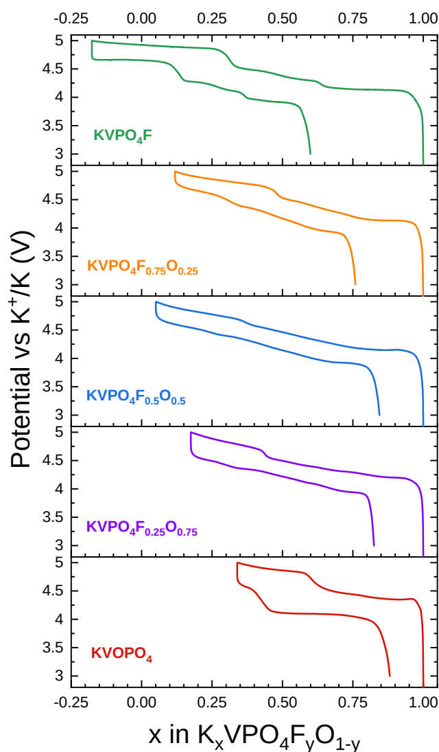
Figure 7. Courbes galvanostatiques du 1 er cycle des électrodes de \text{KVPO}_4\text{F}_x\text{O}_{1-x} (figure telle que transmise par l'ICMCB).
