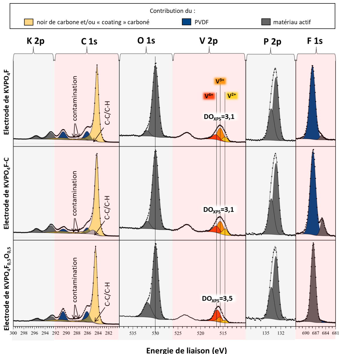
Figure 14. Spectres XPS K 2p-C 1s, F 1s, P 2p et O 1s – V 2p des électrodes KVPO 4 F et KVPO 4 F-C. Tous les spectres ont été calibrés sur le carbone à 285,0 eV, à l'exception de O 1s et V 2p qui sont calibrés sur la composante majoritaire de l'oxygène à 530,0 eV.
