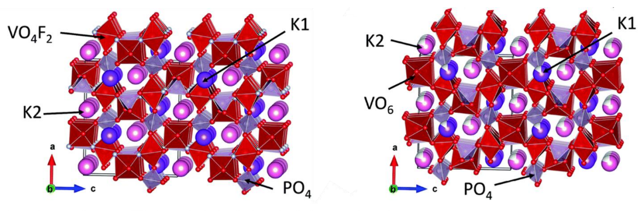
Figure 10. Structures des matériaux \text{KVPO}_4\text{F} (gauche) et \text{KVOPO}_4 (droite). Extrait de la référence [59].
