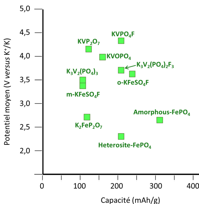
Figure 9. Aperçu des composés polyanioniques utilisés dans les KIBs. Adapté de la référence [25].
