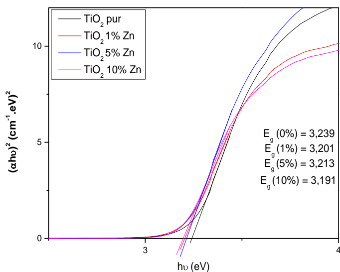
Fig.V.21 Energie de la bande interdite obtenue en extrapolant la partie linéaire de la courbe (\alpha hv)^2 en fonction de l'énergie des photons (eV) des nanoparticules de TiO_2 pur et de TiO_2 dopé au Zn
