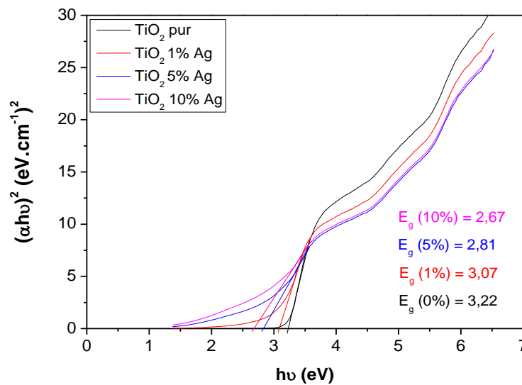
Fig.V.10 Bande interdite obtenue en extrapolant la partie linéaire de la courbe (\alpha h\nu)^2 en fonction de l'énergie des photons (eV) des nanoparticules de \text{TiO}_2 et de \text{TiO}_2 dopé à l'Ag
