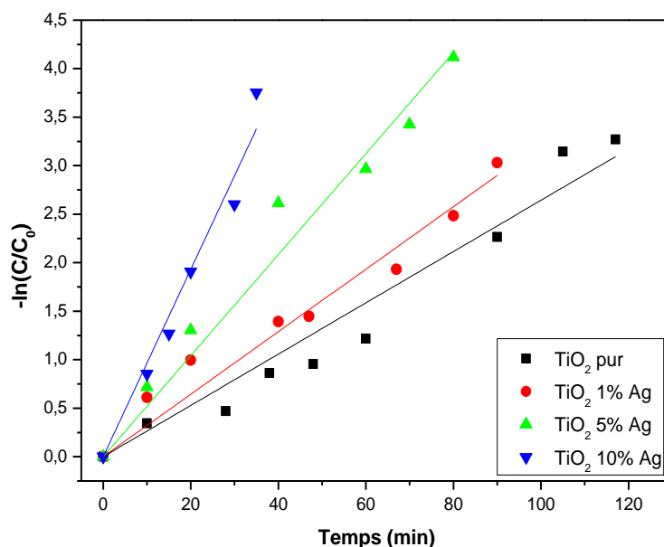
Fig.V.26 Cinétique de pseudo-premier ordre pour la dégradation photo-catalytique du BM par TiO 2 dopé Ag
