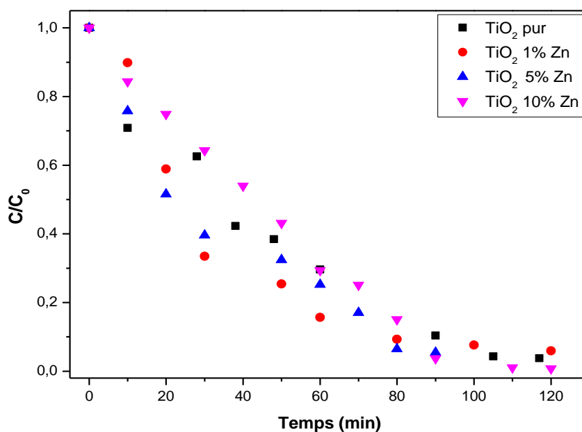
Fig.V.27 Dégradation photo-catalytique du bleu de méthylène (BM) sous irradiation UV en présence des nanopoudres de TiO 2 pur et dopé au zinc
