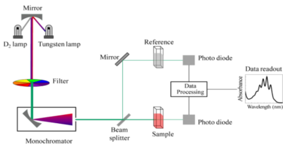
Fig.III.10 Représentation schématique du spectrophotomètre UV-Visible à double faisceau [2]
