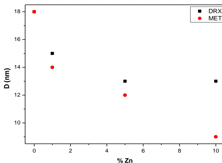
Fig.V.19 Evolution de la taille des grains en fonction de la concentration en Zn par DRX et par MET
