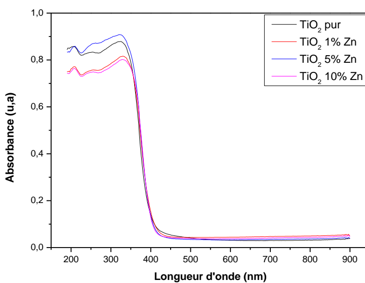
Fig.V.20 Spectres d'absorbance des nanopoudres de \text{TiO}_2 pur et dopé au Zn
