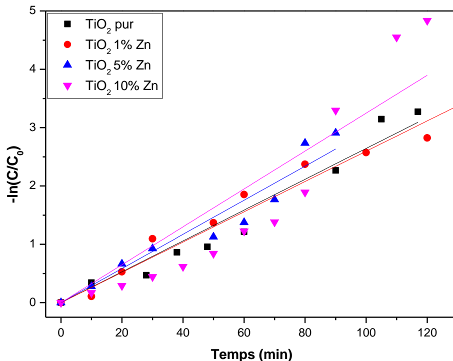
Fig.V.28 Cinétique de pseudo-premier ordre pour la dégradation photo-catalytique du BM par \text{TiO}_2 dopé Zn
