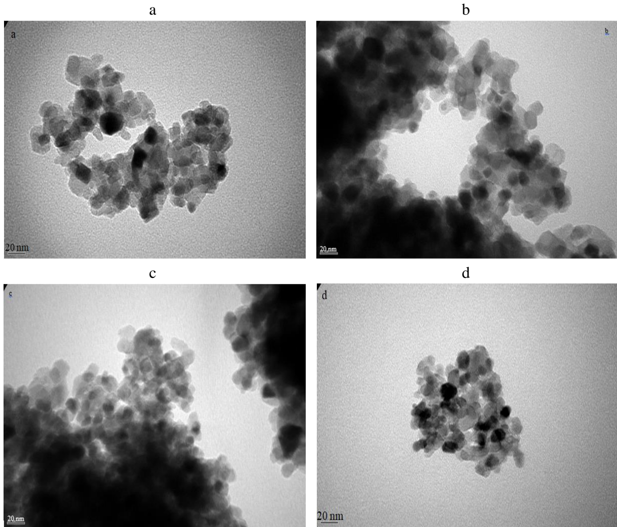
Fig.V.17 Images obtenues par MET des nanopoudres de : (a) \text{TiO}_2 pur et dopé : (b) : 1% Zn, (c) : 5% Zn et (d) : 10% Zn
