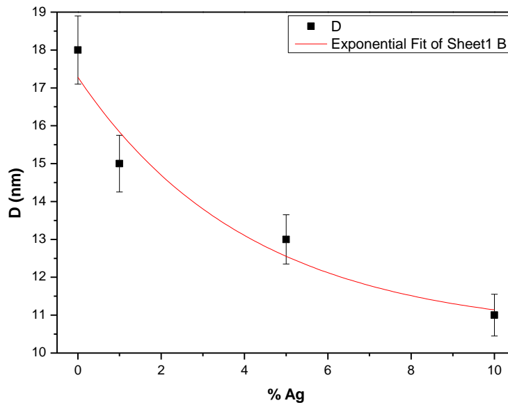
Fig.V.7 Evolution de la taille des grains calculée par MET en fonction de la concentration en Ag
