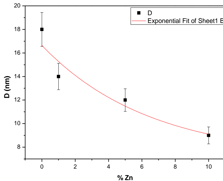
Fig.V.18 Evolution de la taille des grains calculée par MET en fonction de la concentration en Zn
