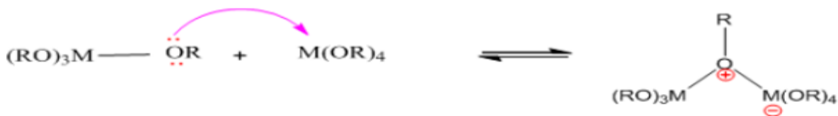
Fig.II.5 Mécanisme d'alcoolation des alcoxydes métalliques \text{M}(\text{OR})_n [4]
