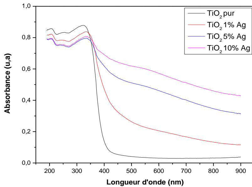
Fig.V.9 Spectres d'absorbance des nanopoudres de TiO 2 pur et dopé à l'Ag
