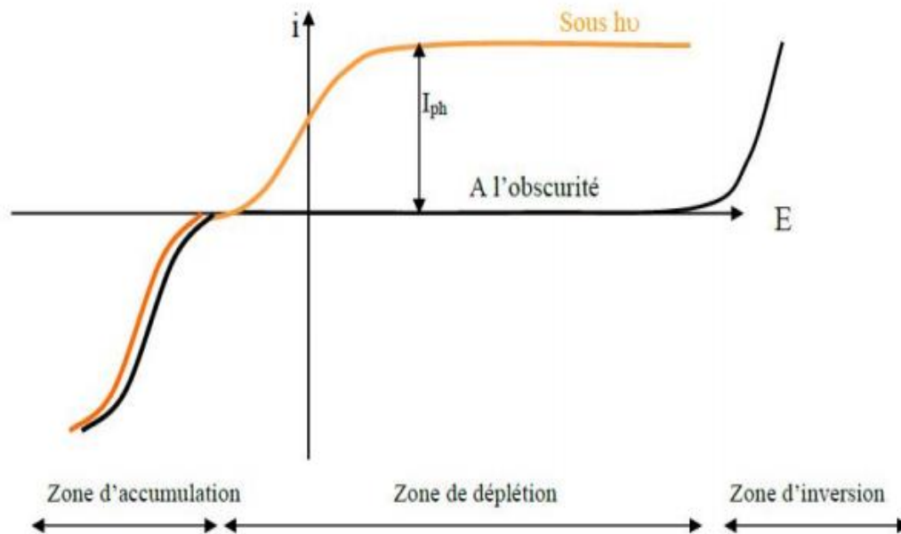
Fig.I.13 Courbe I = f(E) à l'obscurité et sous éclaircissement pour un SC de type n [46]
