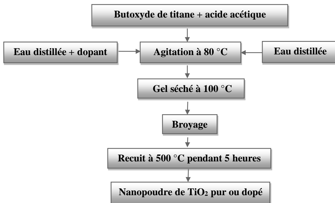
Fig.IV.3 Organigramme des étapes de préparation des nanopoudres de TiO 2 pur et dopé
