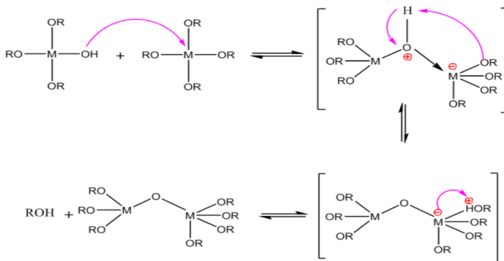
Fig.II.3 Mécanisme d'alcoylation des alcoxydes métalliques M(OR)_n [4]
