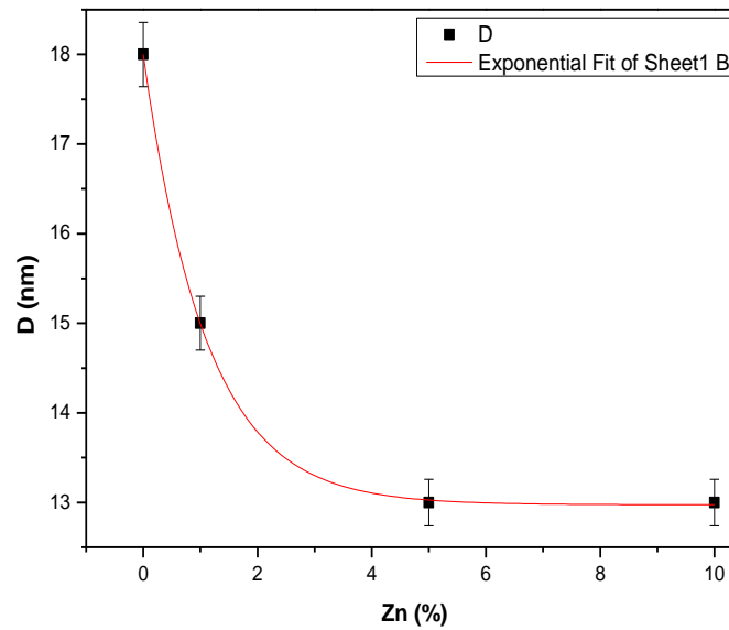
Fig.V.14 Evolution de la taille des grains de Zn-TiO 2 en fonction de la concentration en Zn
