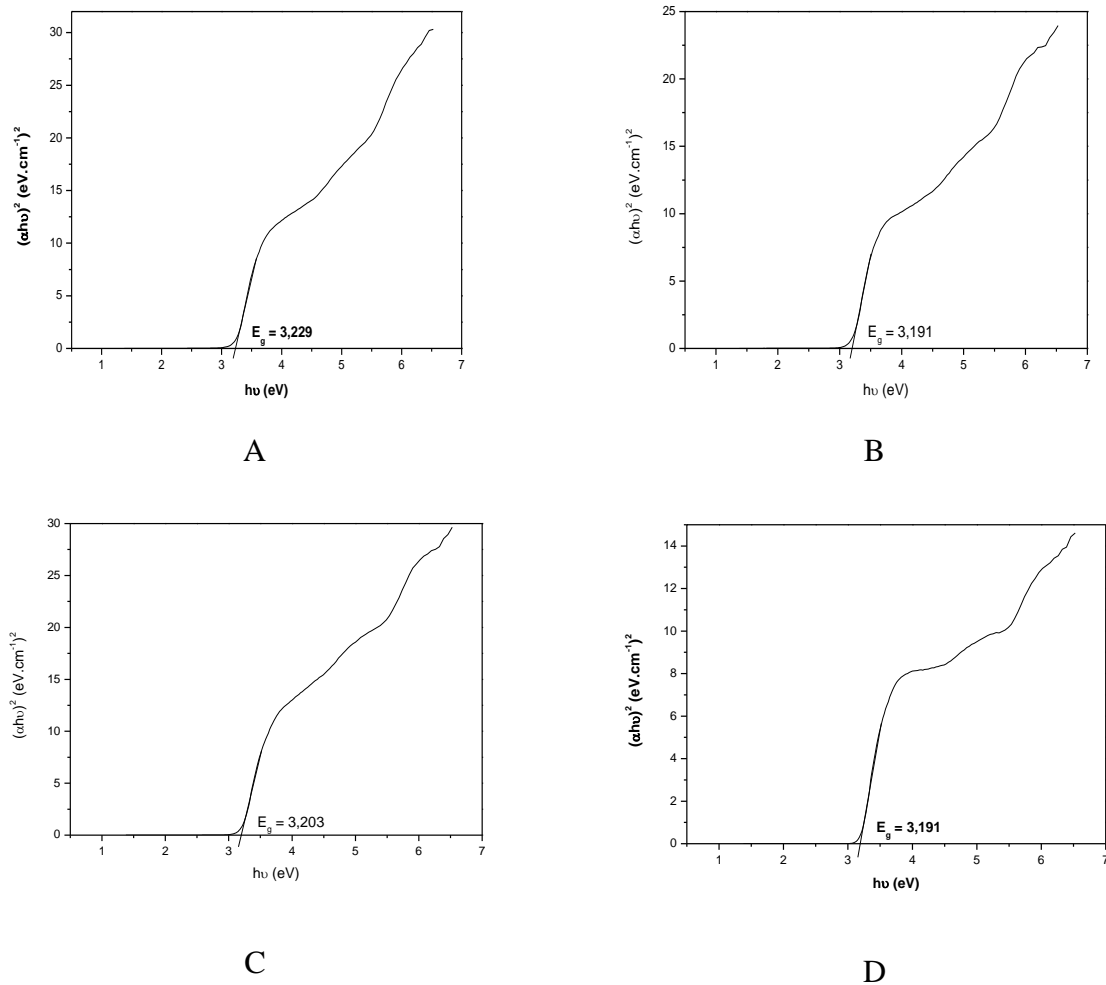
Fig.V.22 Détermination de l'énergie de la bande des nanoparticules de TiO 2 pur (A) et de TiO 2 dopé au Zn : 1% (B), 5% (C) et 10% (D)
