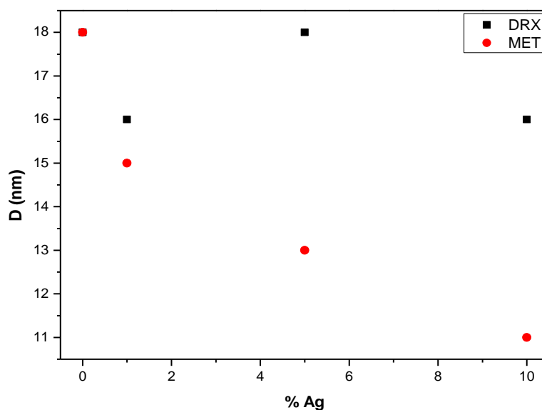
Fig.V.8 Evolution de la taille des grains en fonction de la concentration en Ag par DRX et par MET
