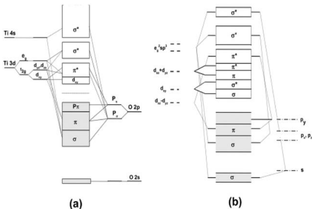
Fig.I.10 Orbitales moléculaires de TiO 2 (a) anatase (b) rutile [39, 40]
