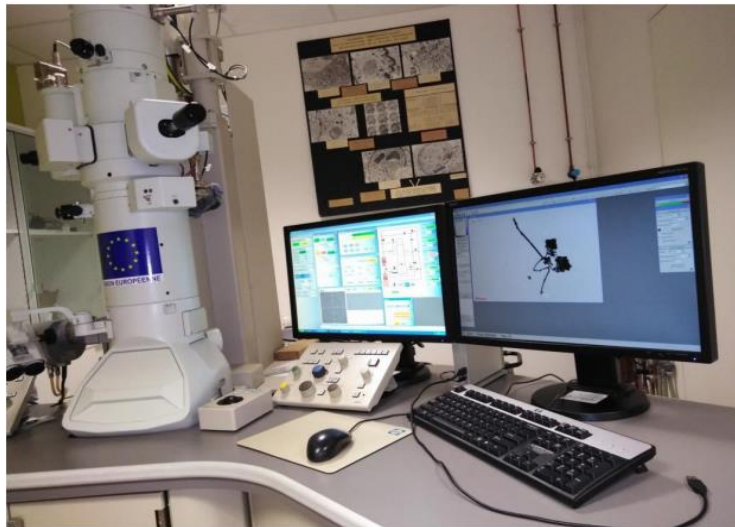
Fig.III.6 Photo du MET « JEOL JEM-1400 Electron Microscope »
