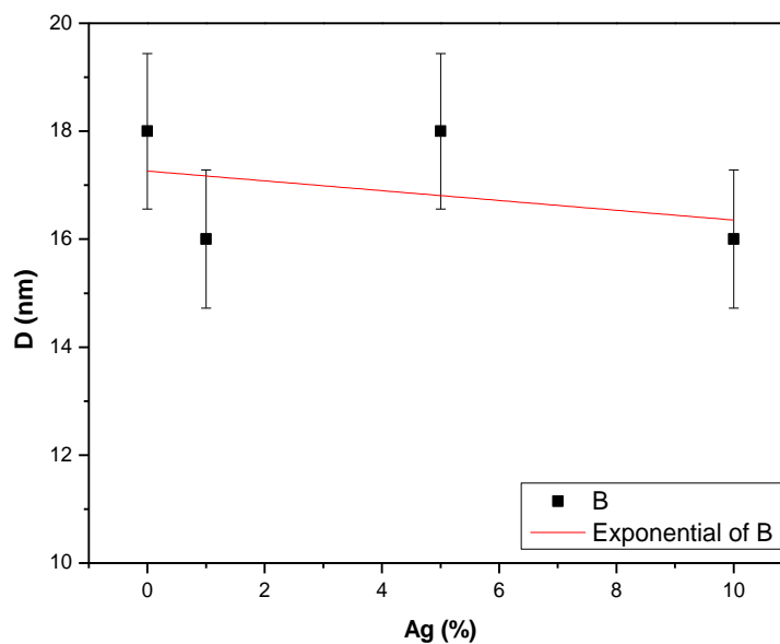
Fig.V.2 Evolution de la taille des grains de Ag-TiO 2 en fonction de la concentration en Ag
