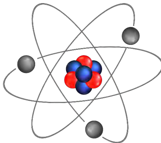
Figure 4.1 : Illustration d'un atome
