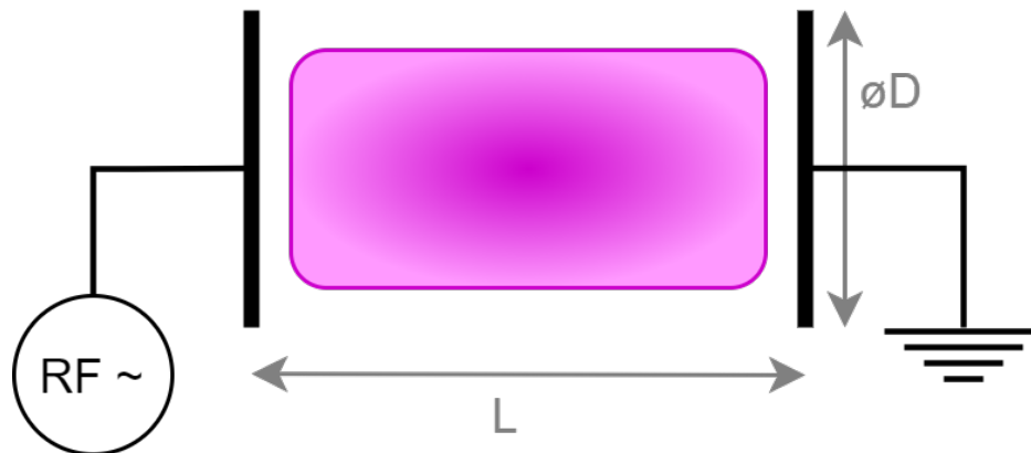
FIGURE 1.2 – Schéma d'une décharge RF capacitive
