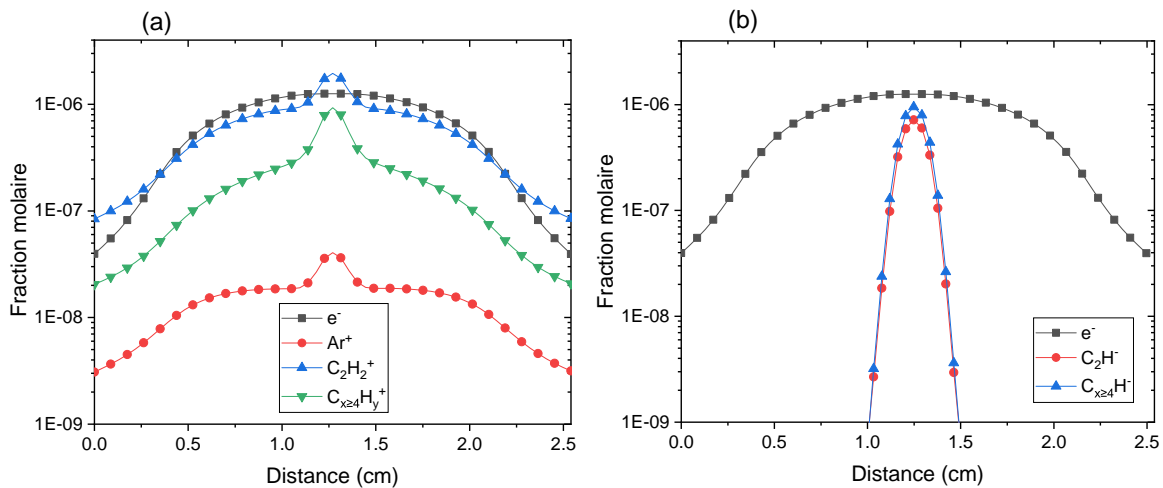
FIGURE 3.9 – Fractions molaires des électrons, Ar + , C 2 H 2 + et les cations de grande taille de type C 2n≥4 H y=2,6 + (a), e - , C 2 H - et les anions regroupés de plus grande taille (b)
