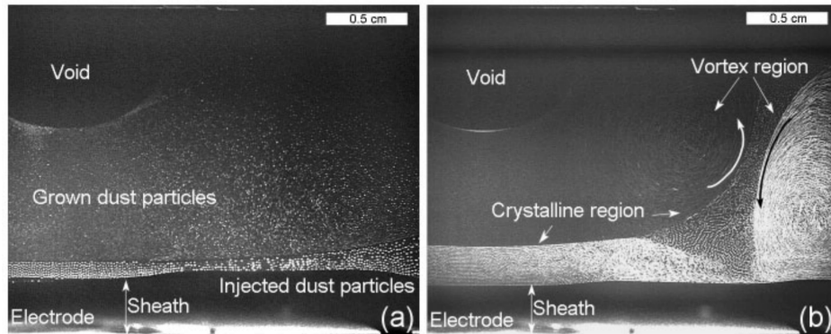
FIGURE 1.11 – Vooids dans un réacteur PKE-Nefedov [82]
