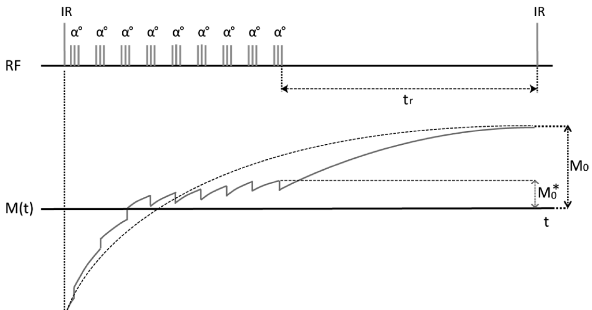
Figure 10 : Diagramme de la séquence de Look-Locker 55 . On remarque que le M_0^* , représentant le signal effectif est inférieur au M_0 théorique du fait de l'application multiple de pulses avec un angle \alpha .
