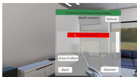
FIGURE 5.4 – Menu pour associer des objets à un besoin spécifique d'une chaîne d'interaction
