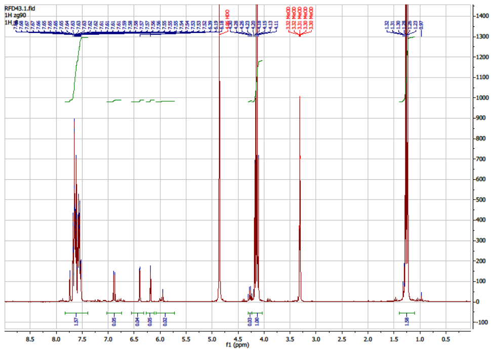
Figure 49- Spectre RMN 1 H (MeOD, 300MHz) de éthyloxyquercétine
