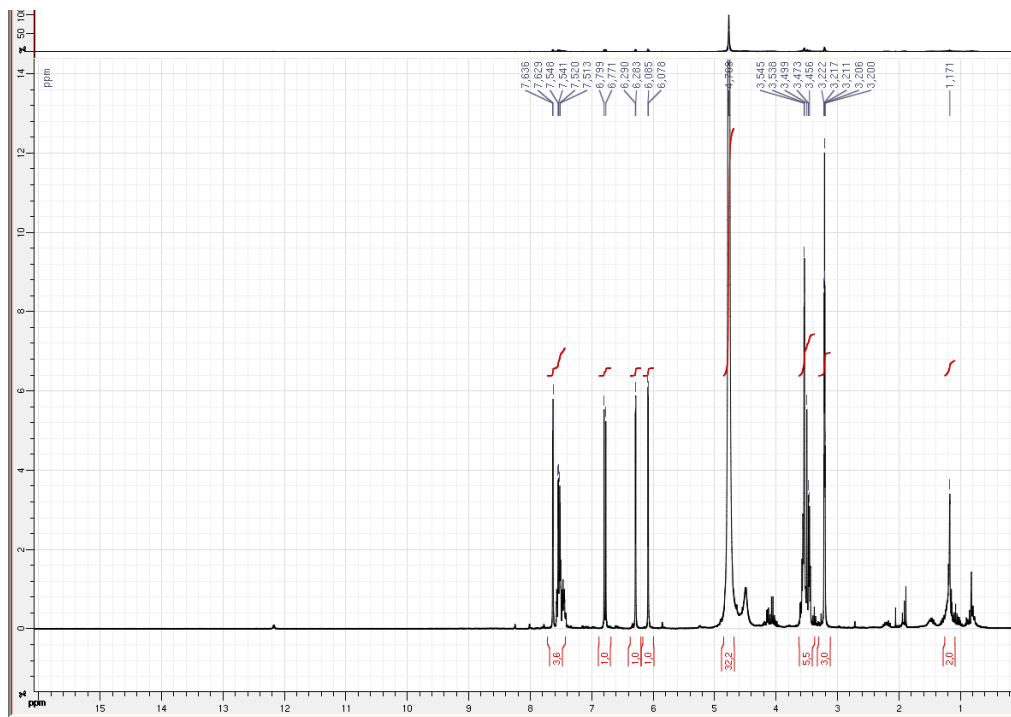
Figure 50- Spectre RMN ^1\text{H} (MeOD, 300MHz) de tétraéthylenglyoxyquercétine
