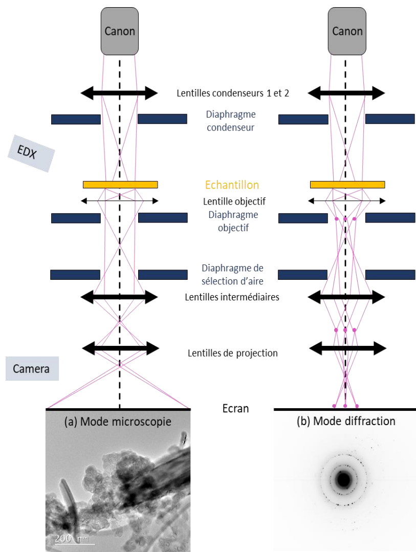
Figure 138 : Schéma de fonctionnement d'un microscope électronique à transmission avec (a) le mode de microscopie pour obtenir une image et en (b) de mode diffraction pour observer le cliché de diffraction pour un échantillon de \text{FeCO}_3 .
