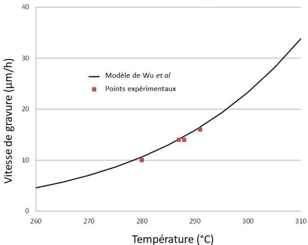
Figure 44 : Vitesse de gravure ( \mu\text{m}/\text{h} ) d'un wafer en saphir en fonction de la température ( ^{\circ}\text{C} ) par une solution acide \text{H}_2\text{SO}_4 / \text{H}_3\text{PO}_4 .
