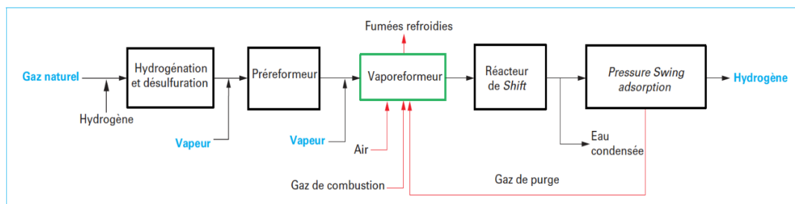
Figure 7 : Vaporeformage pour la production de l'hydrogène [20].
