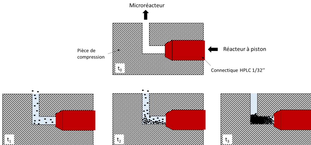
Figure 124 : Schéma du phénomène de bouchage ayant lieu lors du passage des particules de fer au sein de la pièce de compression en fonction du temps : t_0 pièce de compression avant le début de l'injection avec visualisation du coude, t_1 début de l'injection avec passage de particules de fer dans le coude, t_2 dépôt de particule et t_3 bouchage de la pièce.
