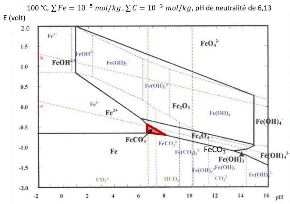
Figure 19 : Diagramme potentiel-pH du fer dans un milieu aqueux concentré en carbonate à 10^{-3} \text{ mol.kg}^{-1} à 100 °C [74].
