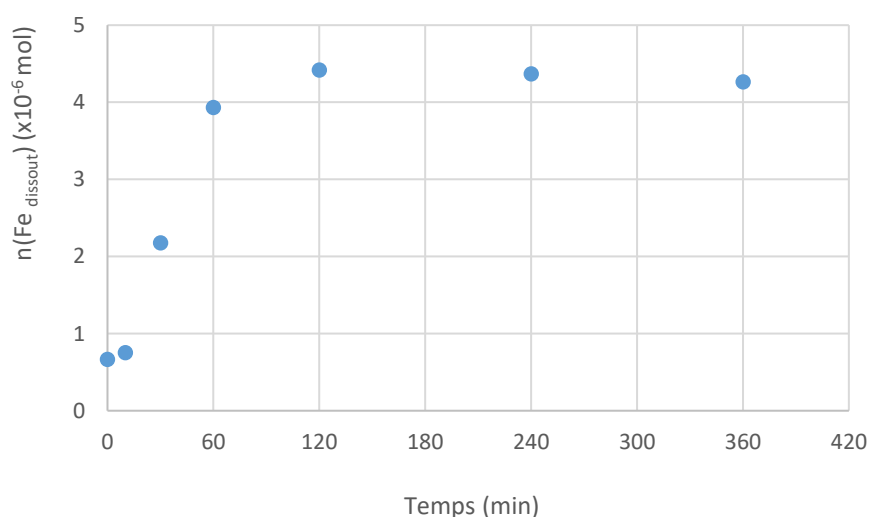
Figure 79 : Quantité de fer dissout dans la phase liquide en fonction du temps (min)
