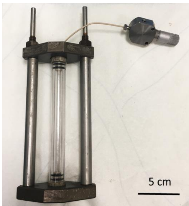
Figure 59 : Image du réacteur millifluidique en saphir fermé.
