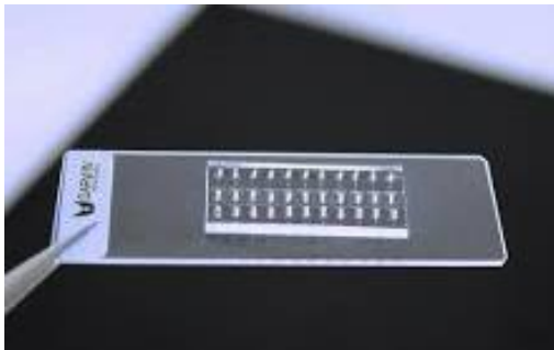
Figure 29 : Microréacteur en PDMS (source darwin-microfluidics.com).
