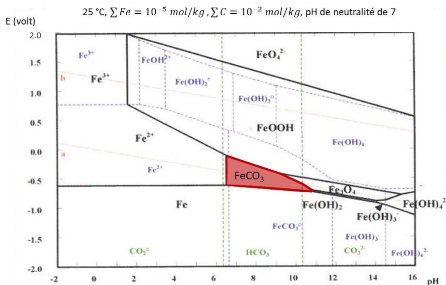
Figure 18 : Diagrammes potentiel-pH du fer à 25 °C dans un milieu aqueux concentré en carbonate avec A) 0 \text{ mol.kg}^{-1} , B) 10^{-4} \text{ mol.kg}^{-1} , C) 10^{-3} \text{ mol.kg}^{-1} et D) 10^{-2} \text{ mol.kg}^{-1} . En rouge est matérialisé le domaine de stabilité de \text{FeCO}_3 [74].
