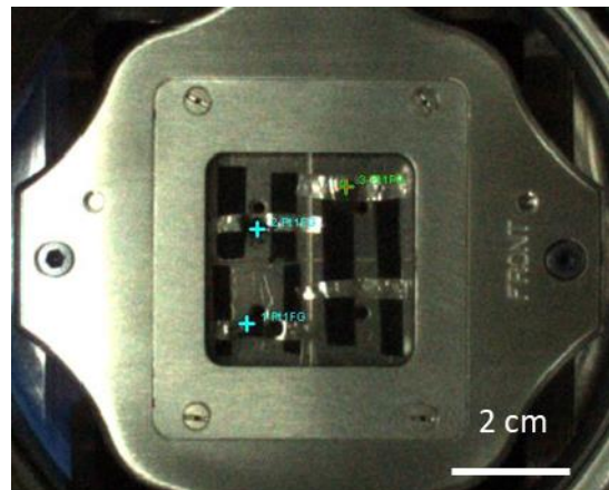
Figure 63 :Vue du dessus du module K-ALPHA avec emplacements spécifiques (croix bleues et vertes) pour les échantillons.
