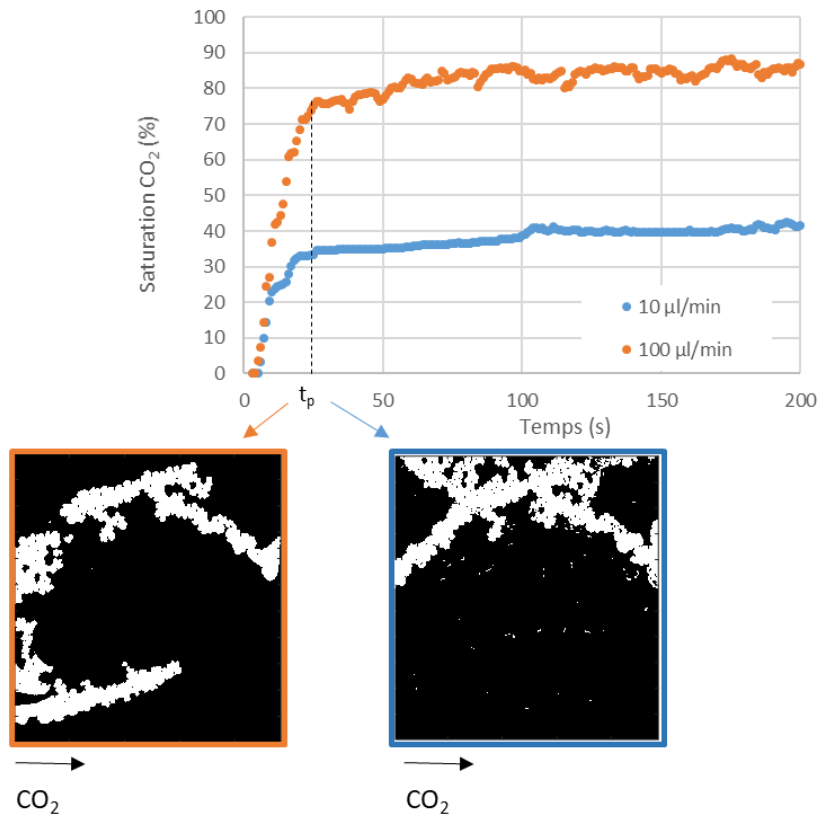
Figure 111 : Saturation en \text{CO}_2 en fonction du temps et de N_{eq} pour un débit d'invasion de 10 \mu\text{l}/\text{min} (courbe bleue) et 100 \mu\text{l}/\text{min} (courbe orange) pour un microréacteur hétérogène.
