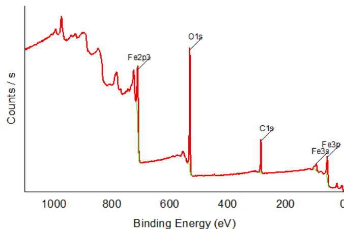
Figure 66 : Spectre général obtenu par analyse XPS de la poudre de fer initiale.
