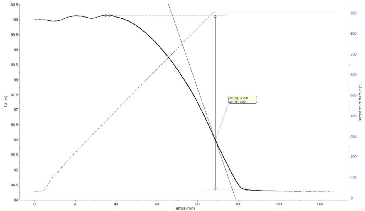
Figure 139 : Analyse thermogravimétrique d'une poudre sous atmosphère Ar/H 2 : représentation du pourcentage en masse et de la température du four en fonction de la température.
