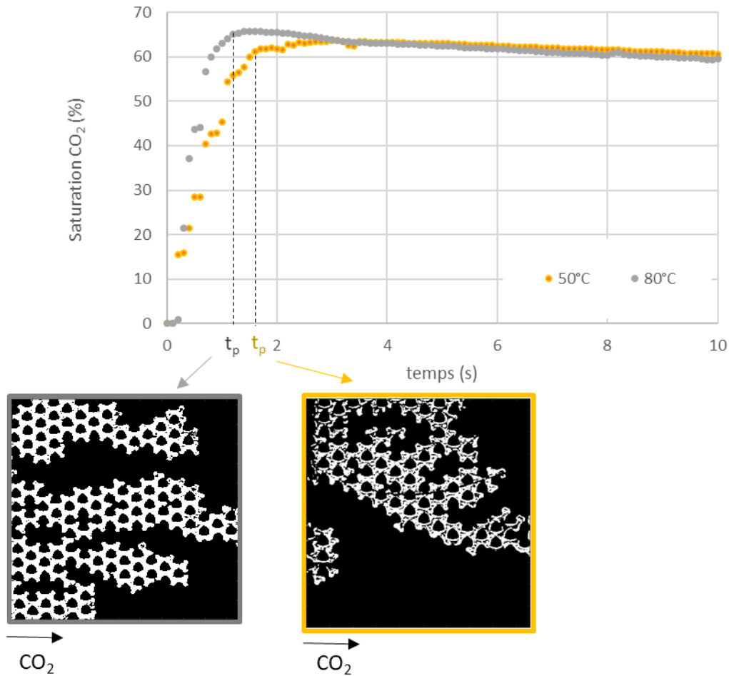
Figure 113 : Saturation en CO 2 en fonction du temps pour une température de 50 °C (jaune) et 80 °C (gris) à une pression de 80 bar et un débit de 100 µl/min pour un microréacteur homogène.
