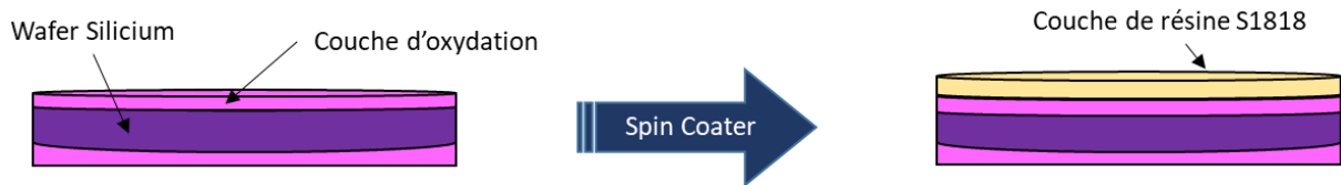
Figure 35 : Schéma explicatif de l'étape 1 concernant le dépôt d'une couche de résine sur un wafer oxydé en silicium.
