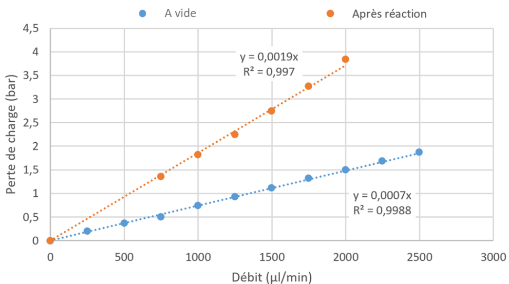
Figure 127 : Perte de charge du milieu poreux homogène avant et après la réaction des particules de fer
