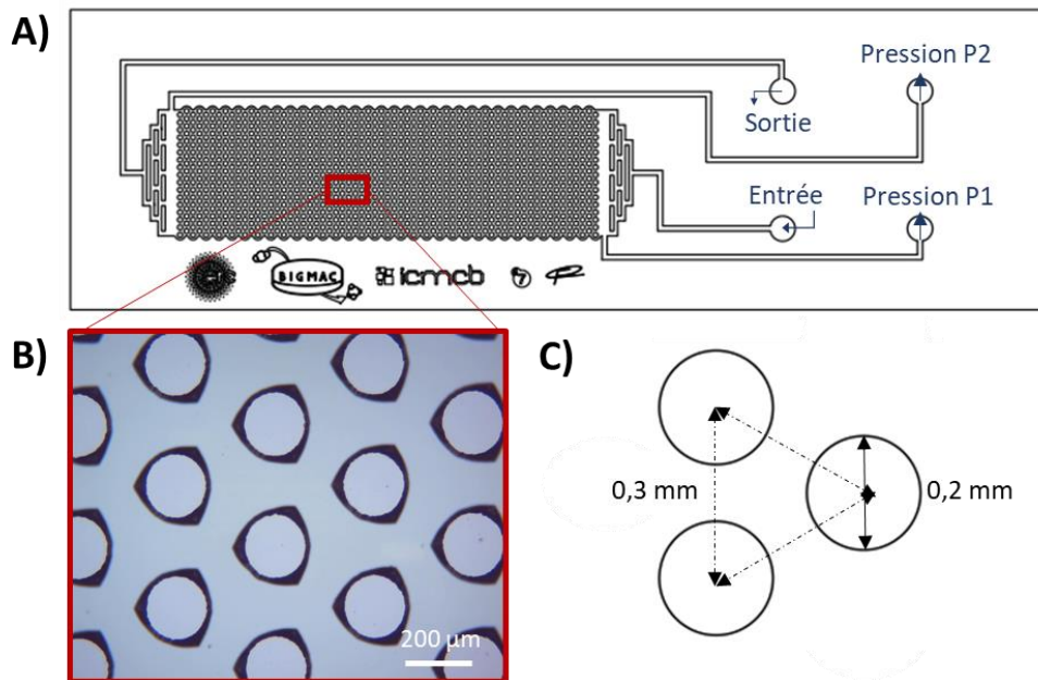
Figure 95 : Microréacteur en saphir de type poreux homogène avec A) une vue plan du « design » du microréacteur, B) un cliché de microscopie optique de l'intérieur du milieu poreux et C) les caractéristiques géométriques des plots.
