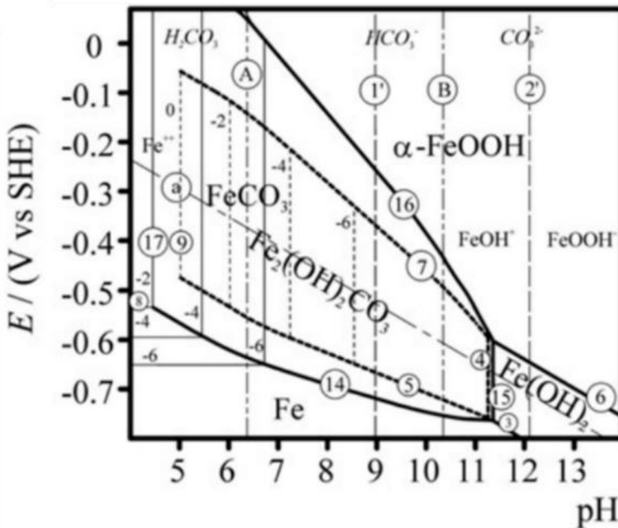
Figure 21 : Diagramme potentiel-pH du fer à 25 °C dans un milieu carbonaté avec le domaine de prédominance de la chukanovite ( \text{Fe}_2(\text{OH})_2\text{CO}_3 ) représenté en ligne pointillée [72].
