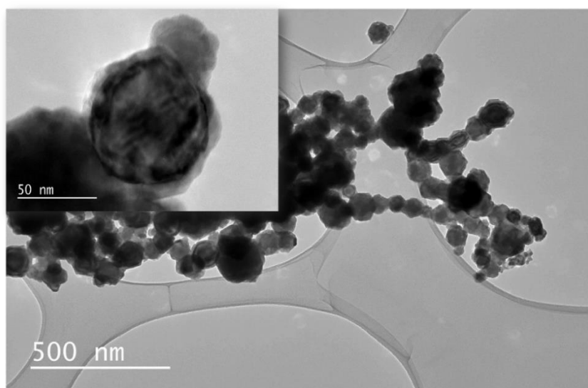
Figure 71 : Images réalisées par microscopie électronique à transmission sur la poudre de fer initiale.
