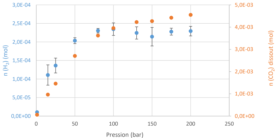
Figure 80 : Evolution de la production d'H 2 (en mole) en fonction de la pression du système CO 2 /H 2 O (en bar) dans un environnement maintenu à 50 °C pendant 1 h.
