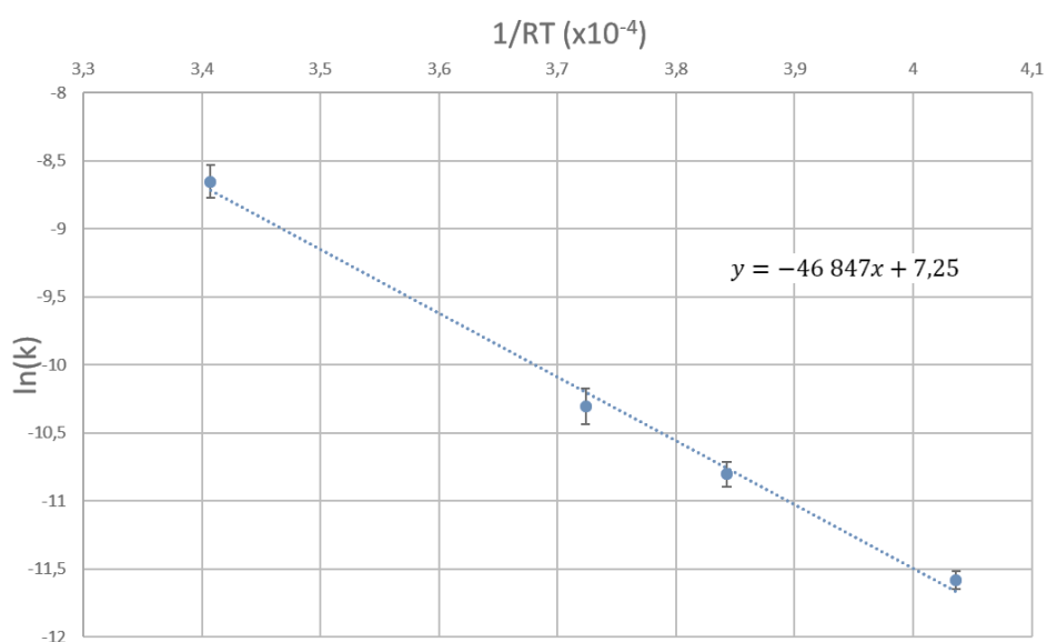
Figure 87 : Représentation du logarithme népérien de la constante de vitesse en fonction de l'inverse de RT avec R égale à 8,314 \text{ J.mol}^{-1}\text{K}^{-1} et T en kelvin.
