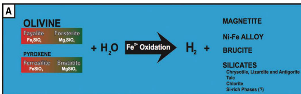
Figure 16 : Réaction de serpentinisation avec production d'hydrogène à partir d'olivine et de pyroxène [51].
