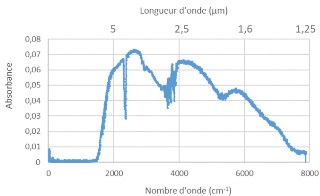
Figure 55 : Spectre d'absorption du microréacteur en saphir.
