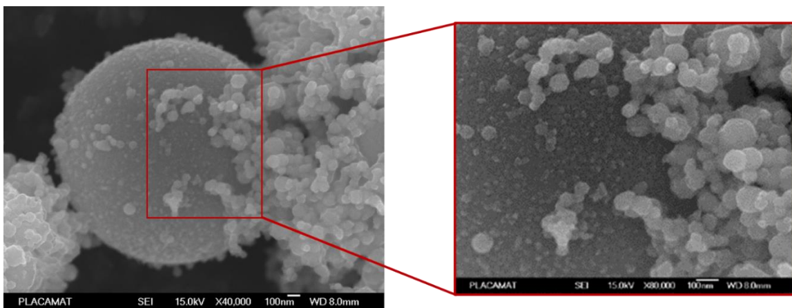
Figure 70 : Images réalisées par microscopie électronique à balayage sur la poudre de fer initiale.
