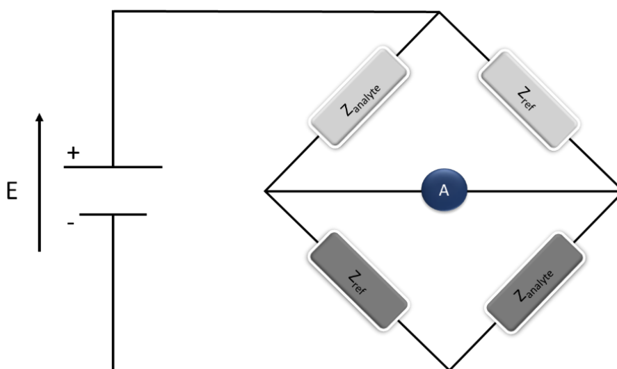
Figure 131 : Schéma du pont de Wheastone avec A l'ampèremètre qui mesure le courant électrique, Z_{ref} l'impédance du filament de référence et Z_{analyte} l'impédance du filament parcouru par l'analyte..
