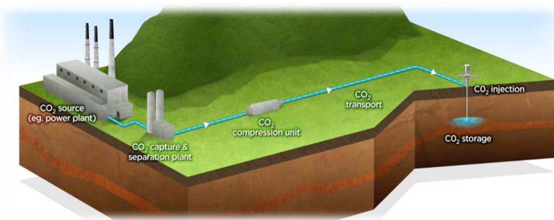
Figure 5 : Schéma de principe du CGS contenant cinq grandes étapes à partir de la capture du CO 2 jusqu'au lieu de stockage [13].
