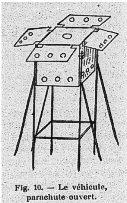
Fig. 10. — Le véhicule, parachute ouvert. Illustration 16: Le système de ralentissage atmosphérique imaginé par Coissac
