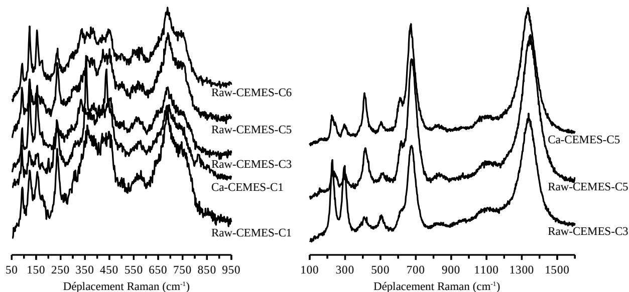
Figure 86 : Spectres Ramans de phase \epsilon - \text{Fe}_2\text{O}_3 (gauche) et d'hématite (droite) enregistrés sur les échantillons soumis aux cycles de la série CEMES
