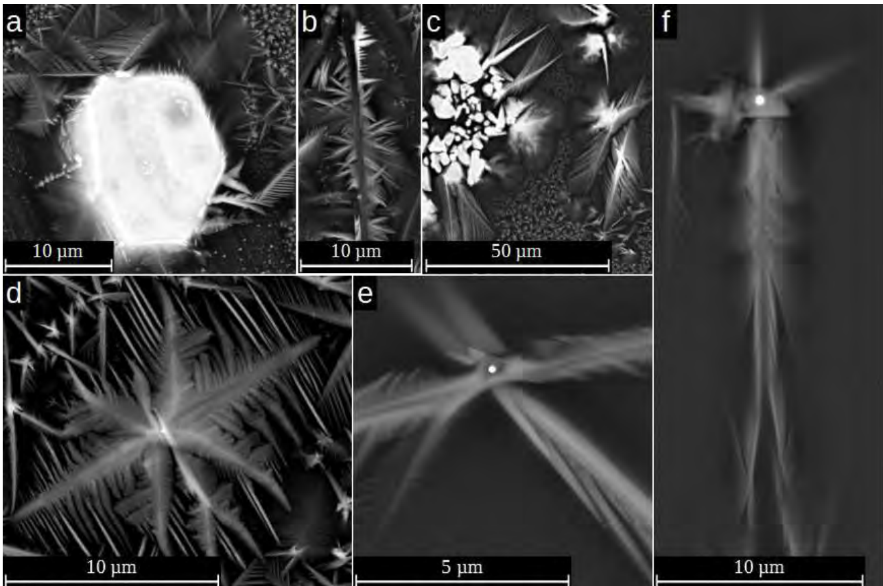
Figure 74 : Images SEM (BSE, 18 kV, grossissements x1000 à x10000) de grosse dendrites poussant sur un cristal de zircon sur Fuj1-CP-C2 (a), une aiguille de mullite sur Jish1-CP-C3 (b), des cristaux géométriques riches en fer sur Jish1-CP-C3 (c) et des nanoparticules sur Fuj1-CP-C2 (d) et Fuj2-CP-C2 (e et f)
