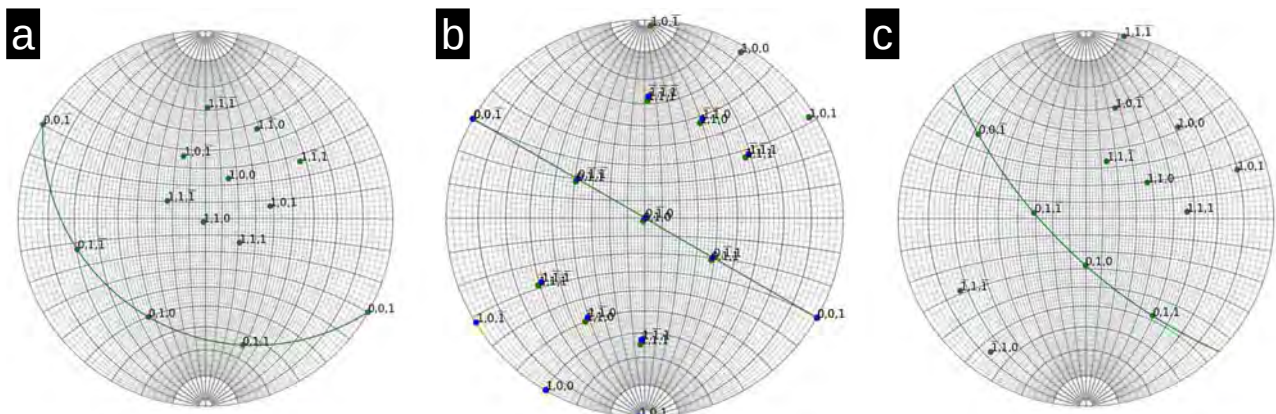
Figure 40 : Figures de pôle associées à l'orientation de la phase \varepsilon\text{-Fe}_2\text{O}_3 dans les dendrites de LHP-01 (a), LHP-02 (b) et BG-01 (c)
