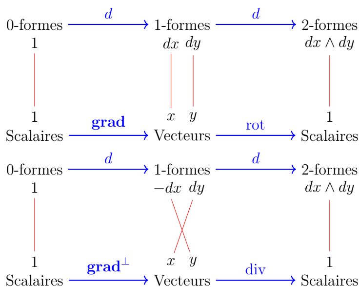
Figure 1.3: Deux identifications possibles entre les vecteurs et les formes en dimension 2.
