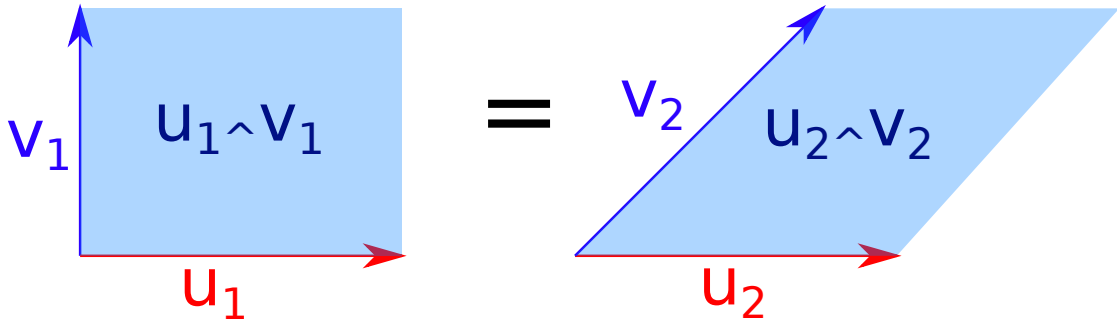
Figure 1.1: Deux paires de vecteurs ayant un même produit extérieur.
