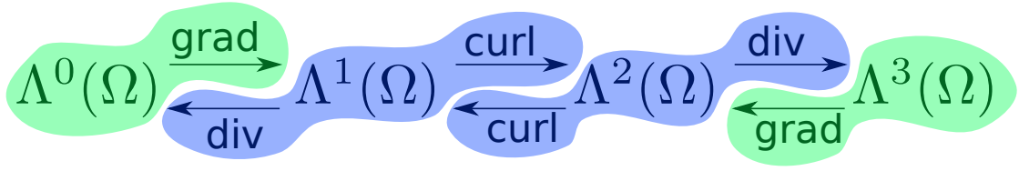
Figure 1.4: Répartition des problèmes de Hodge-Dirac sur le complexe de De Rham.
