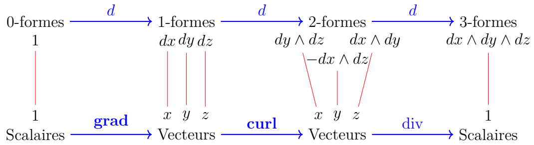
Figure 1.2: Identification entre les vecteurs et les formes en dimension 3.
