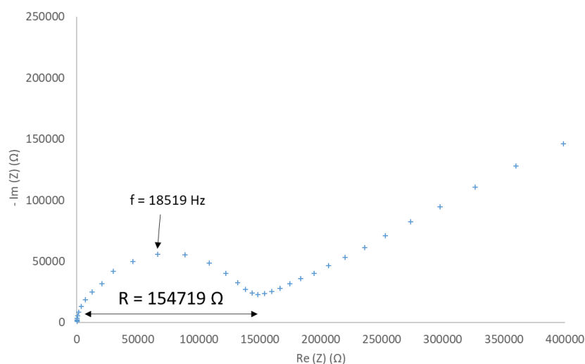
Figure 95. Diagramme de Nyquist obtenu avec un séparateur de résine époxy et l'électrolyte liquide OMIMTFSI, 1M LiTFSI. La résistance R dans ce séparateur est très supérieure à la résistance bulk ( \sim 300 \text{ } \Omega ). La conductivité dans la résine époxy peut donc être négligée.
