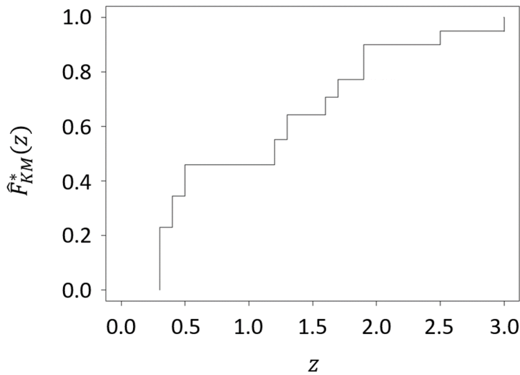
FIGURE 3.4 – Exemple d’application de l’estimateur de Kaplan-Meier pour l’estimation d’une fonction de répartition empirique.
