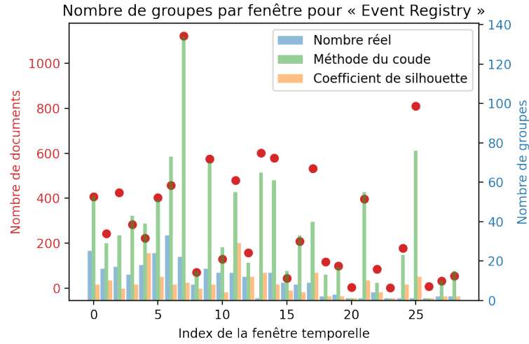
FIGURE 4.4 – Nombre de clusters par fenêtre temporelle découvert par la méthode du « coude » ou du coefficient de silhouette par rapport à la réalité.
