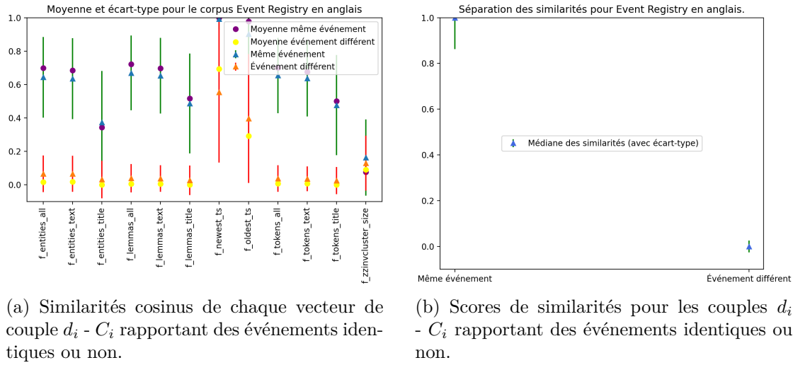
FIGURE 4.2 – Scores de similarités durant le processus d'entraînement de l'algorithme, avant et après le calcul de l'équation 4.5 et application de la fonction sigmoïde
