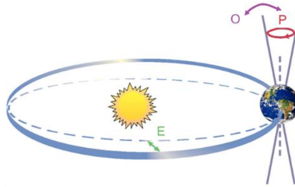
Orbite circulaire sans inclinaison
