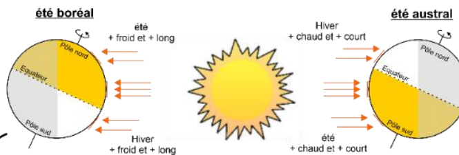
Orbite ecliptique (E) + Inclinaison (O) + Précession (P)
