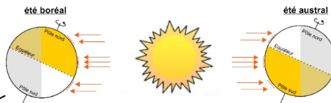
Orbite ecliptique (E) + Inclinaison (O)
