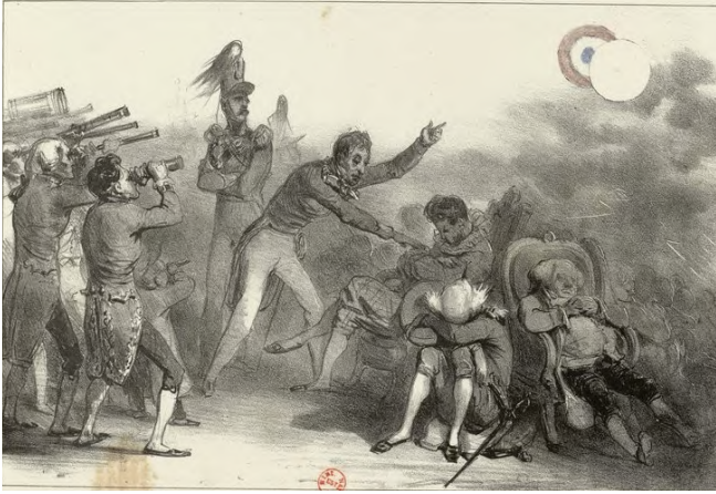
Fig. 36 : L'éclipse de 1832
