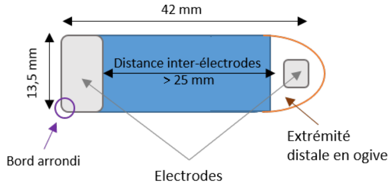
FIGURE 3.9 – Schéma du dispositif intra-gastrique : géométrie et dimensions.
