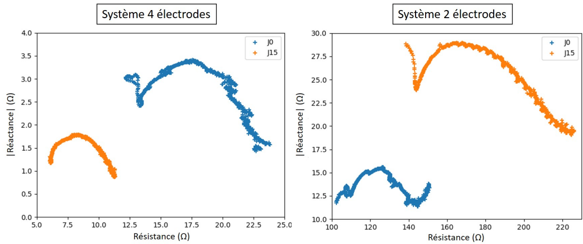
FIGURE 4.16 – Représentation de l'évolution de la courbe résistance/réactance à différentes fréquences en post-implantation immédiate (courbes bleues) et 15 jours après implantation (courbes oranges). A gauche : mesures de l'impédance gastrique avec 4 électrodes. A droite : mesures de l'impédance gastrique avec 2 électrodes.
