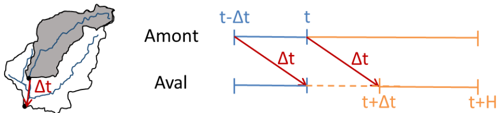
Figure 7-3 : Représentation schématique de l'adaptation de la prévision en contexte semi-distribué. Les sections bleues représentent les périodes où le débit est observé et les sections oranges où le débit est prévu. La zone en pointillée correspond à la période de temps où le débit prévu à l'aval est influencé par le débit déjà observé à l'amont. Cette zone est de longueur \Delta t , correspondant au temps de propagation du bassin amont vers l'aval.
