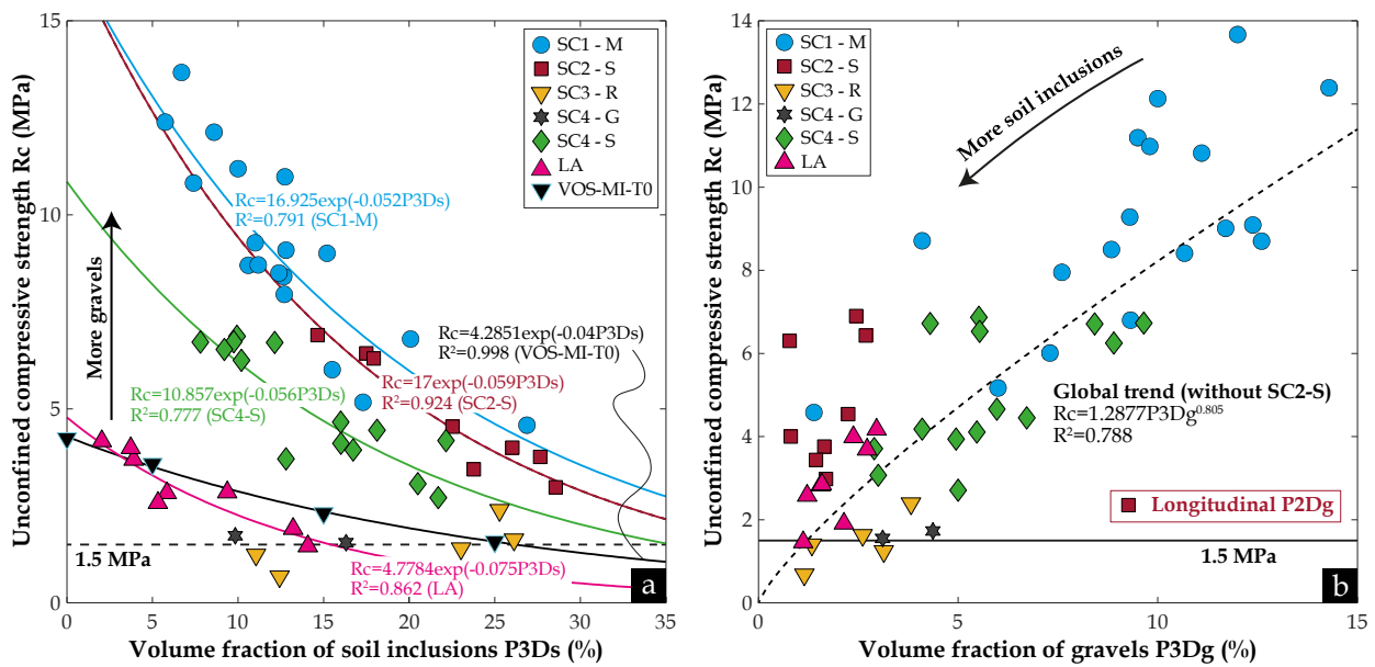
Fig. 184. Variation de la résistance à la compression simple R_c en fonction de : (a) Fraction volumique réelle d'inclusions de sol P_{3Ds} ; (b) Fraction volumique réelle de graviers P_{3Dg} [85 données + 4 données de VOS-MI-T0]
