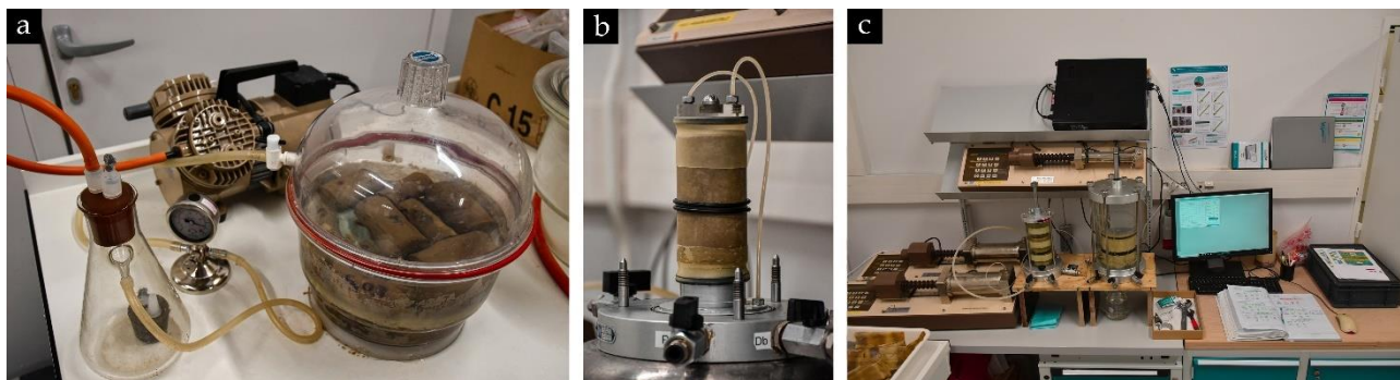
Fig. 66. (a) Saturation des éprouvettes de DSM sous vide ; (b) Montage d'une épreuve dans une membrane étanche ; (c) Dispositif de mesure de la perméabilité à l'eau dans une cellule triaxiale
