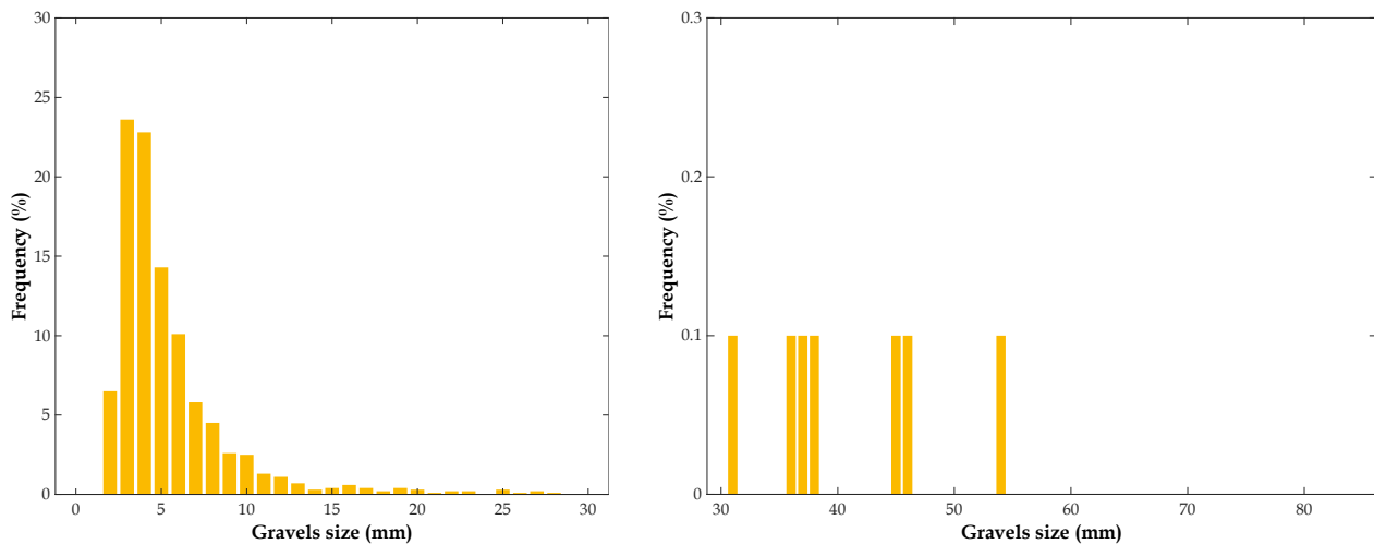
Fig. 330. Distribution de taille de graviers en 3D des 4 éprouvettes de SC4-S : (gauche) < 30 mm ; (droite) > 30 mm
