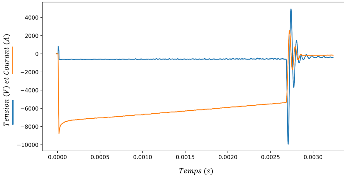
FIGURE 4.12 – Exemple d’une onde de courant et de tension expérimentale
