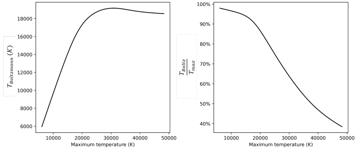
FIGURE 2.20 – (Gauche) : Température résultant de la mesure simulée par la méthode du diagramme de Boltzmann en fonction de la température maximale du profil gaussien correspondant. (Droite) : Pourcentage du maximum du profil que représente la mesure simulée en fonction de la température maximale du profil
