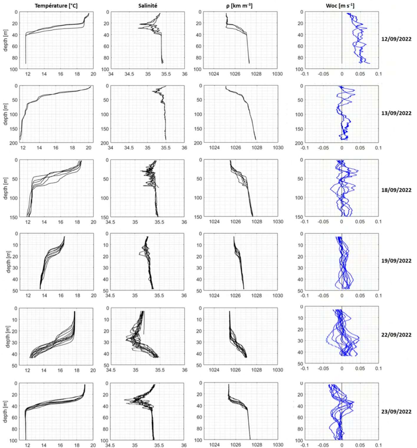
FIGURE 5.9. – Ensemble des profils de mesures effectués par le VVP durant la campagne PROTEVS-Gascogne (2022).
