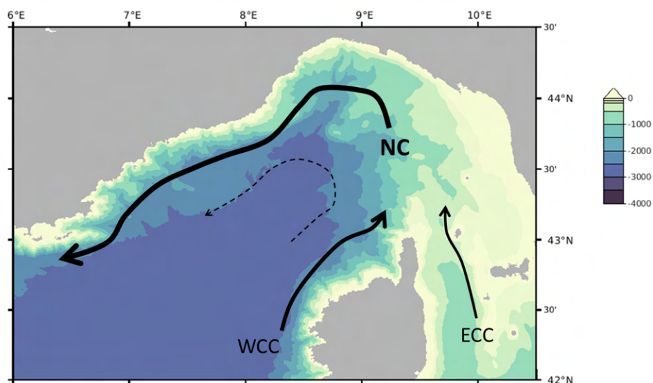
FIGURE 2.13. – Circulation générale des eaux de surface et bathymétrie en mer Ligurie, adaptée de MILLOT et al. 2005. NC : courant Nord , WCC : courant Ouest-Corse , ECC : courant Est-Corse . La ligne pointillée représente la recirculation cyclonique de surface induite par le WCC et le NC.
